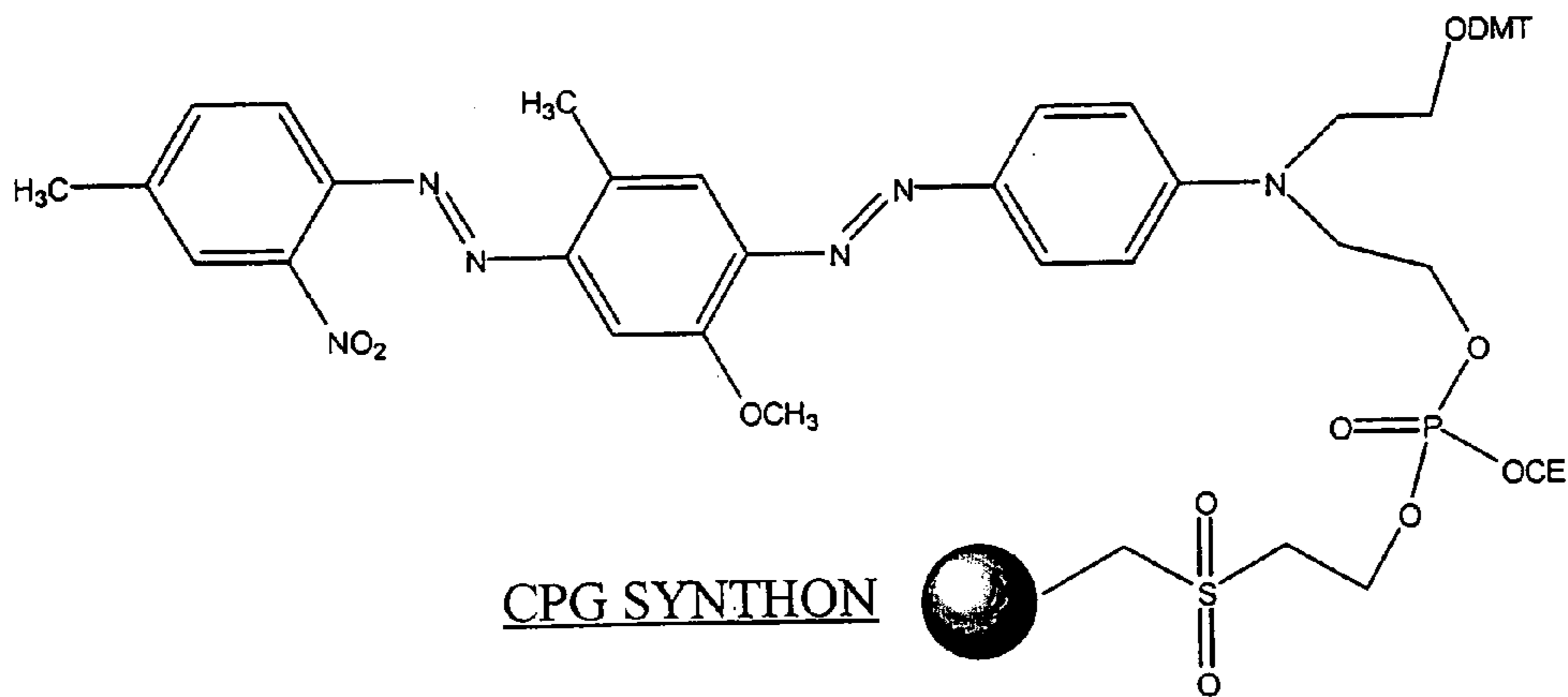
AMIDITE
