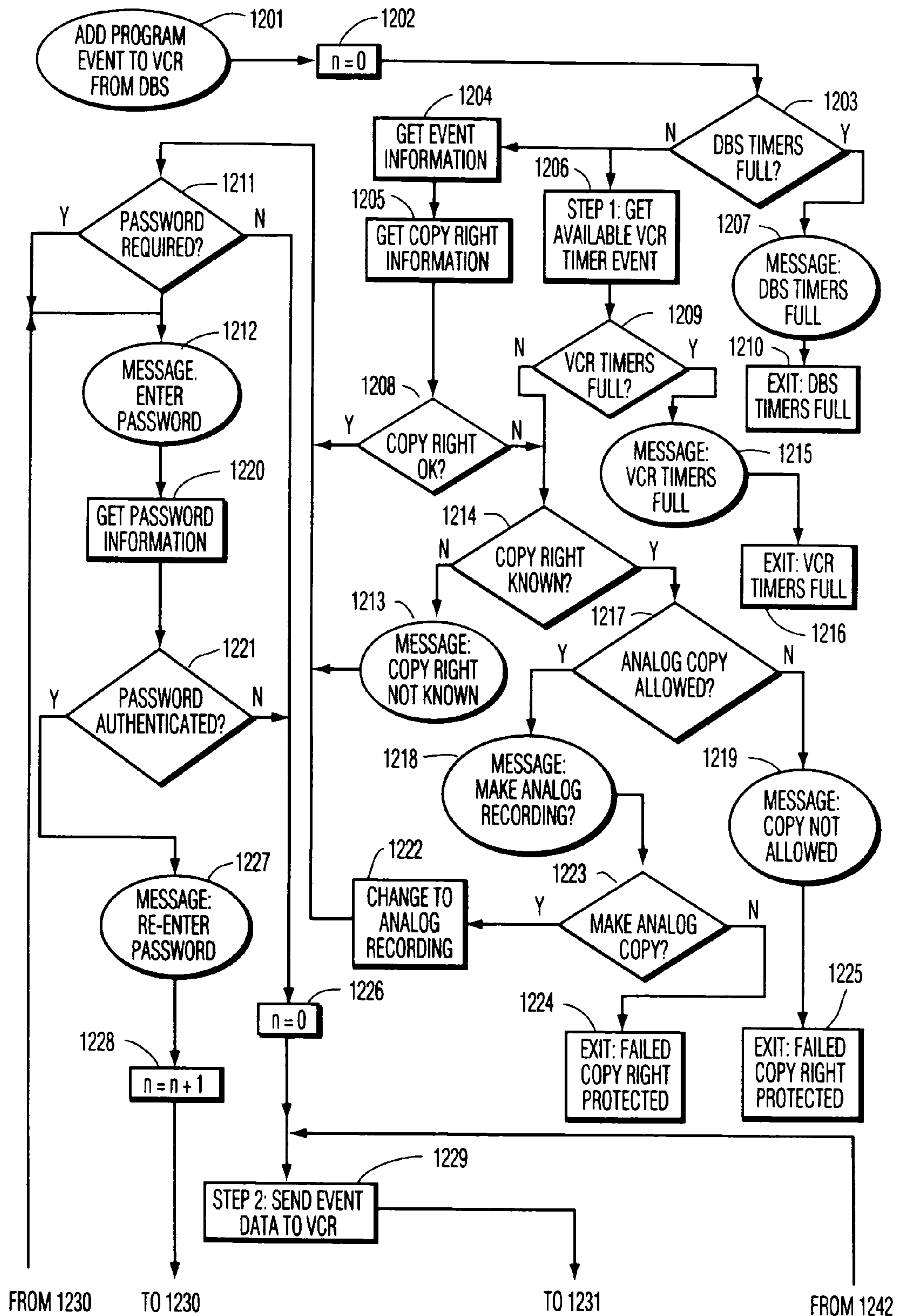
FIG. 12A
