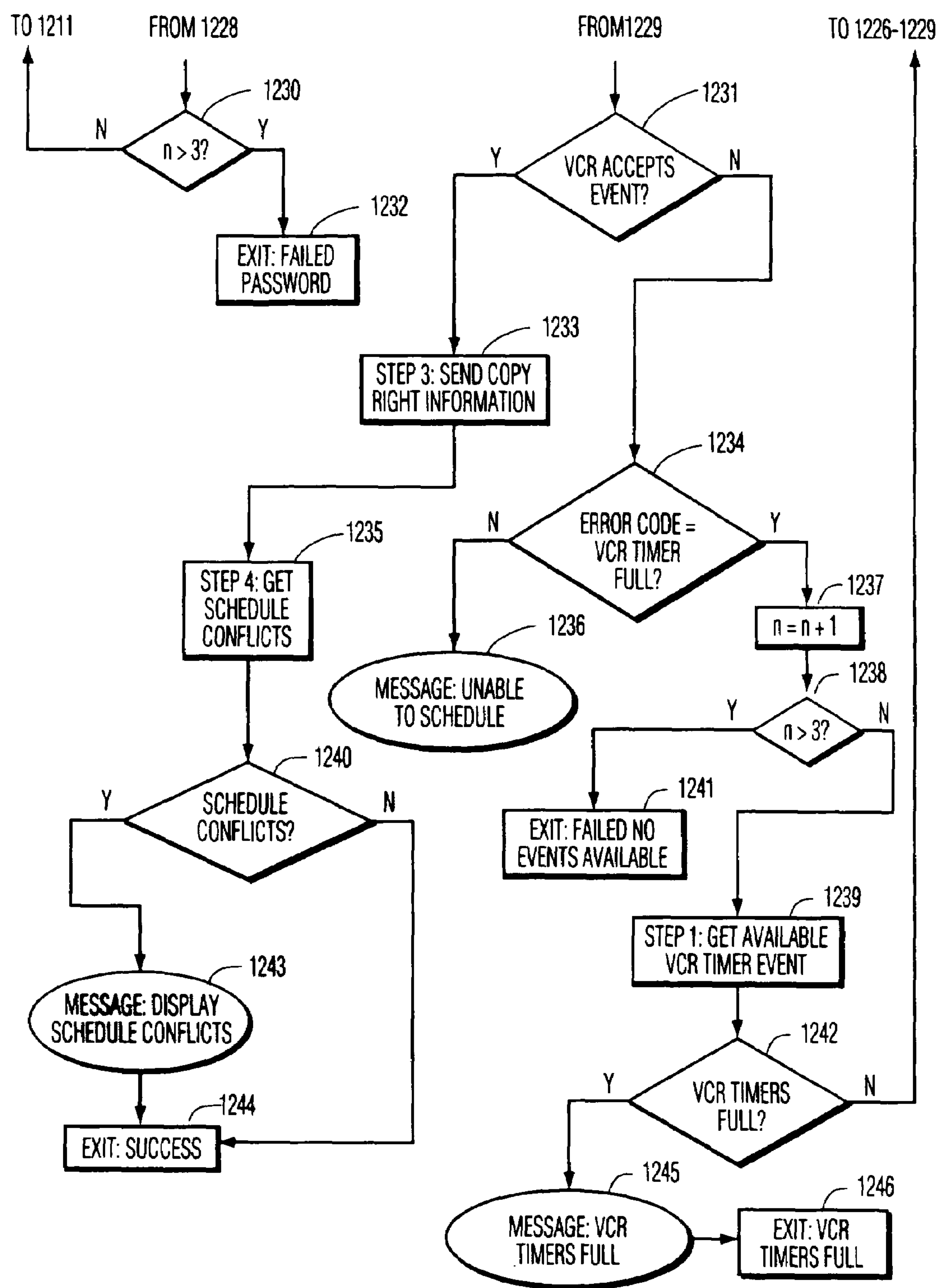
FIG. 12B
