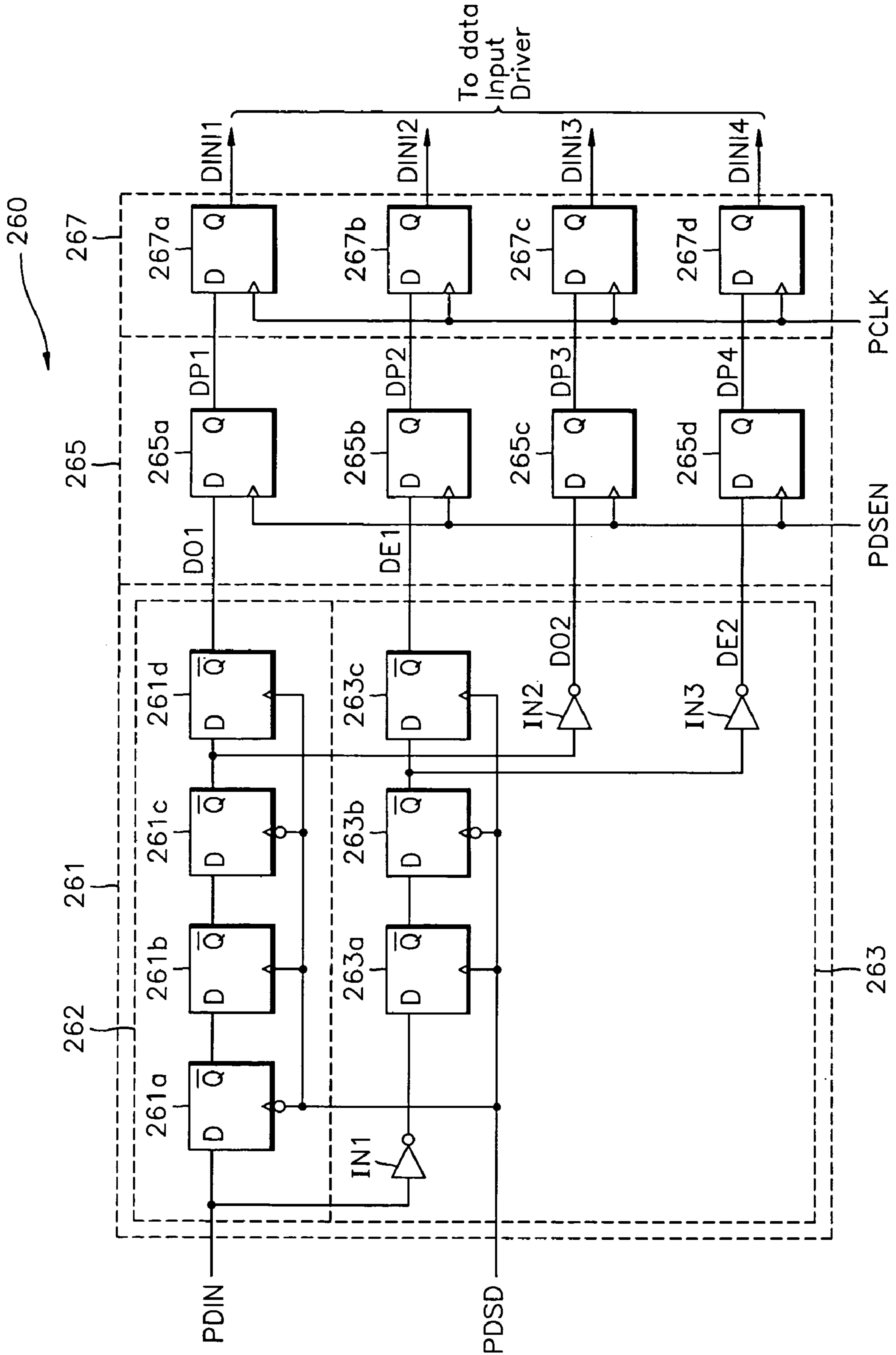
FIG. 9A
