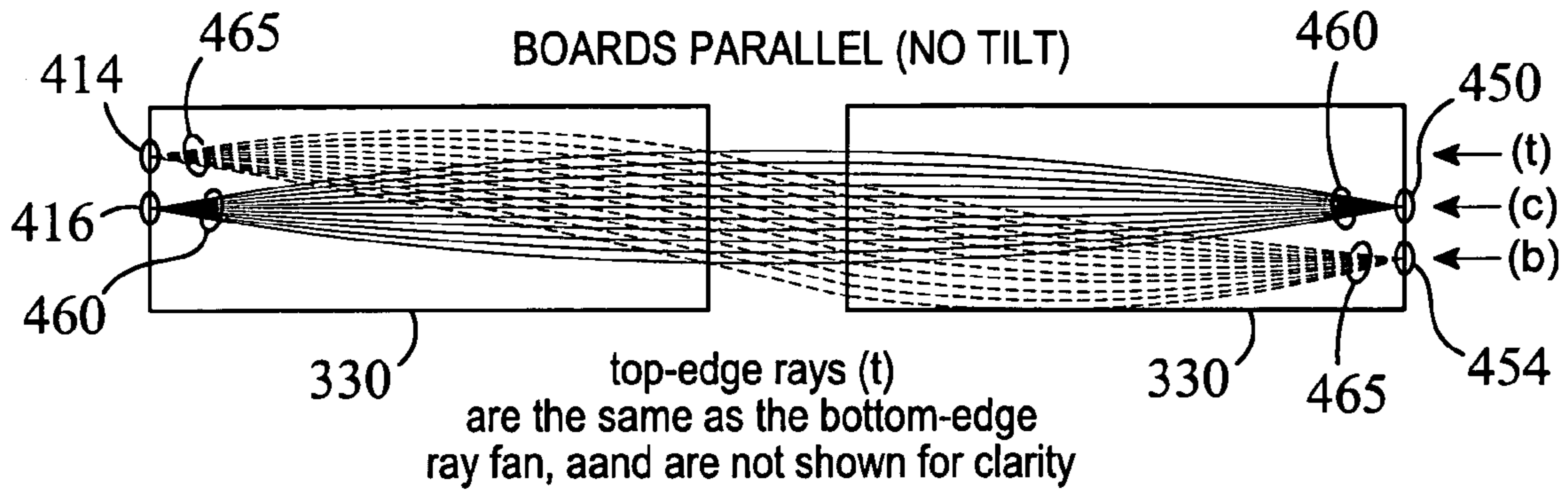
FIG. 16A
