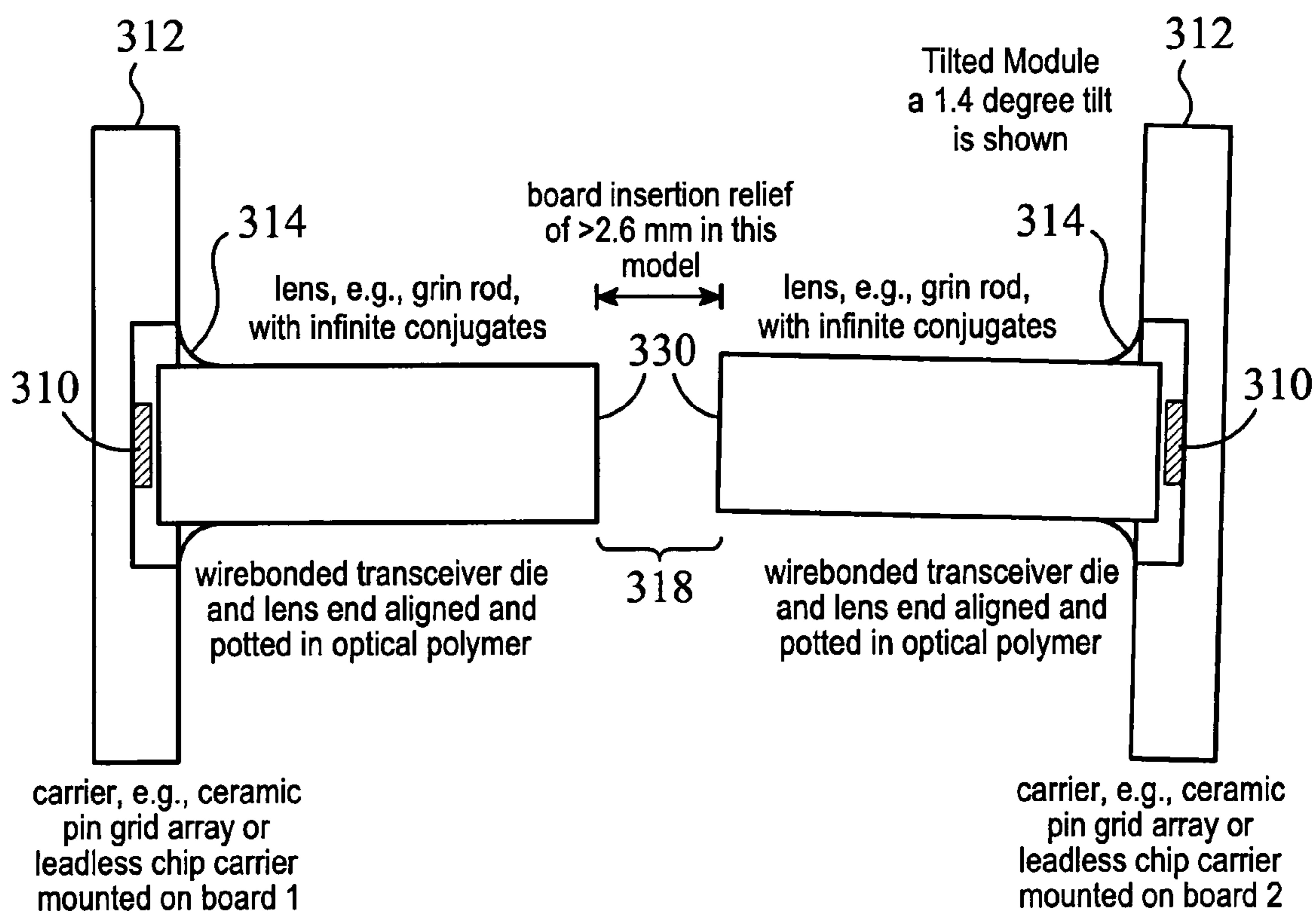
FIG. 17
