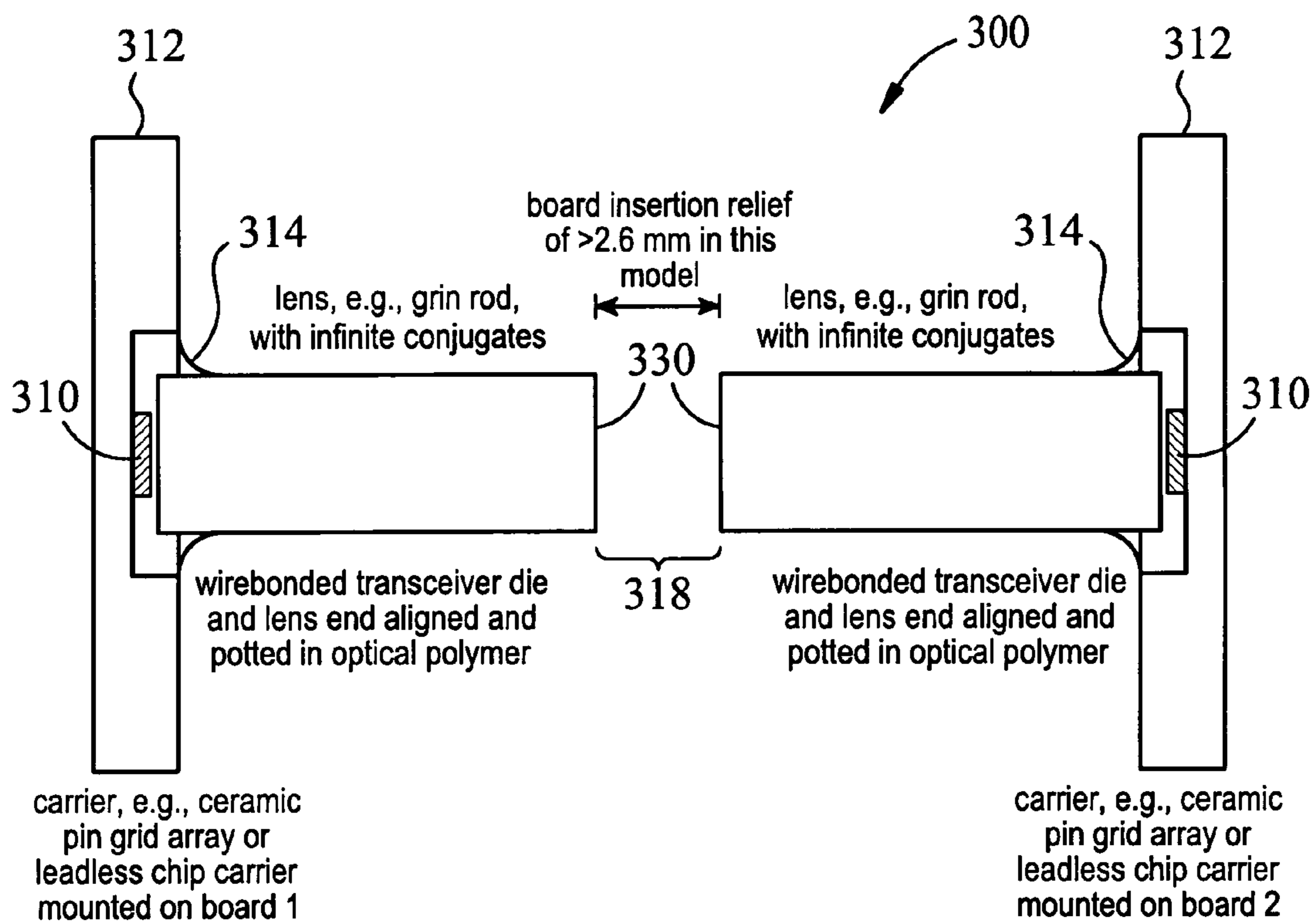
FIG. 14
