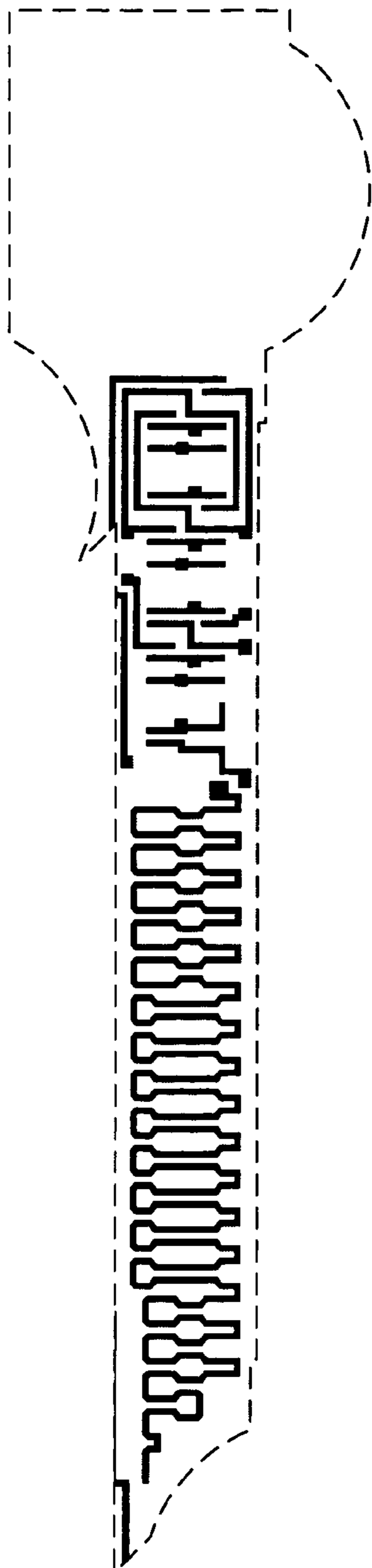
Poly mask
