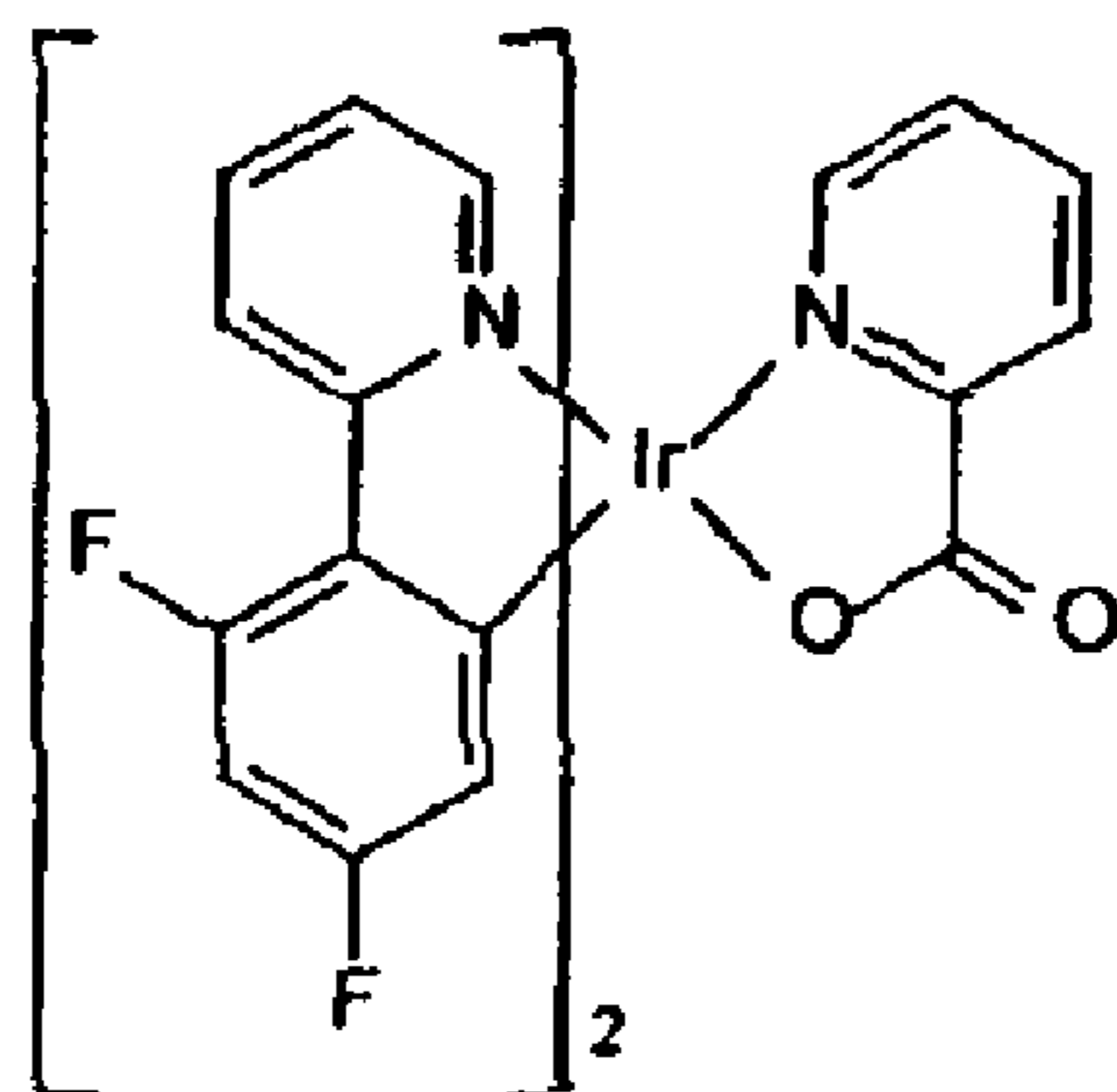
Ir(pic)
