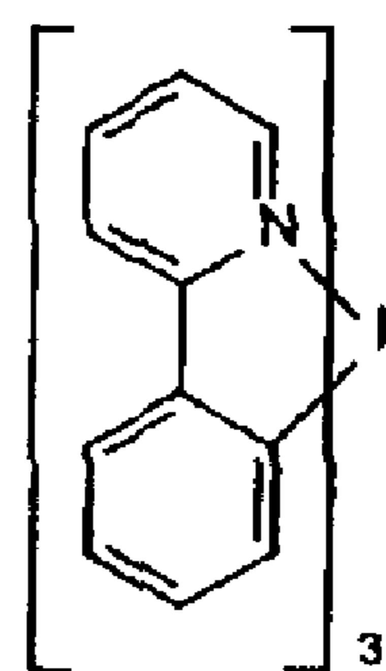
Ir(ppy) 3
