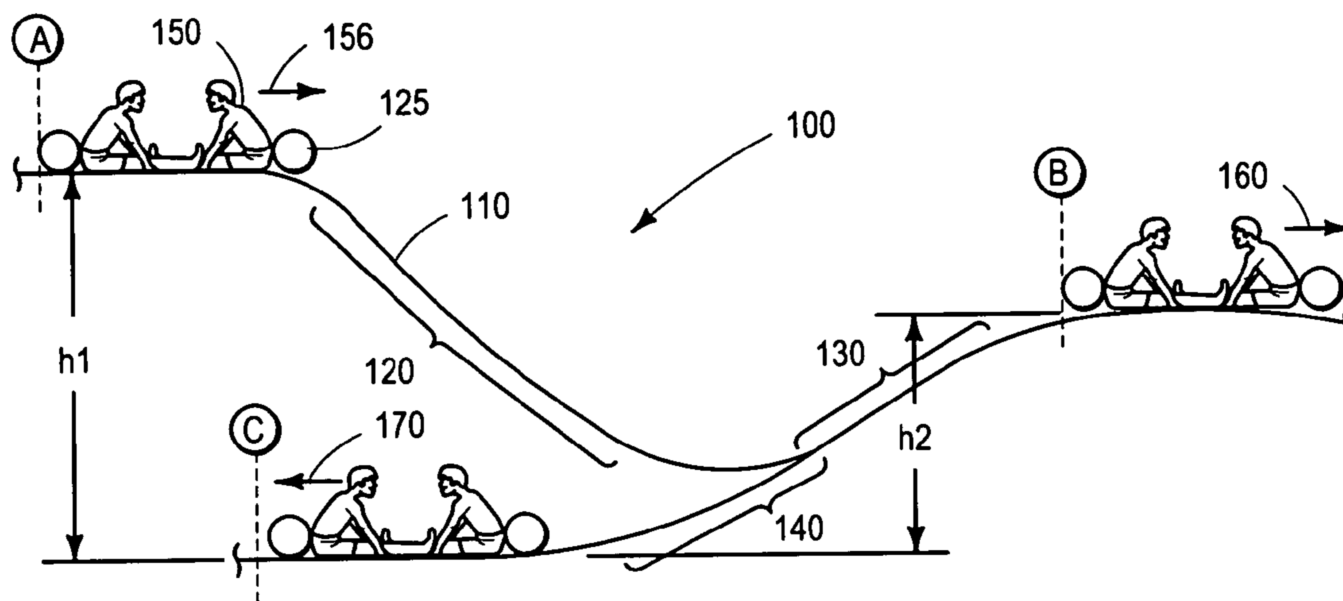
FIG. 1A
