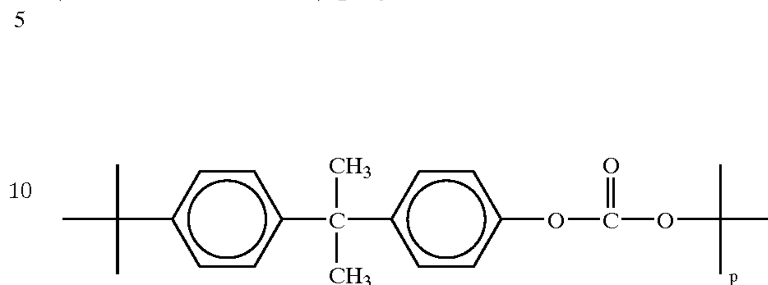
Lexan® 141: p \sim 120 , T_g \sim 150^\circ \text{C} . Makrolon® 5700: p \sim 280 , T_g \sim 157^\circ \text{C} .
