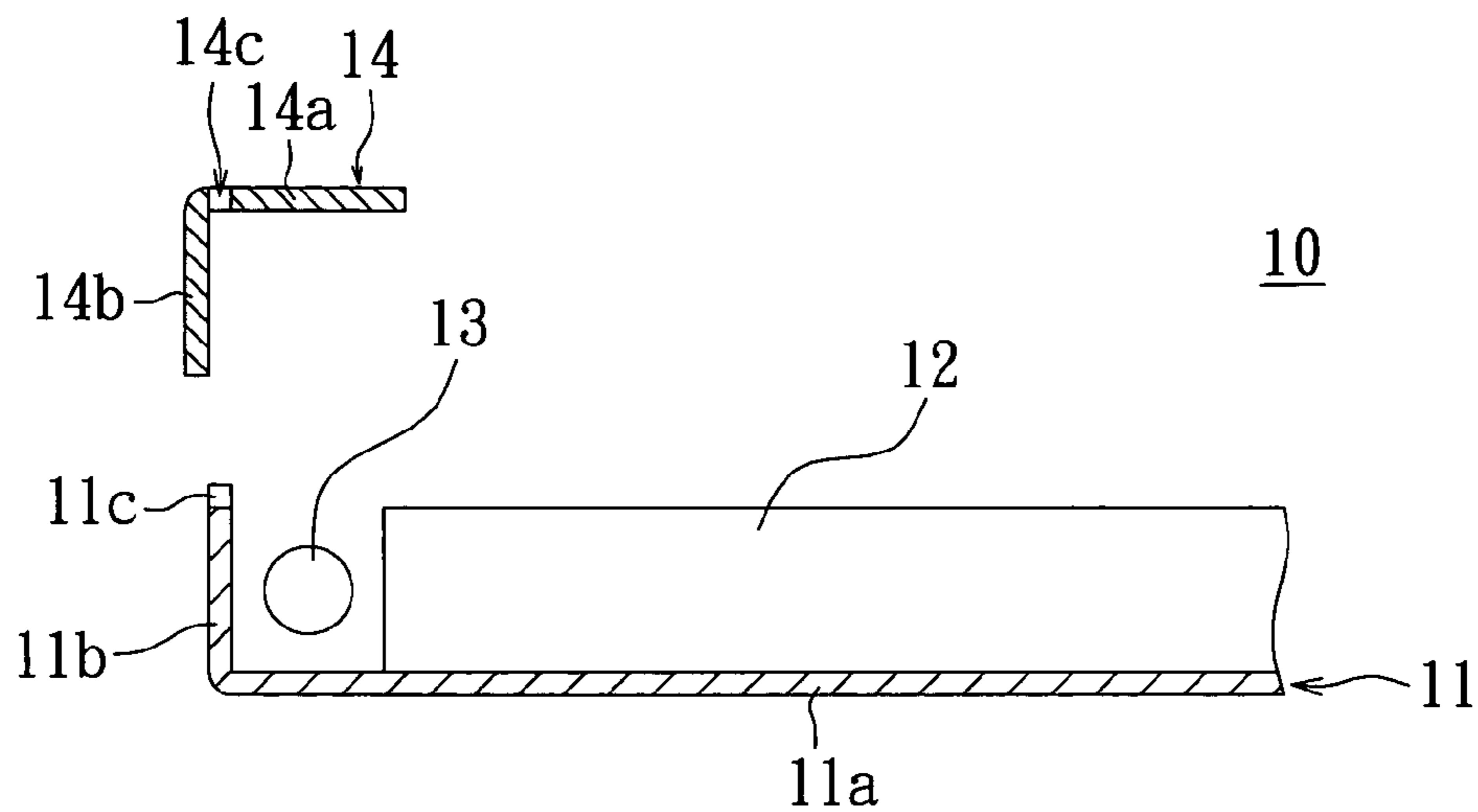
FIG. 1B(PRIOR ART)
