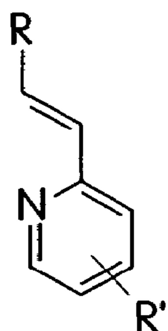
vinylpyridines
