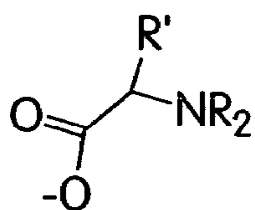
aminoacids
