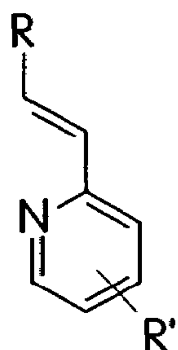
vinylpyridines
