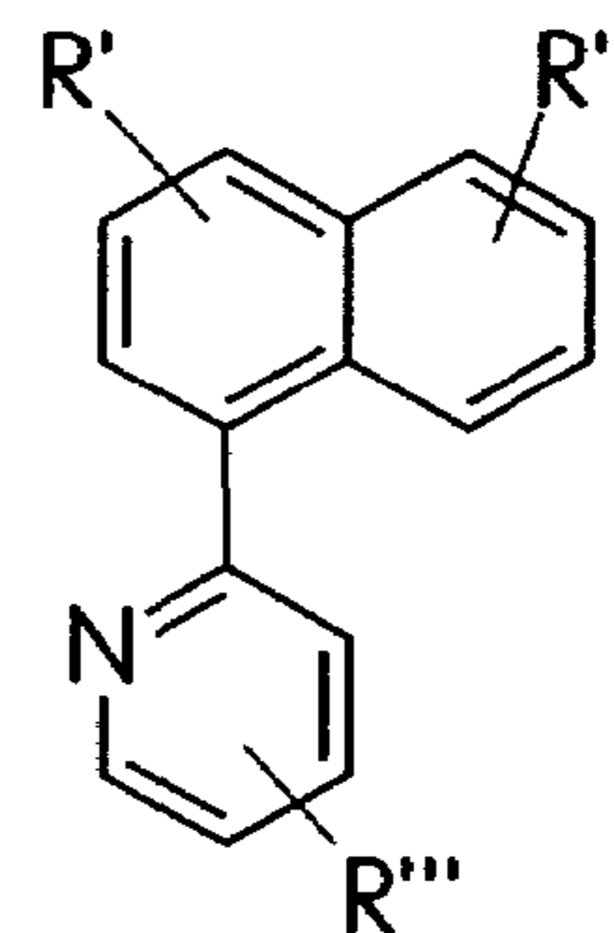
pyridylnaphthalenes
