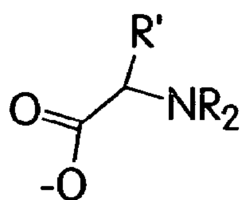
aminoacids
