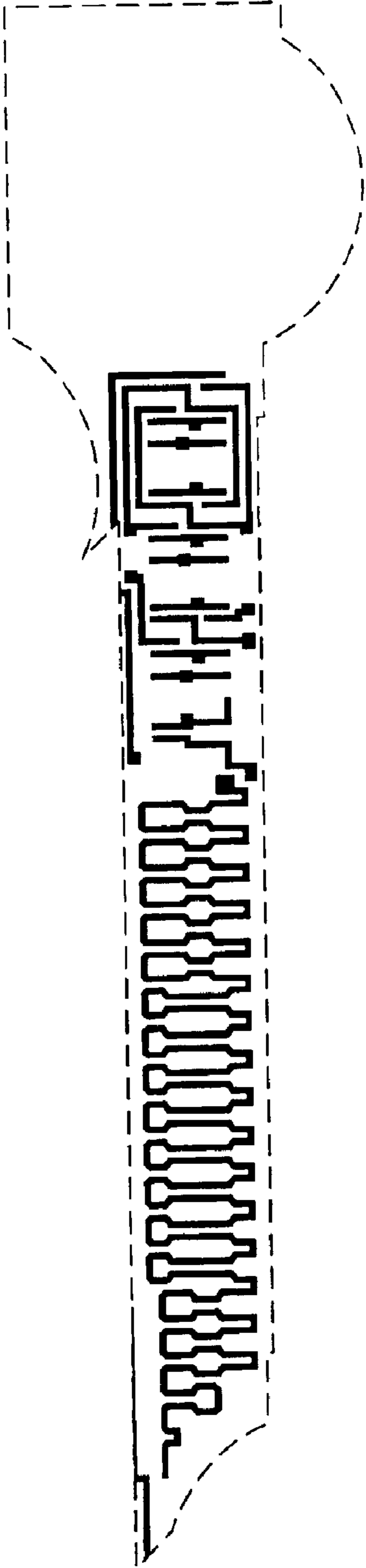
Poly mask
