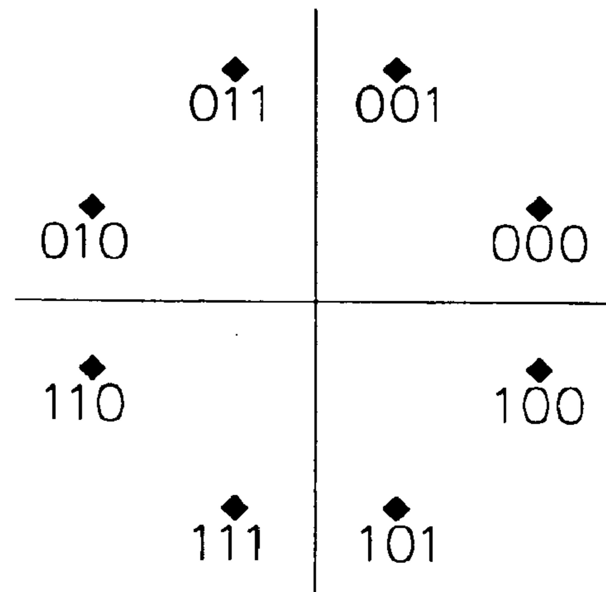
FIG. 12b 3 BITS PER BAUD
