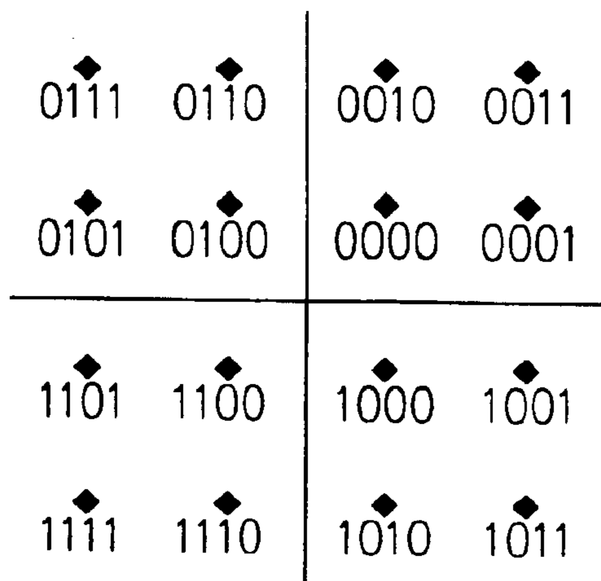
FIG. 12c 4 BITS PER BAUD
