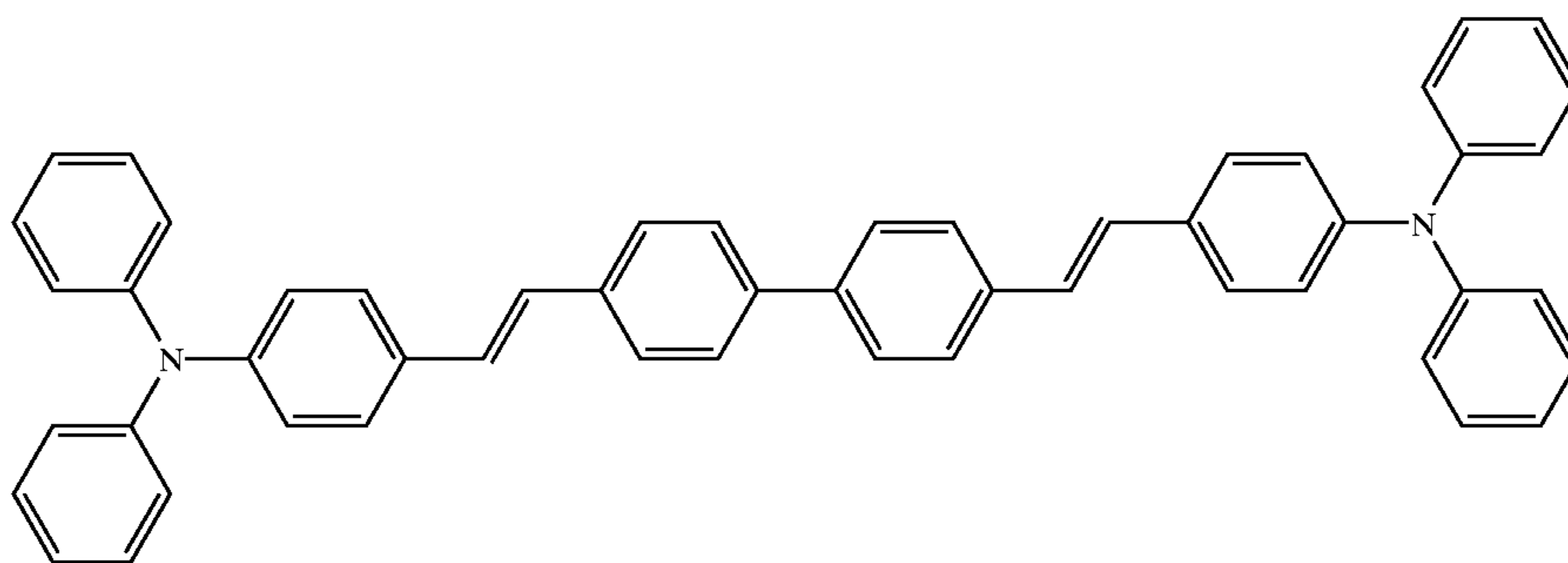
DSA amine
