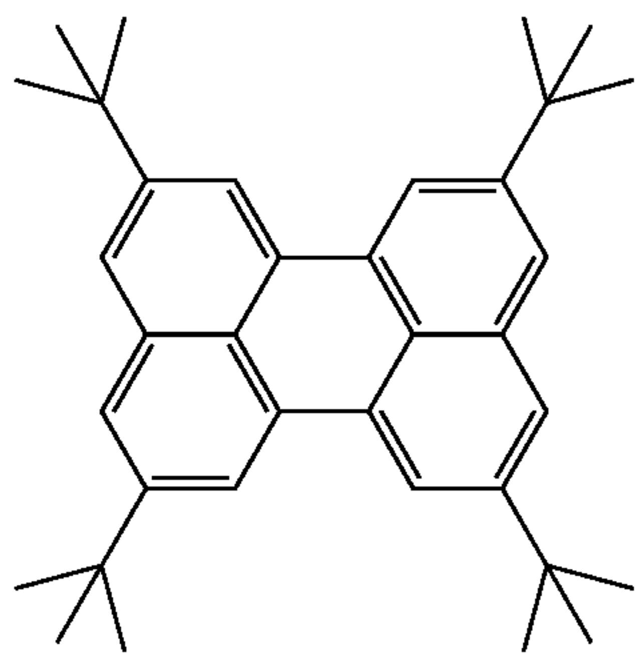
Tetra t-butyl perylene
