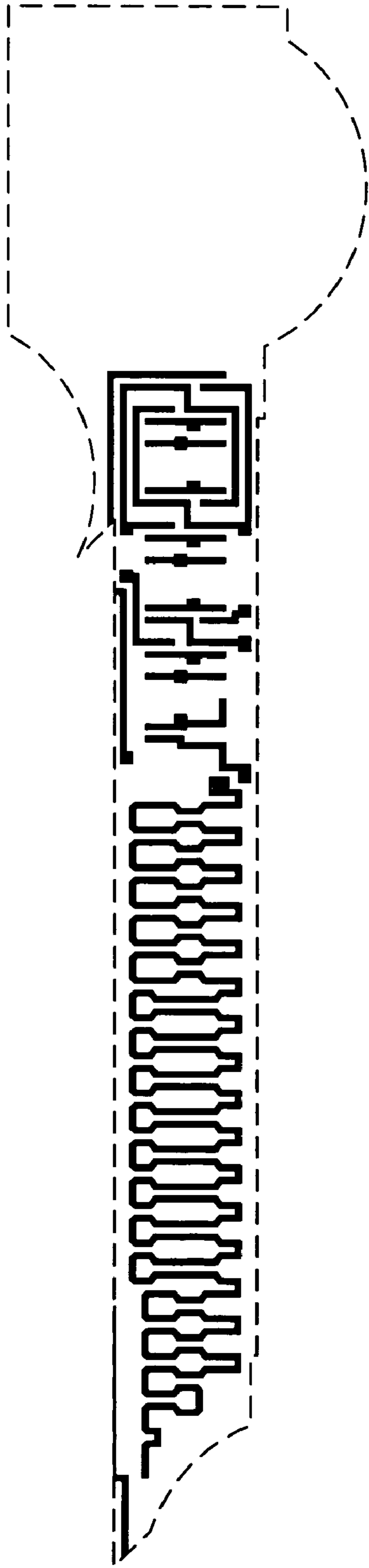
Poly mask
