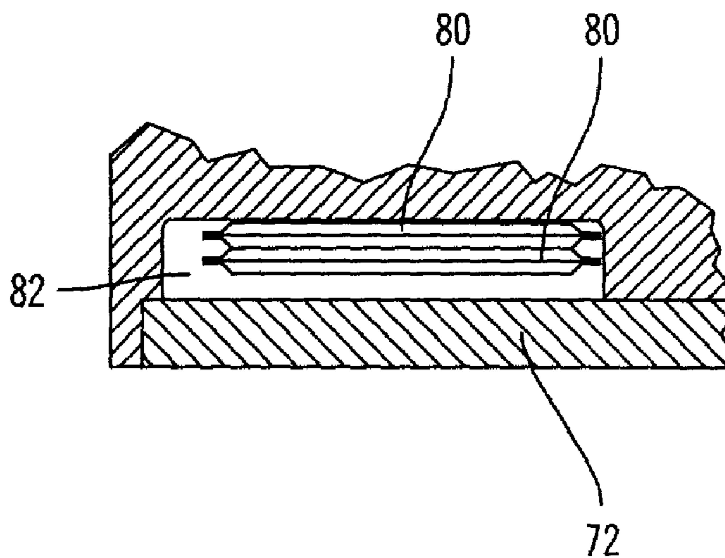
FIG. 10
