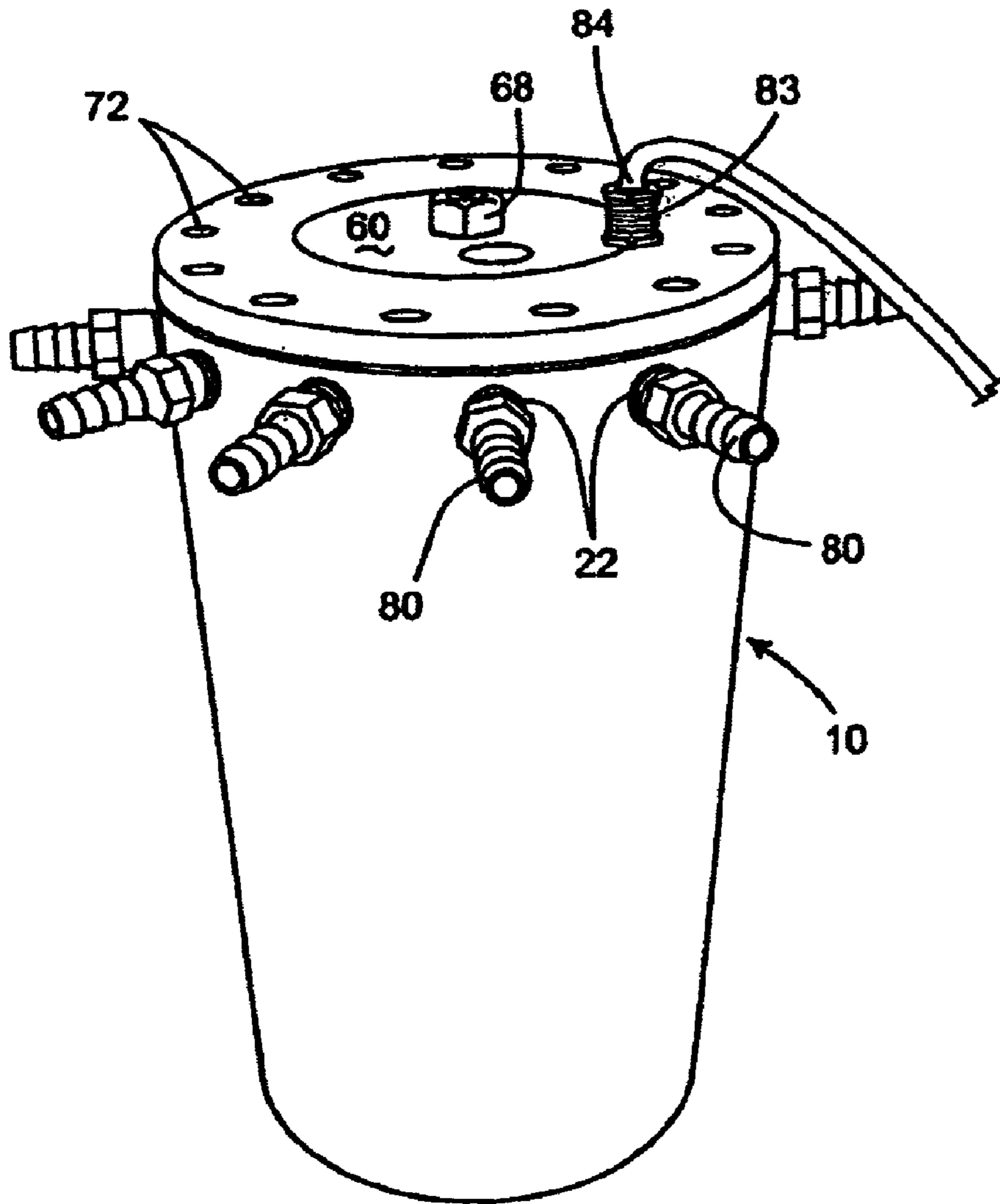
FIG. 1A
