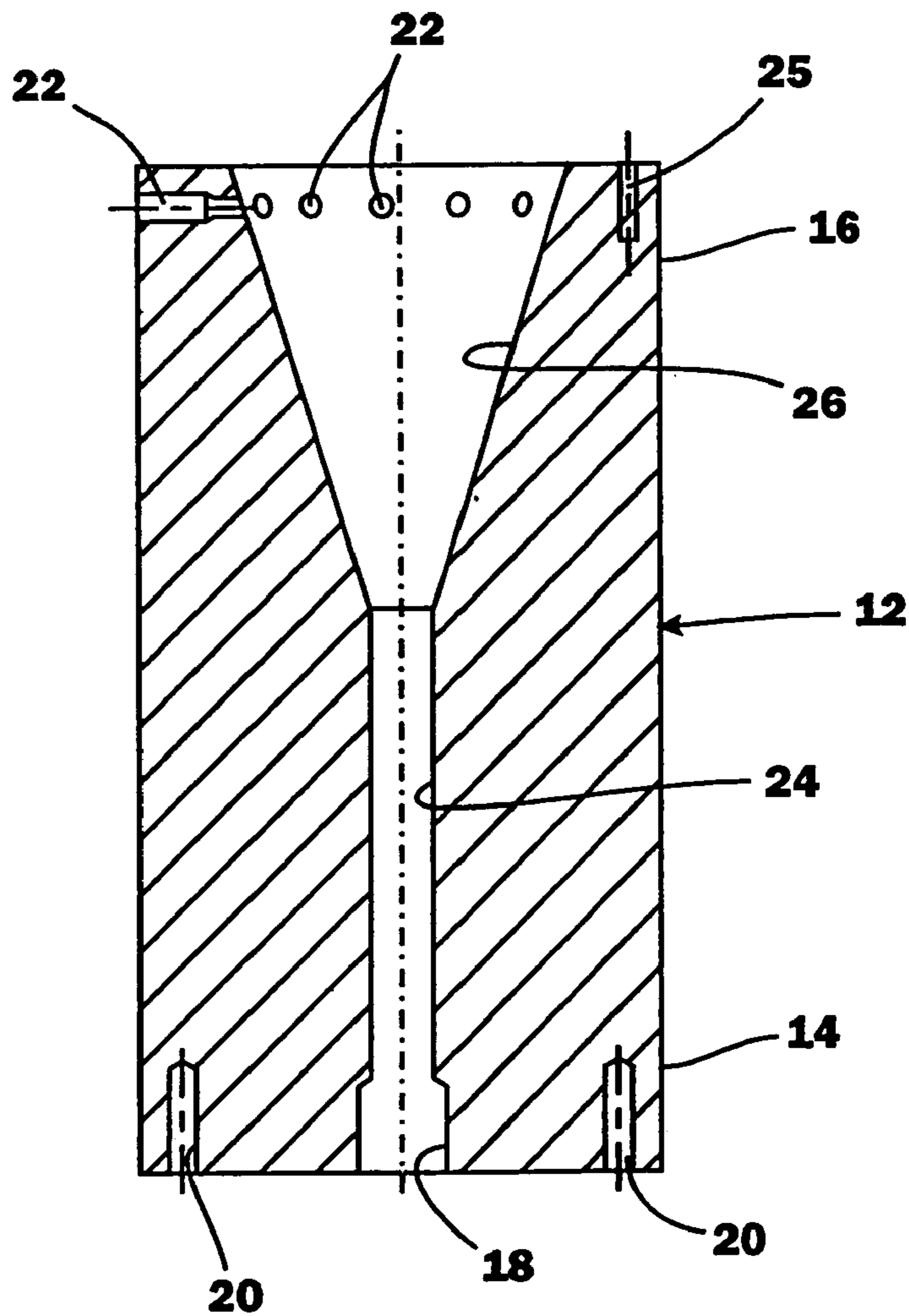
FIG. 2G
