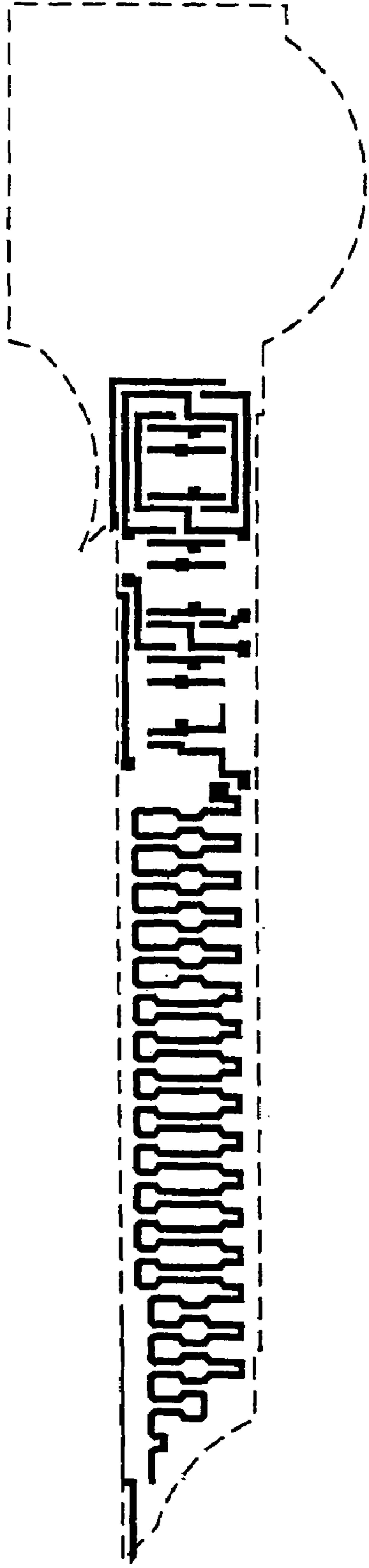
Poly mask
