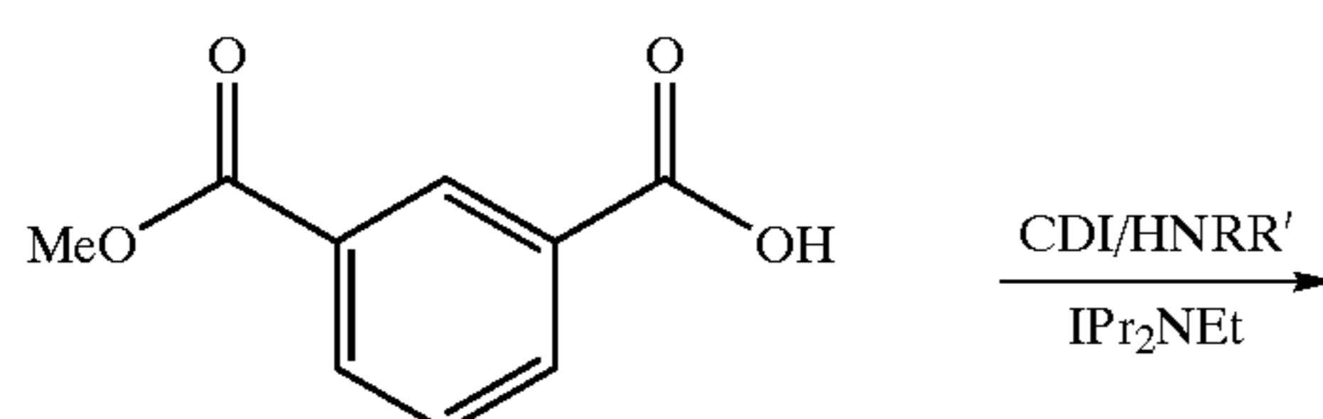
Scheme IVB
