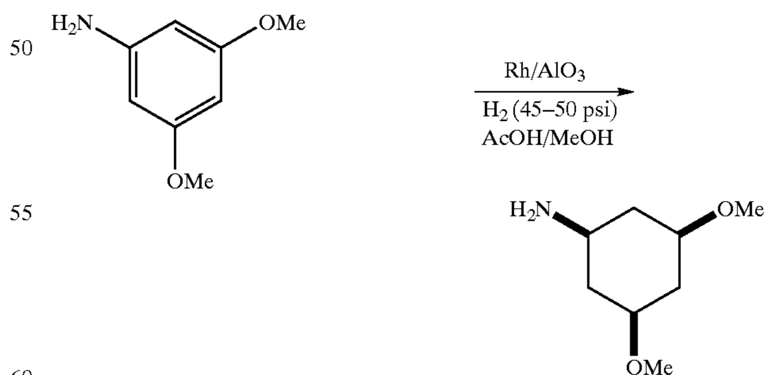
Scheme VI B
