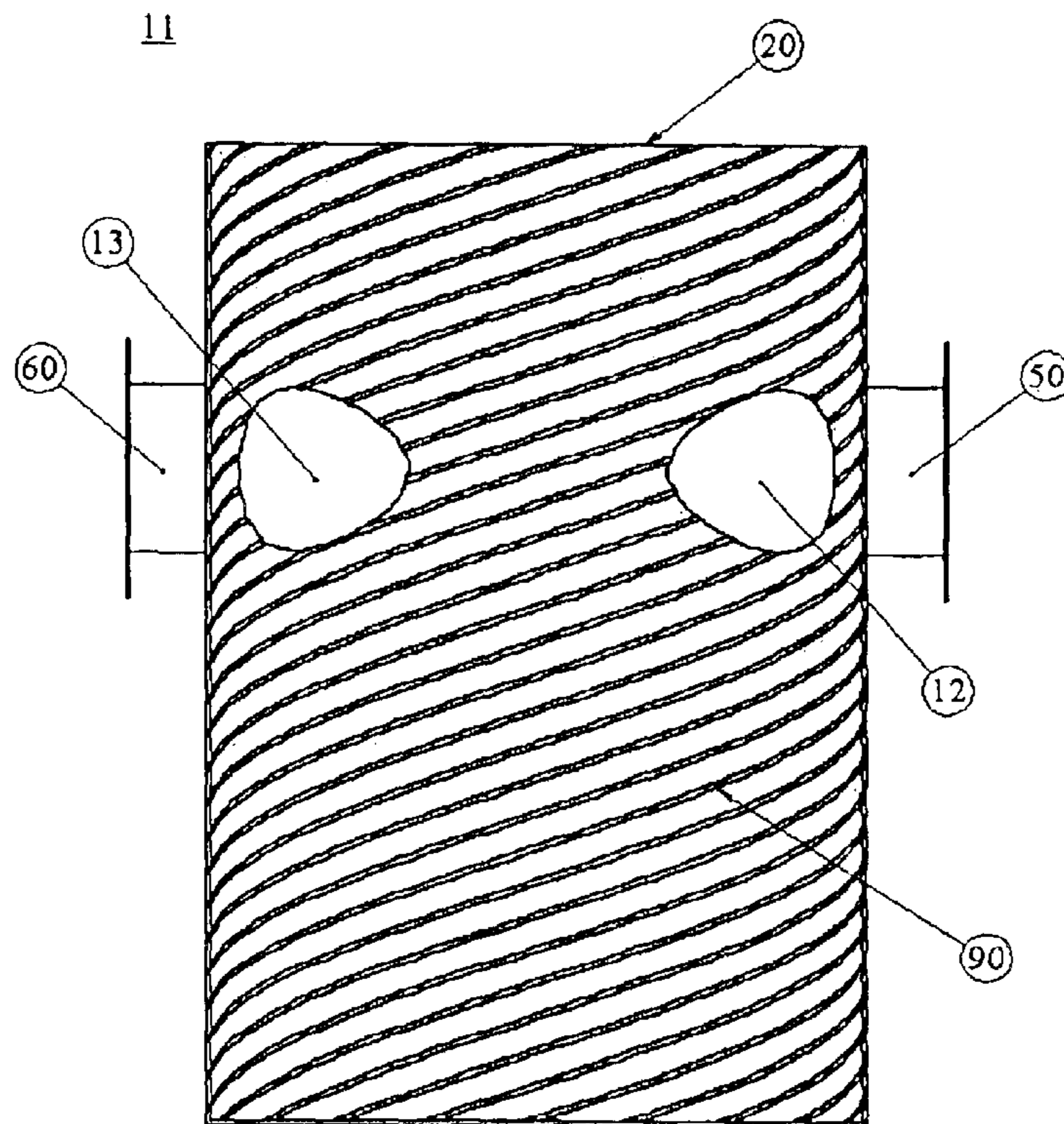
FIG. 8A (SECTION A-A)
