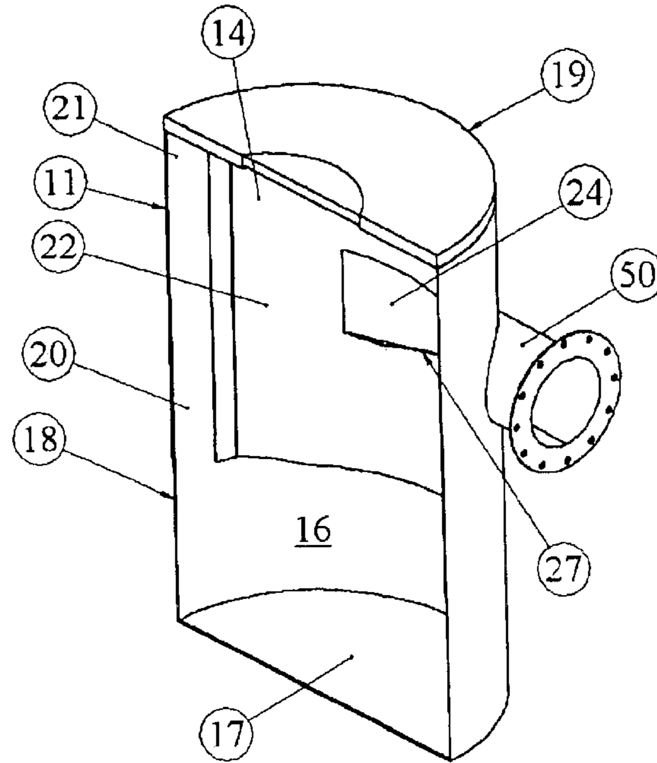
FIG. 2A (SECTION A-A)
