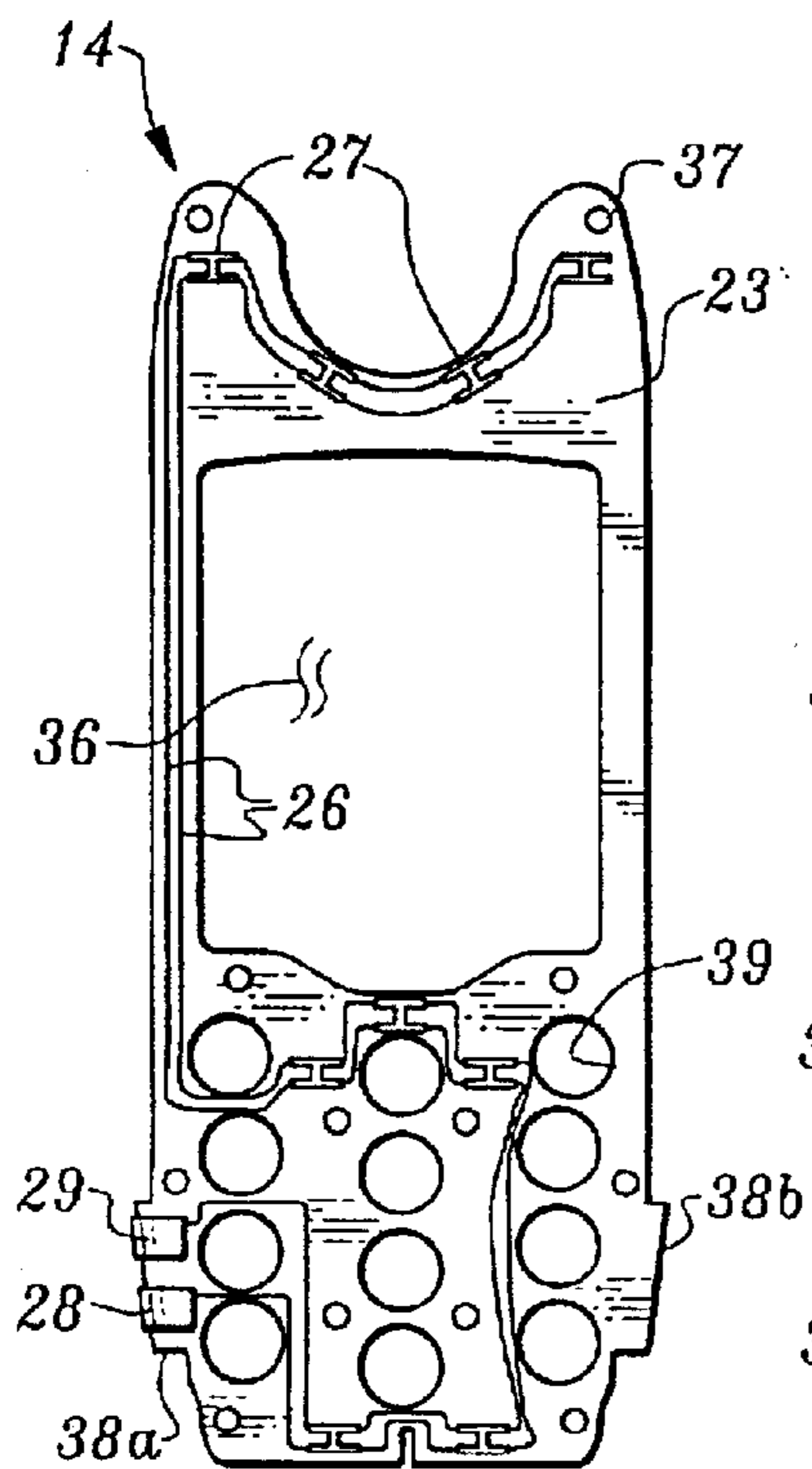
Fig. 2
