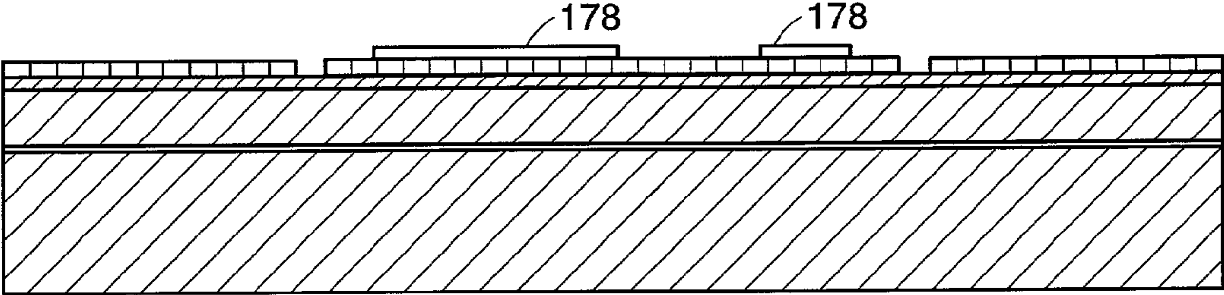
FIG. 24
