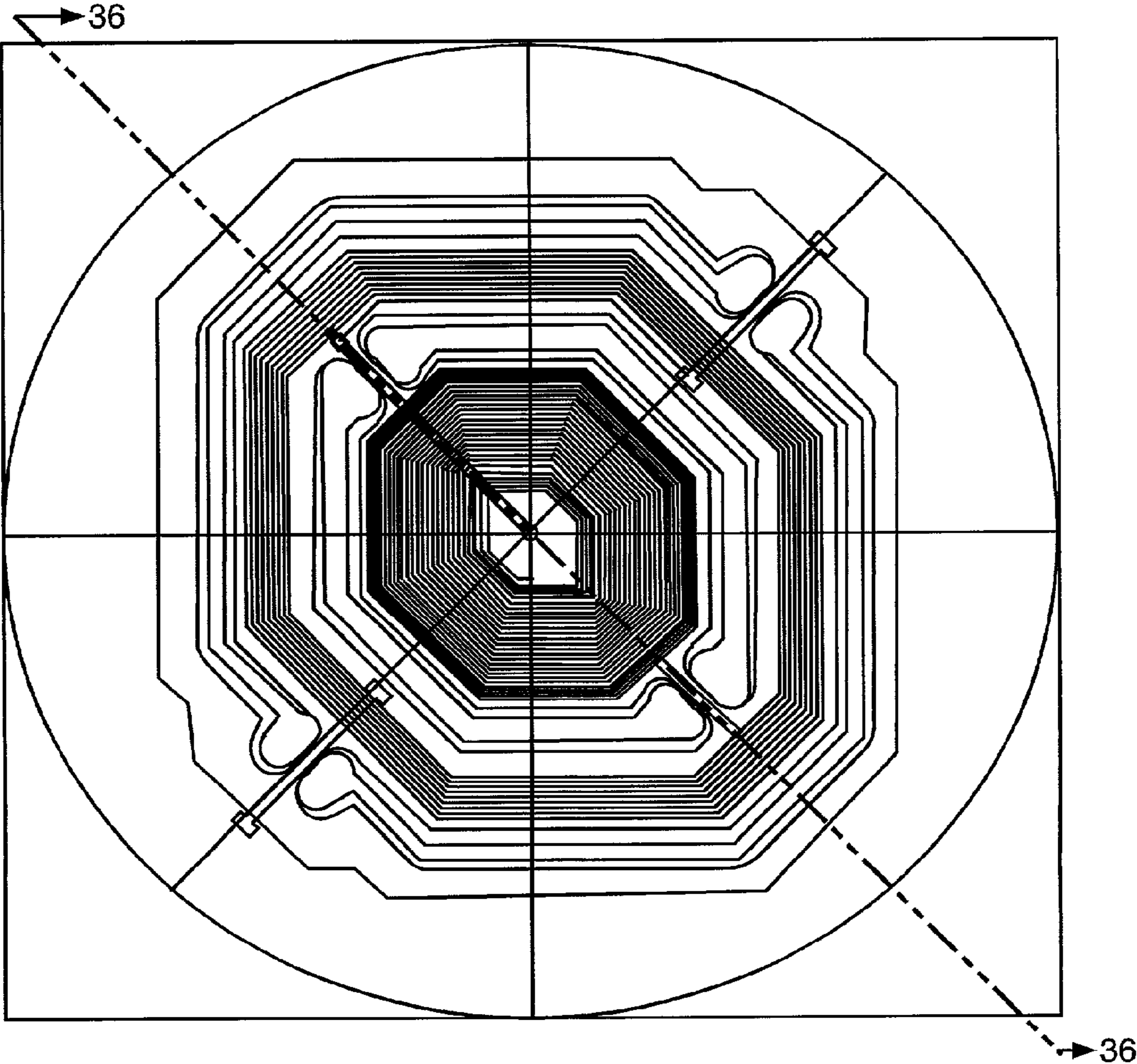
FIG. 35
