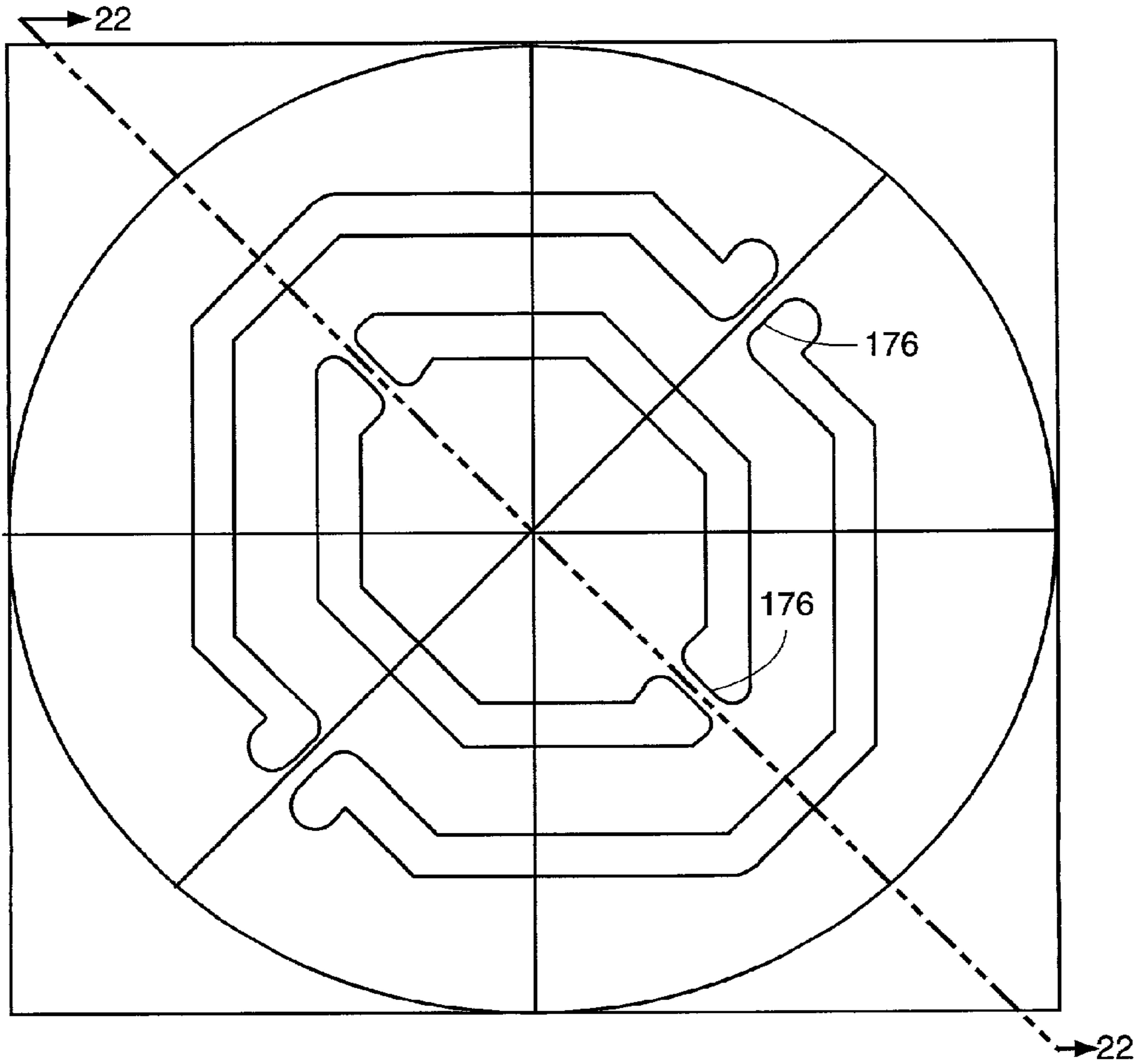
FIG. 21
