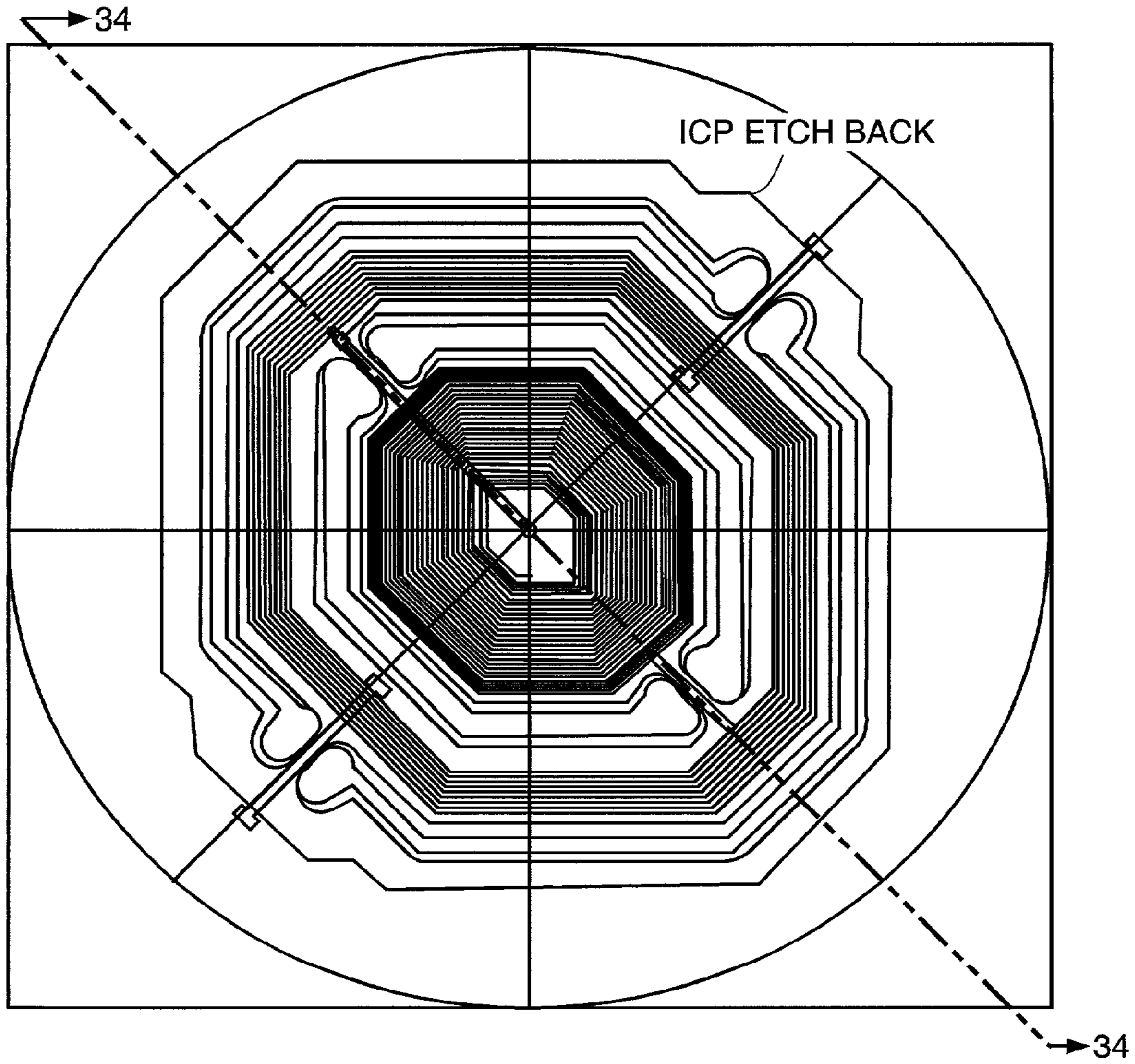
FIG. 33
