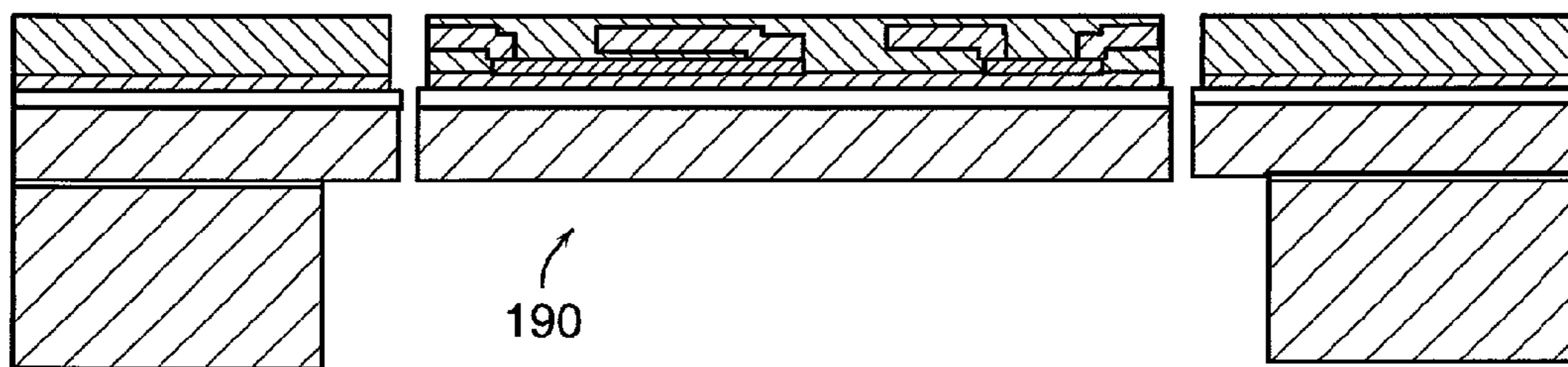
FIG. 34
