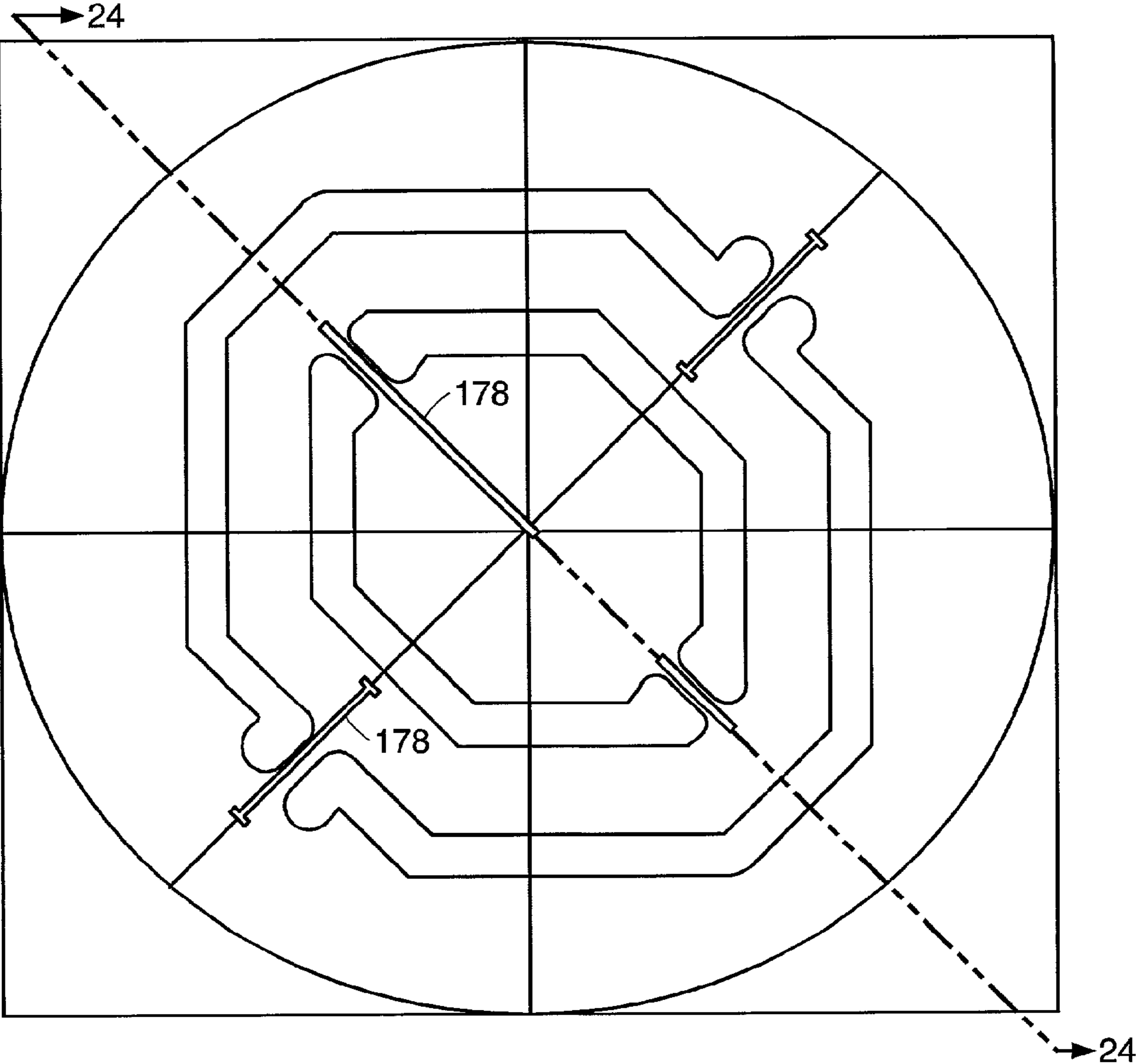
FIG. 23
