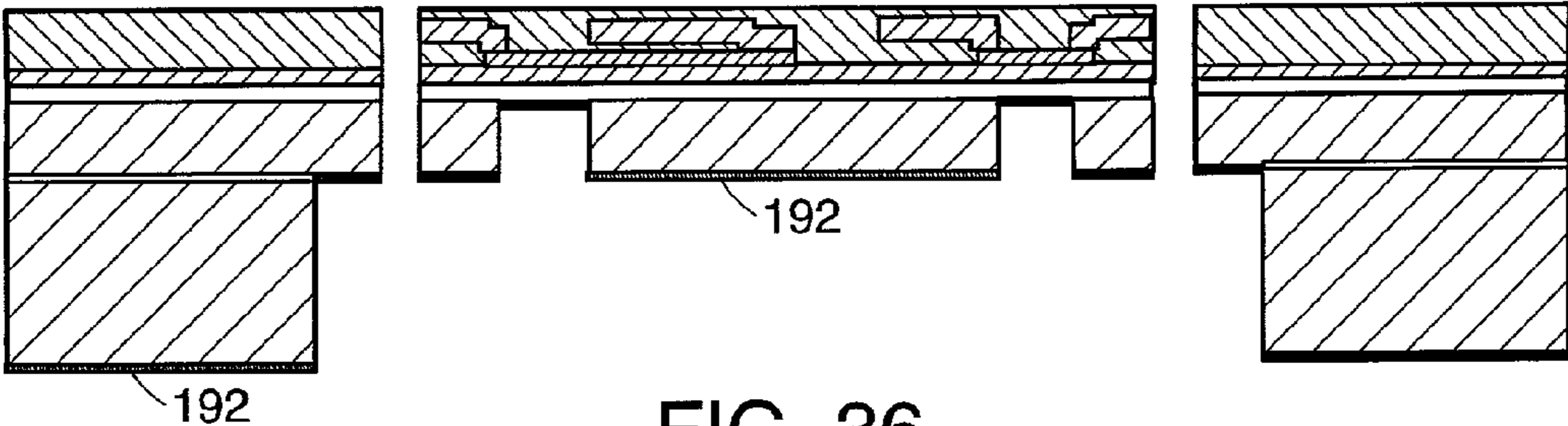
FIG. 36
