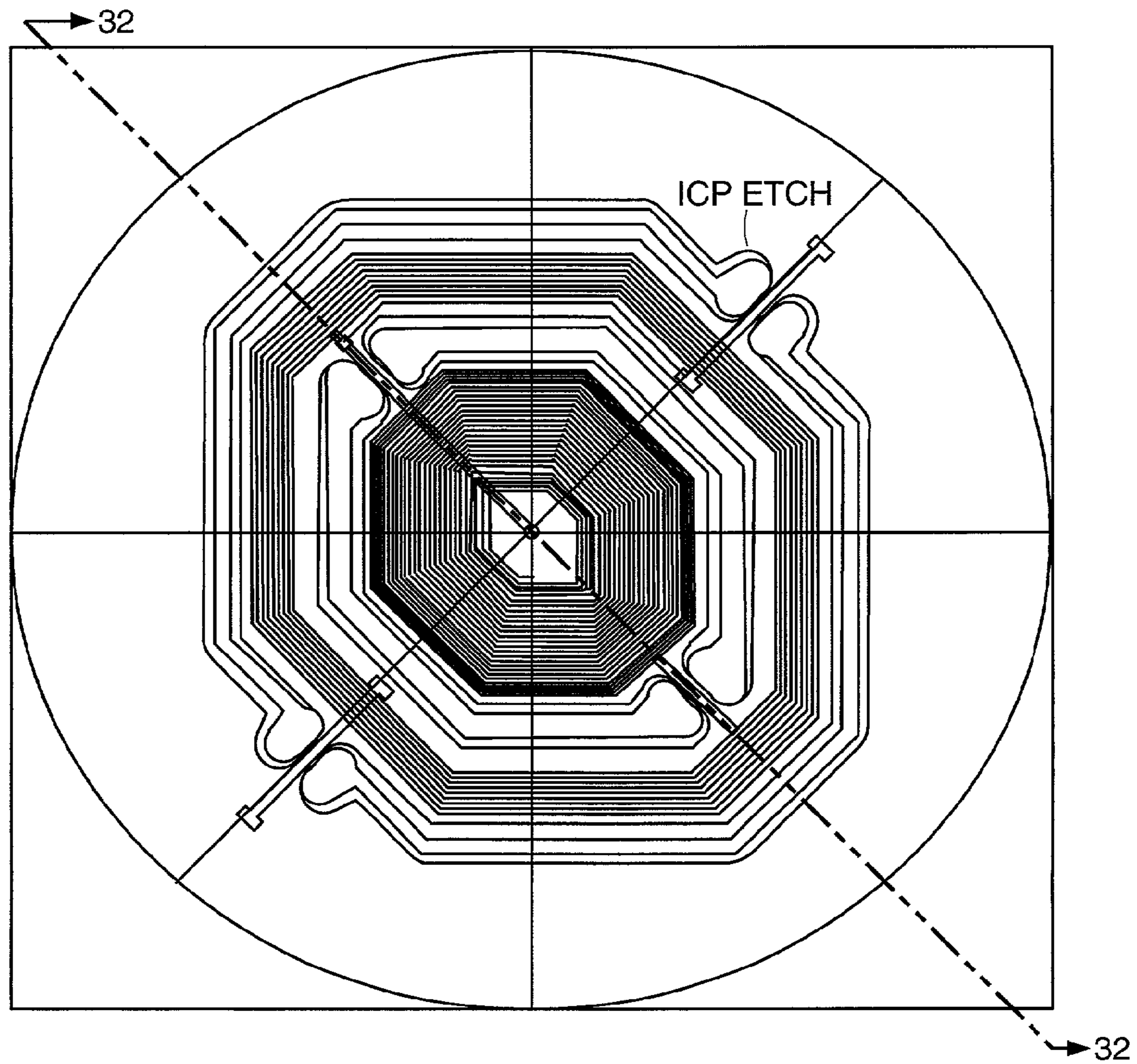
FIG. 31
