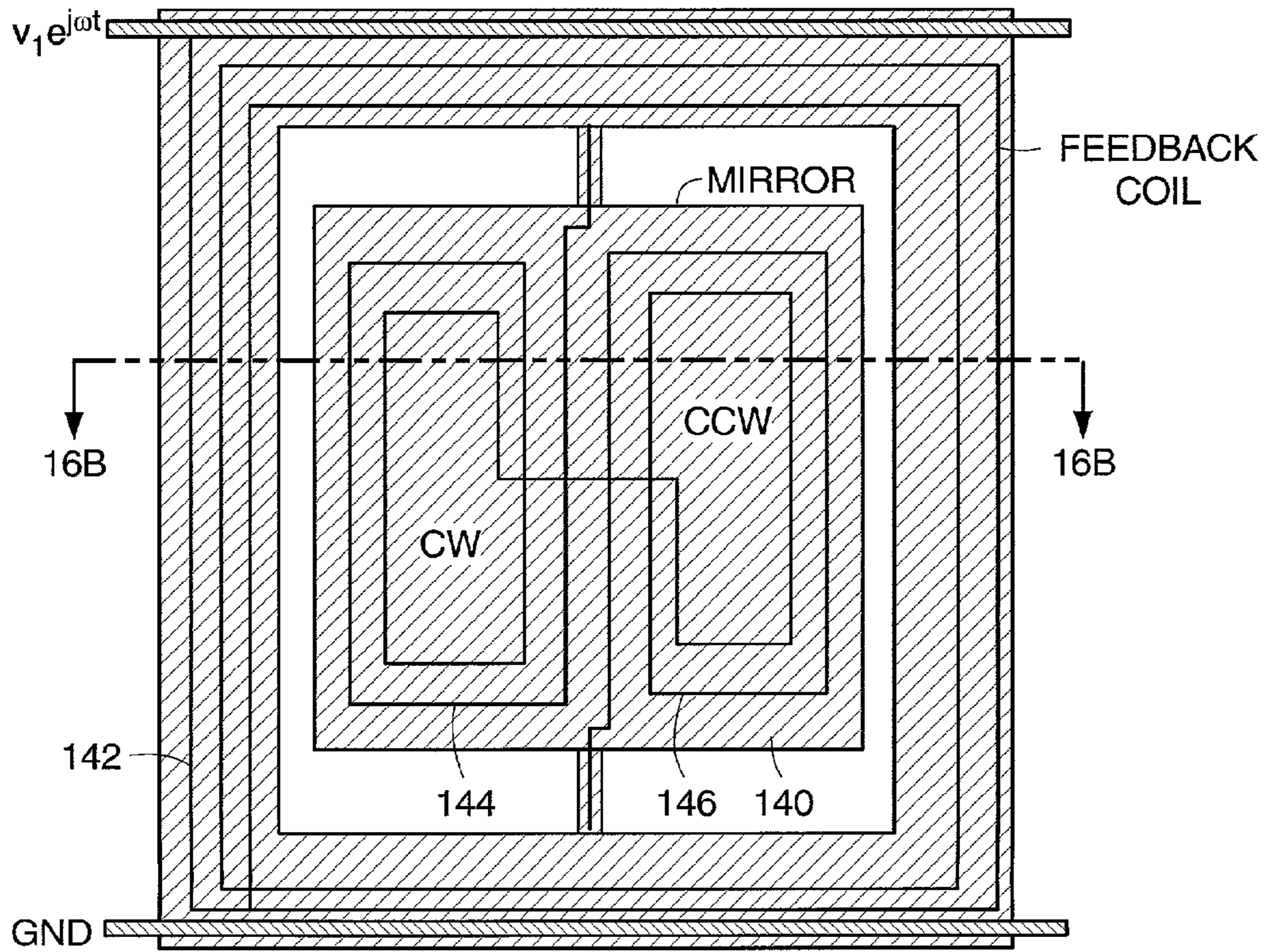
FIG. 16A
