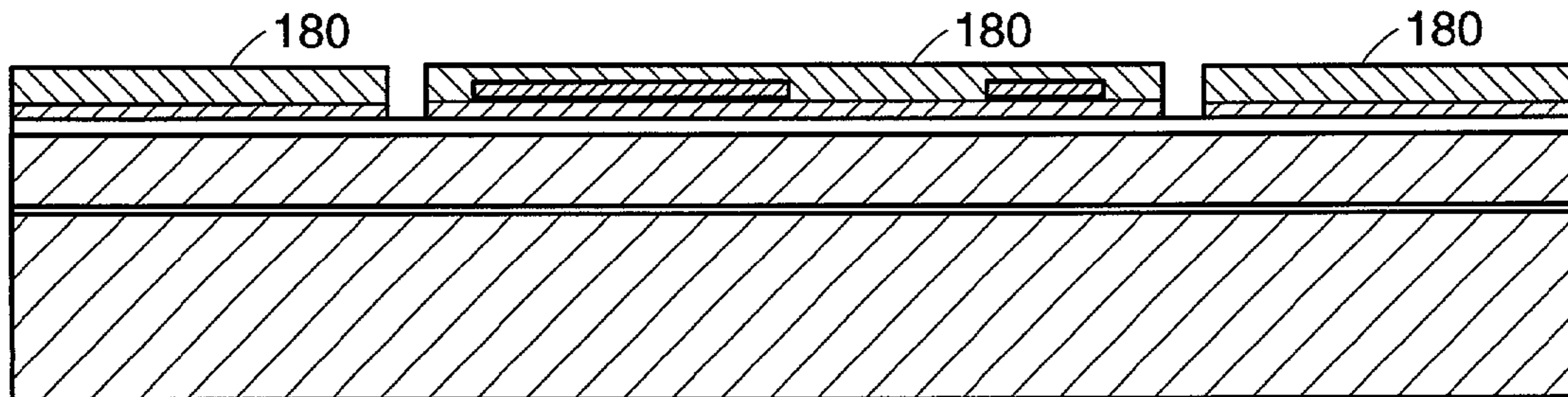
FIG. 26
