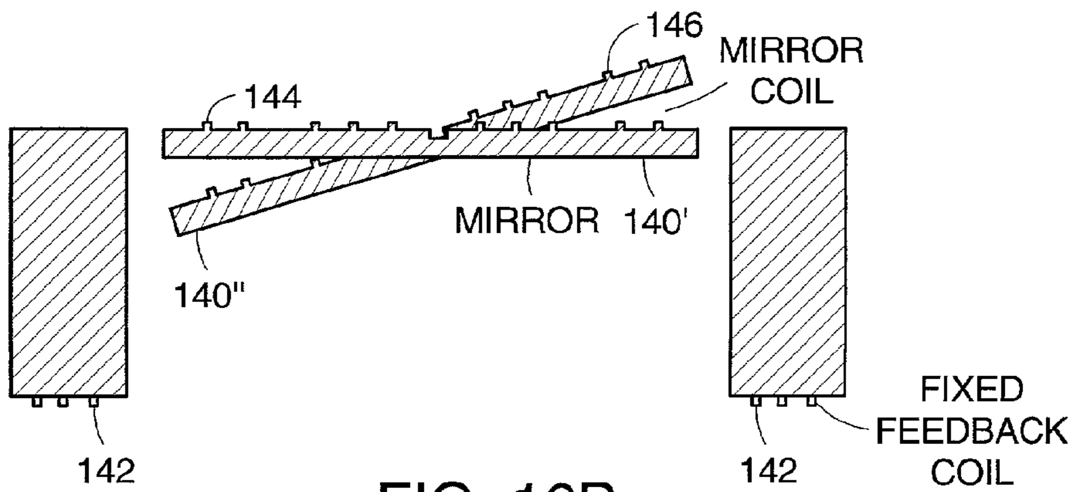
FIG. 16B
