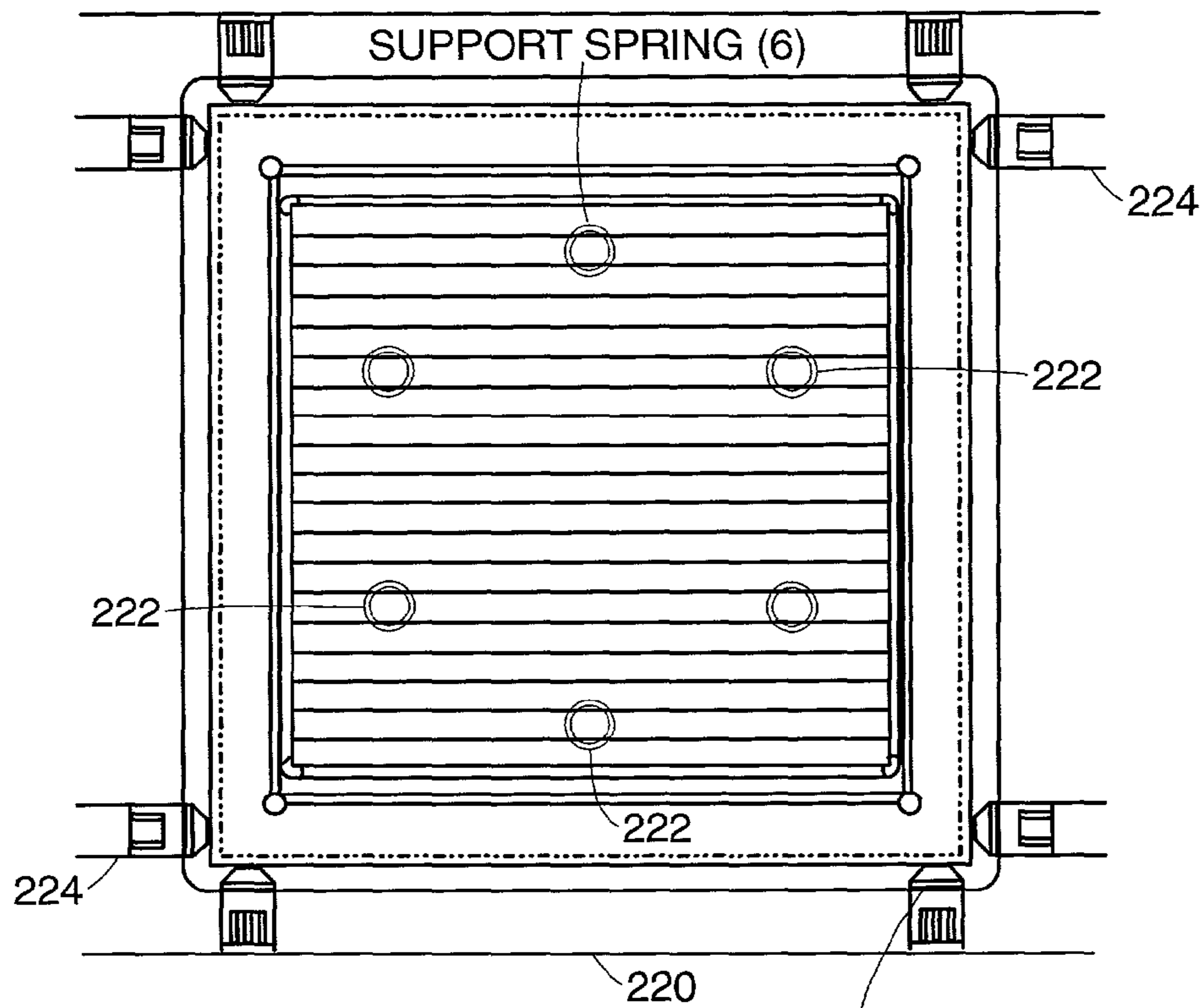
FIG. 40
