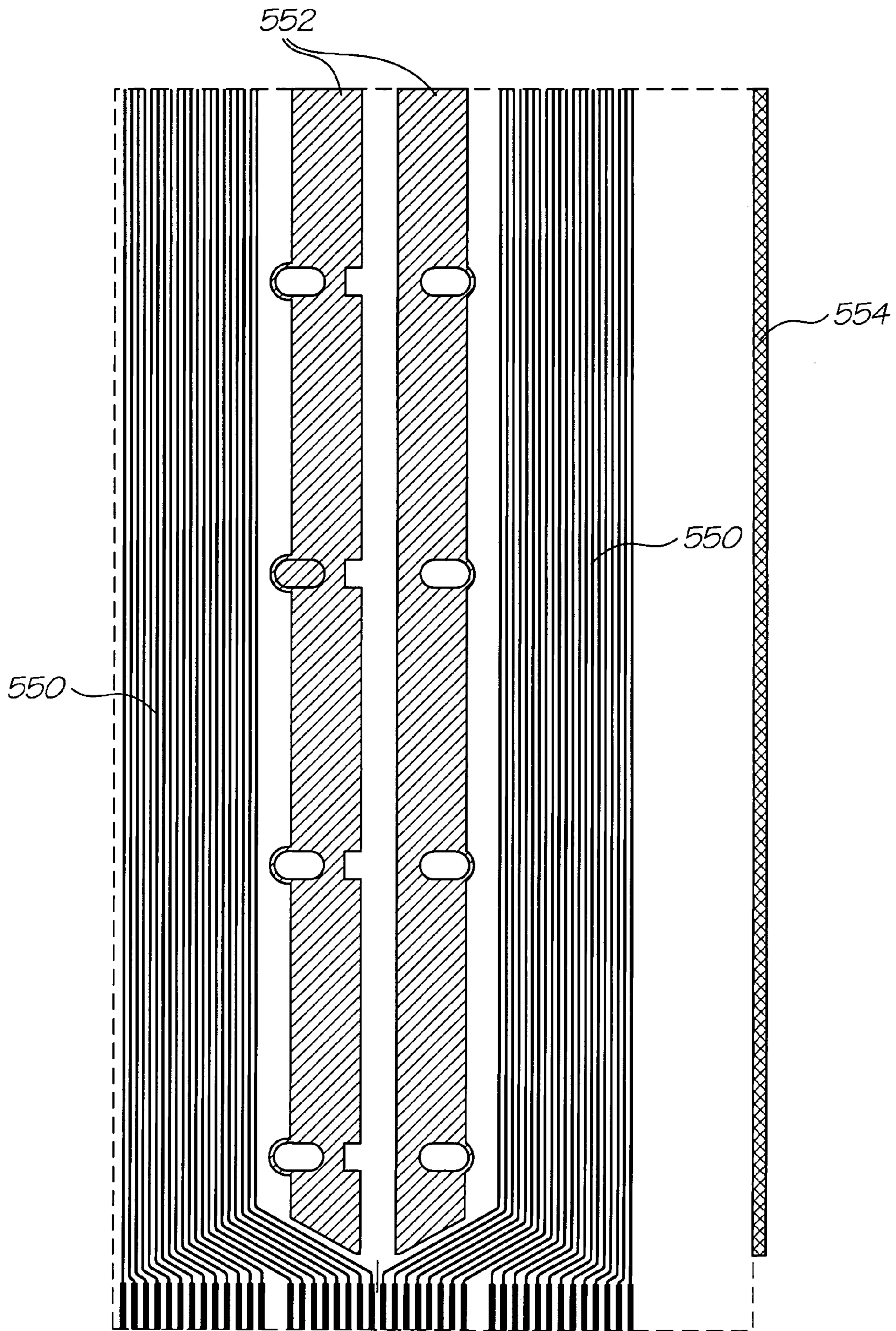
FIG. 102
