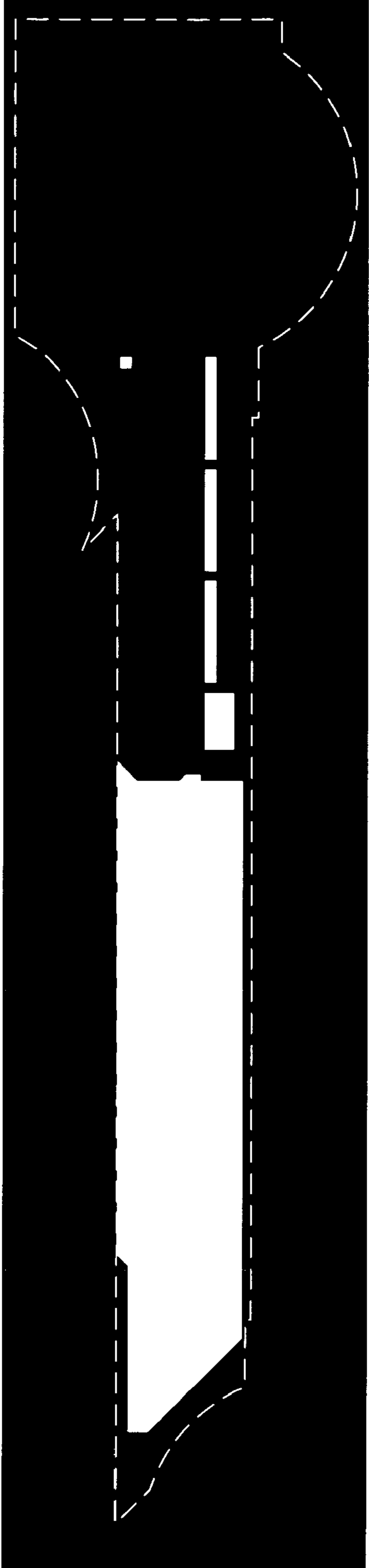
p+ mask
