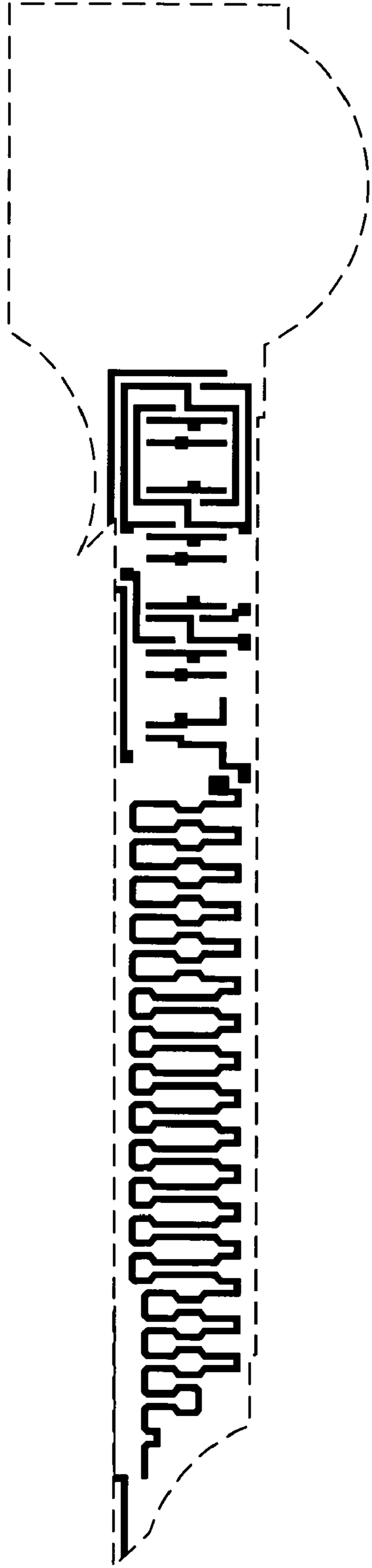
Poly mask
