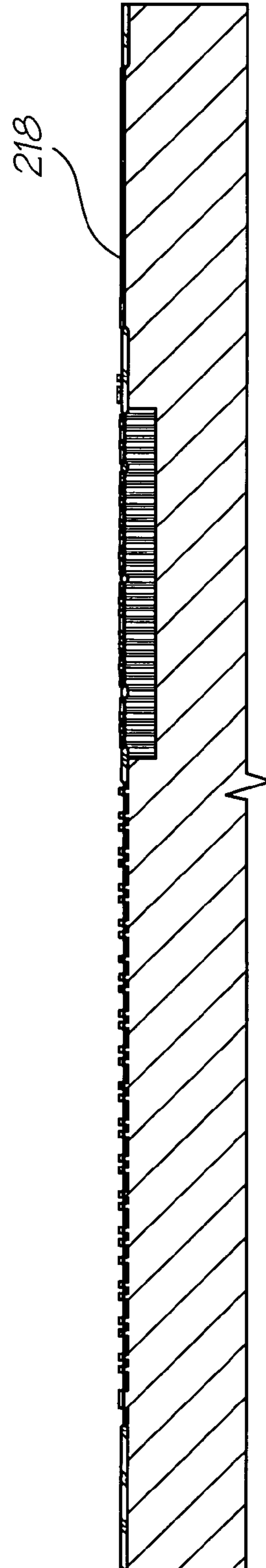
p+ implant
