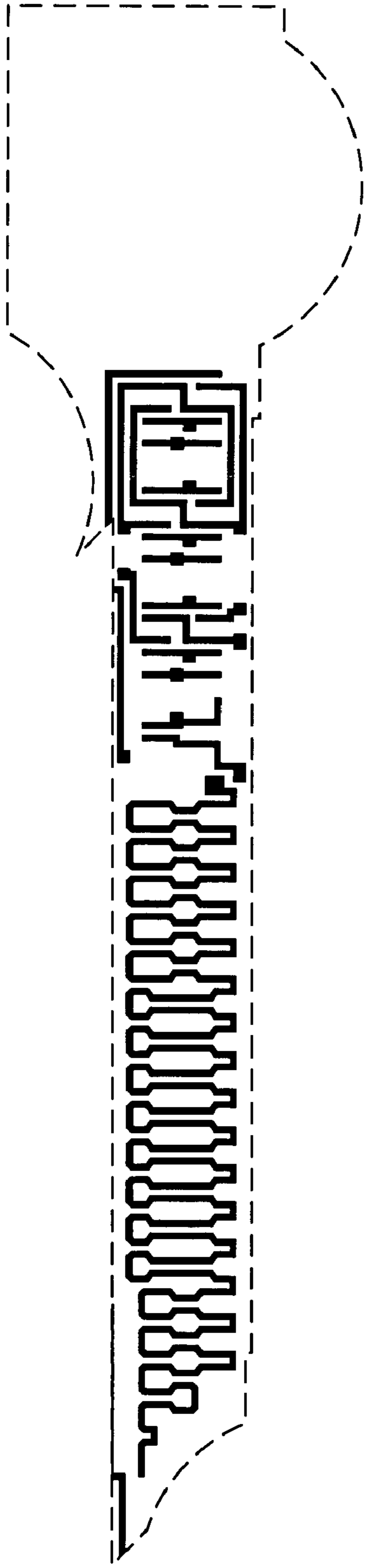
Poly mask
