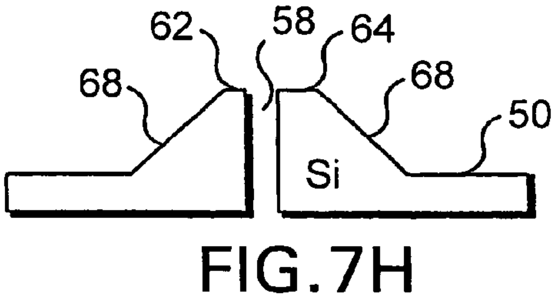
STEP 8. REMOVE NITRIDE LAYER
