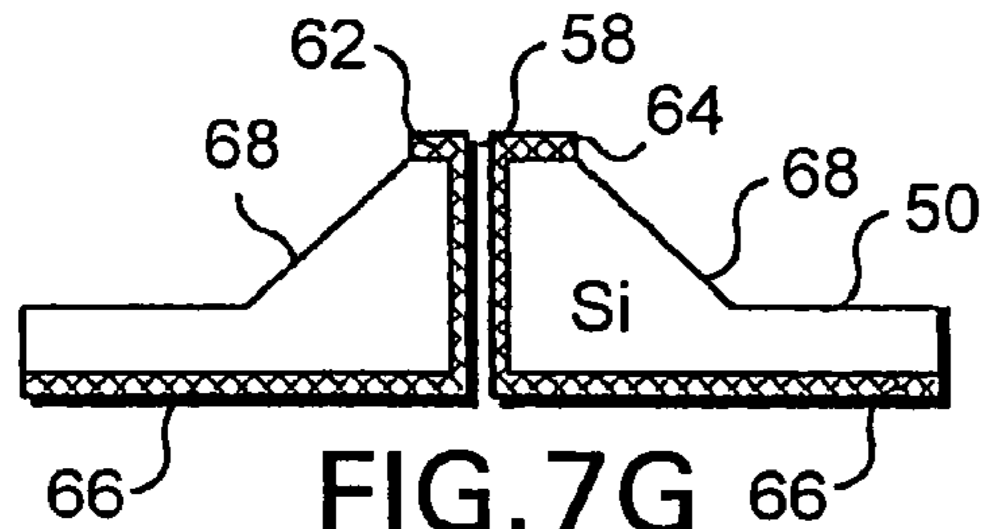
STEP 7. ANISOTROPIC ETCH
