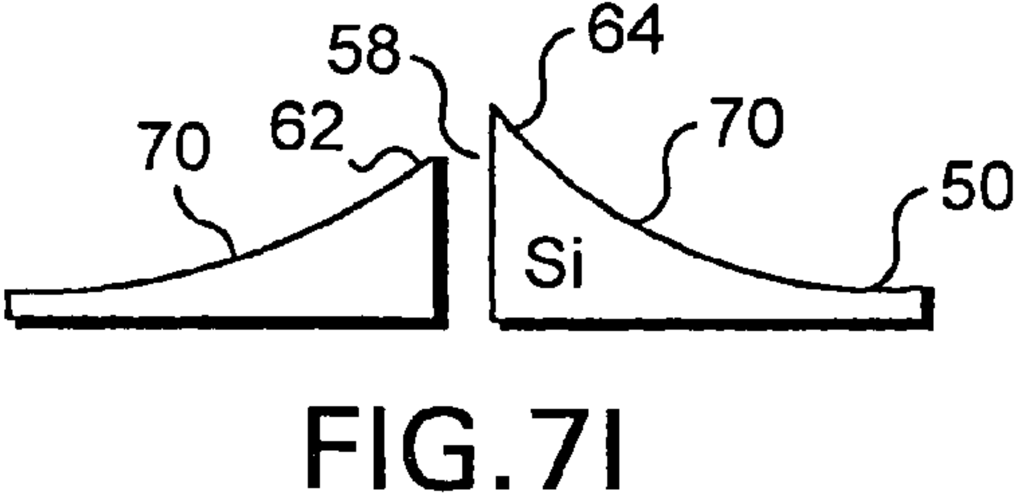
STEP 8. ISOTROPIC ETCH
