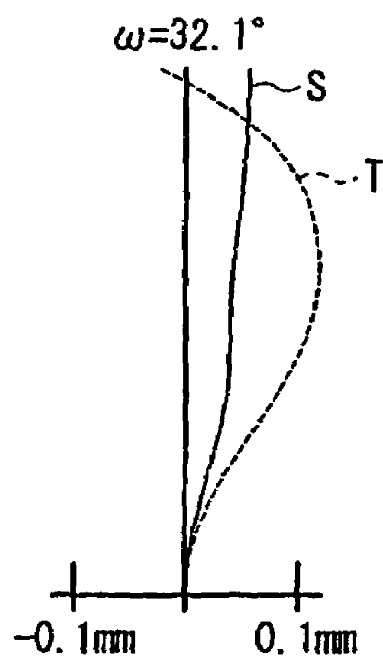
Astigmatism Fig. 3B
