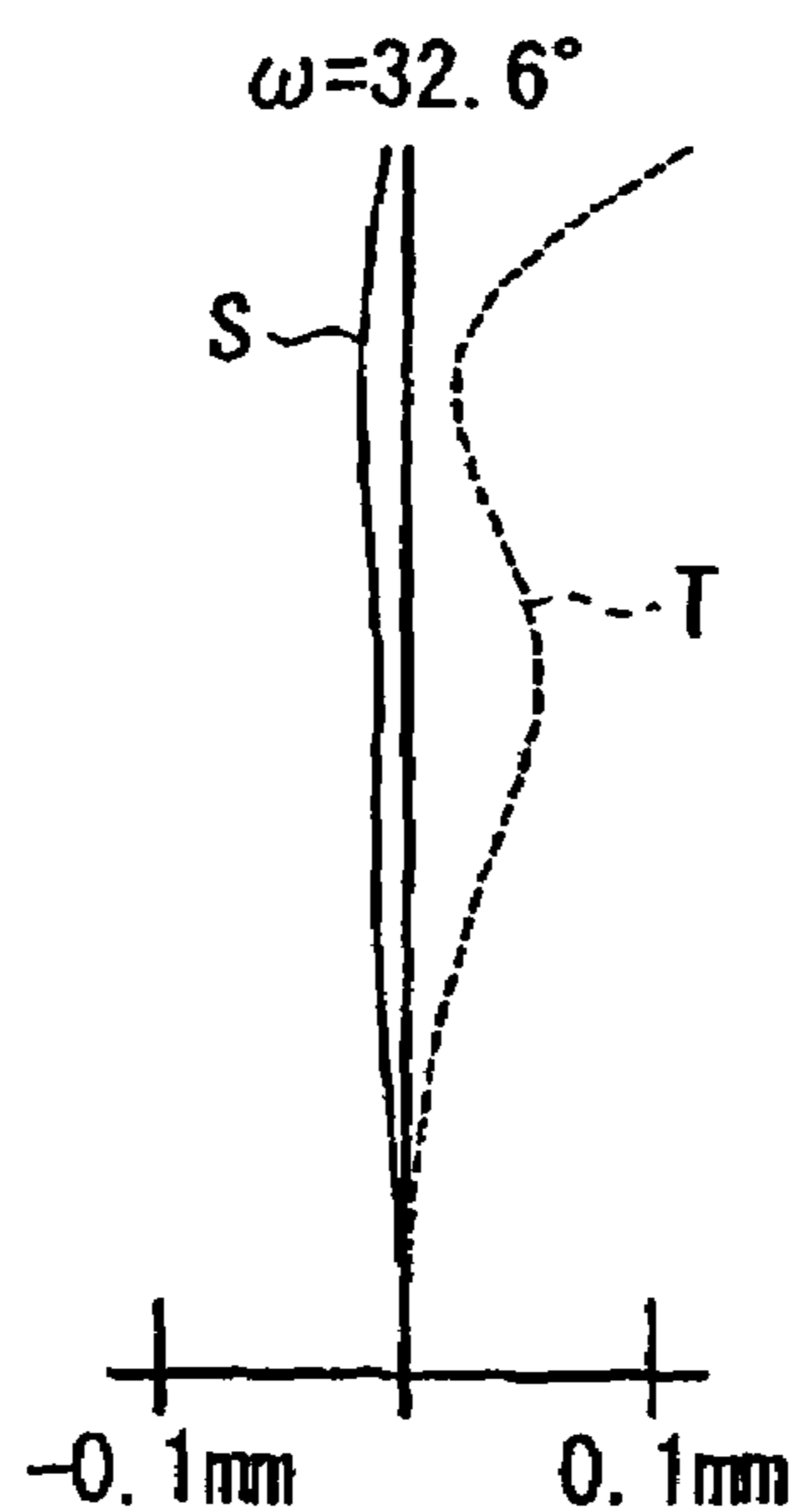
Astigmatism Fig. 4B
