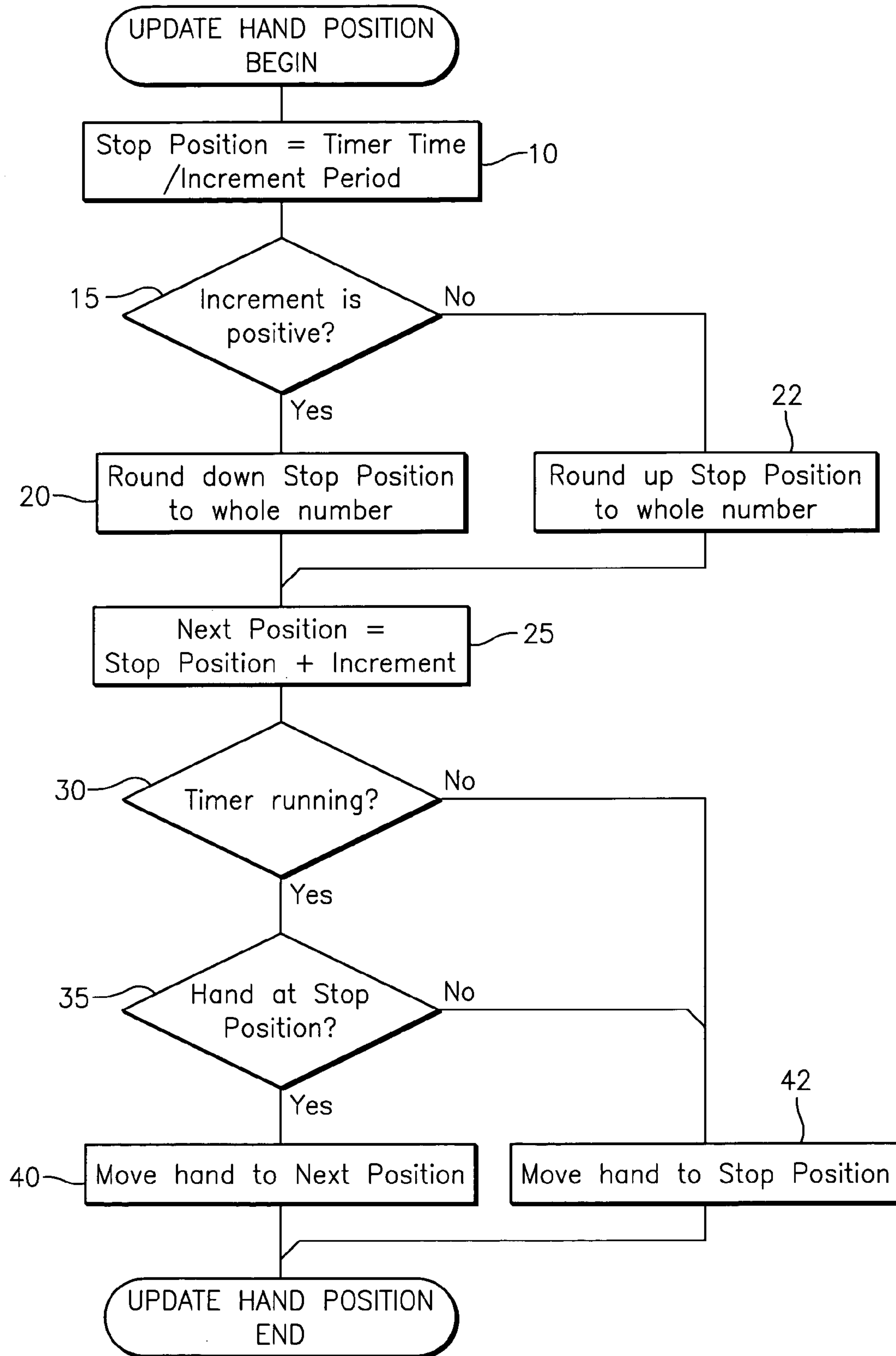
FIG. 8C
