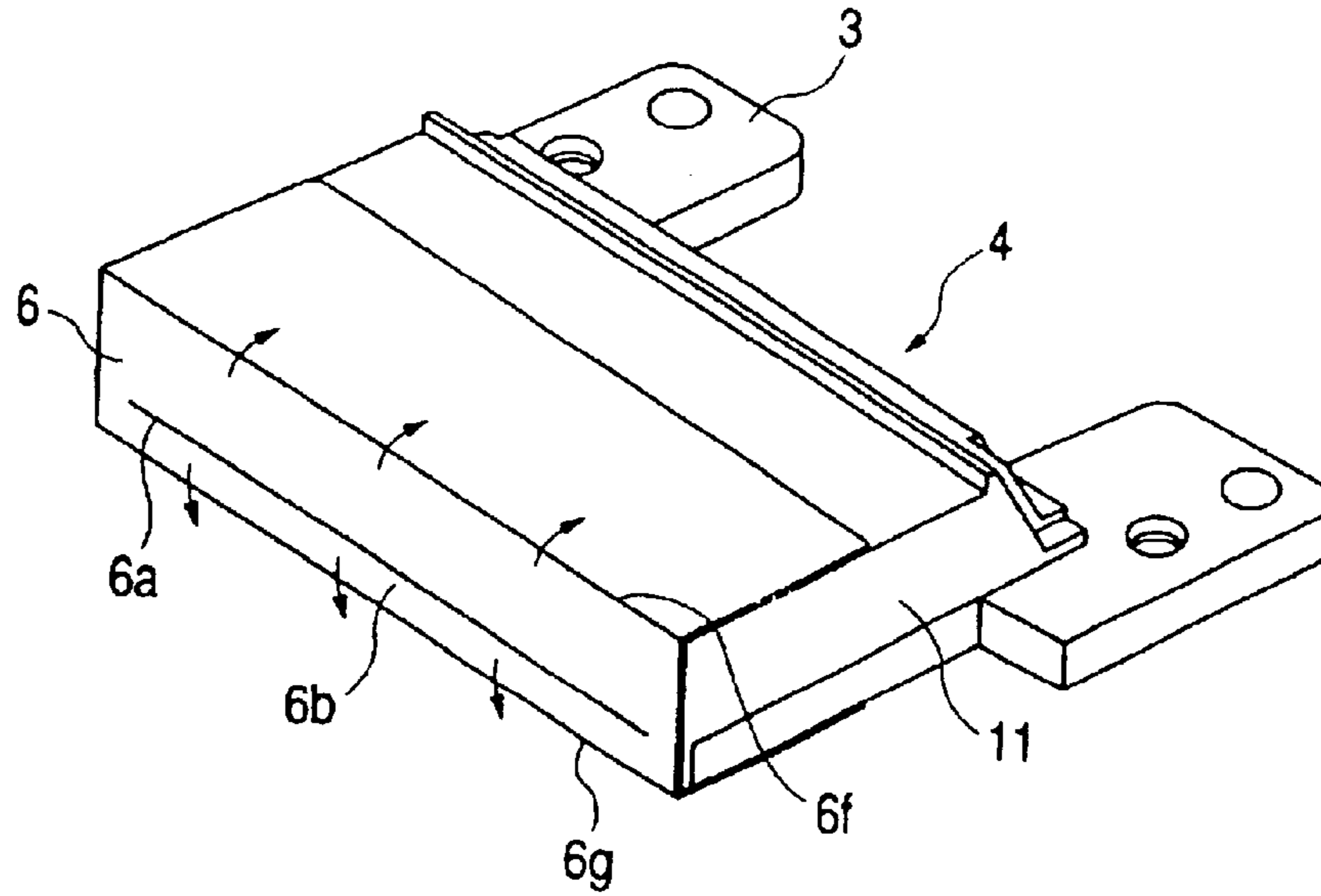
FIG. 33
