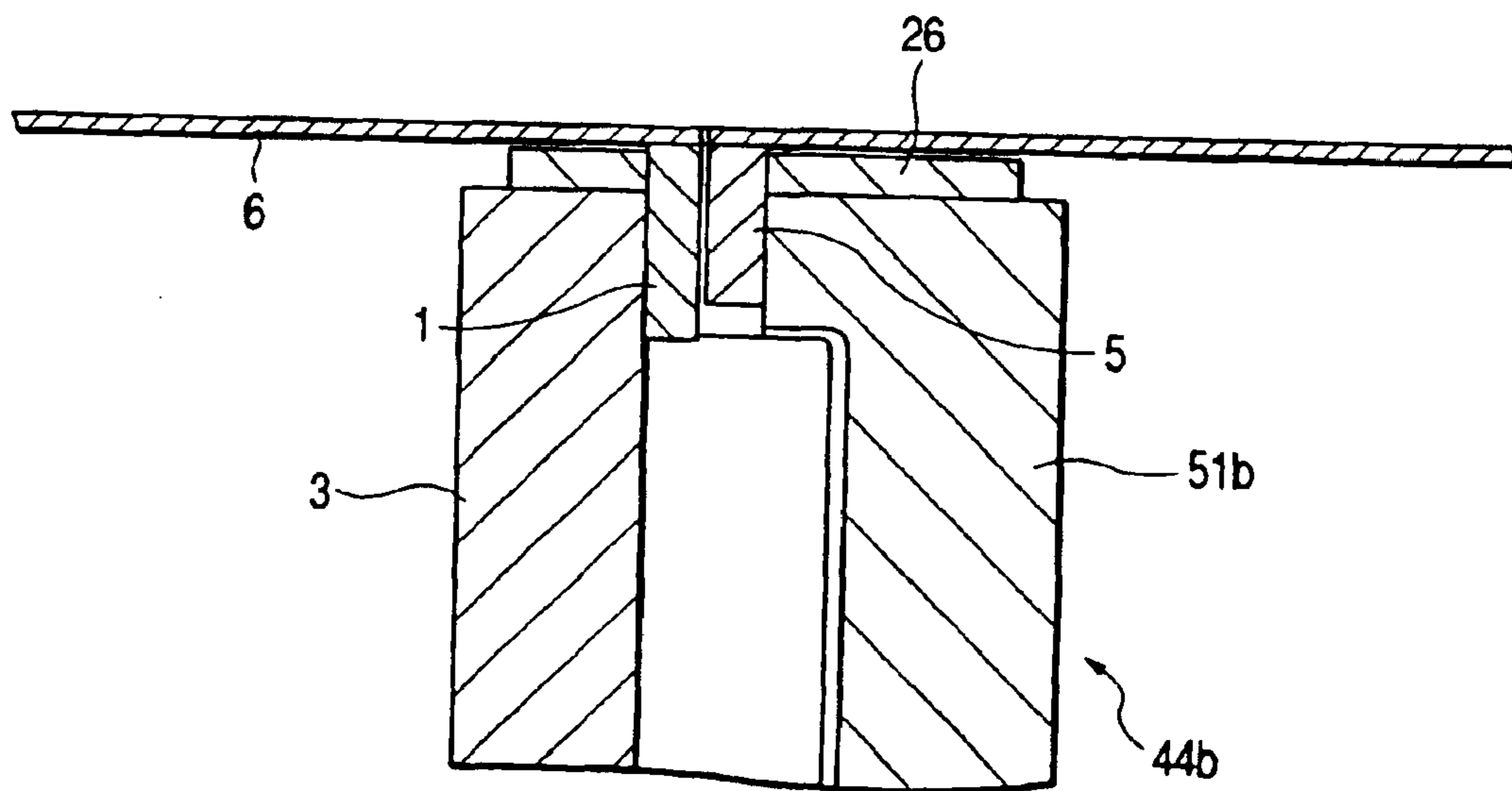
FIG. 41
