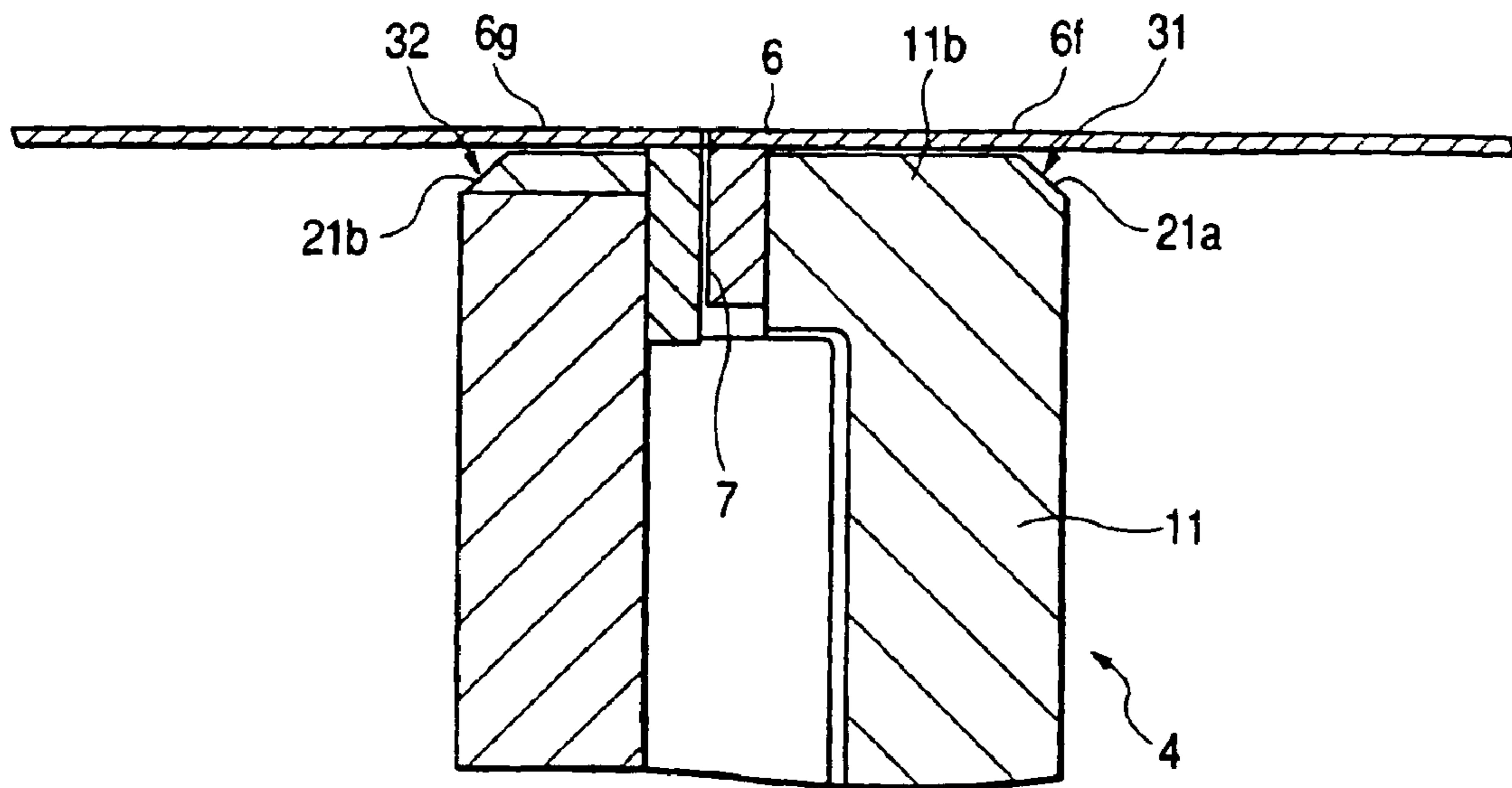
FIG. 36
