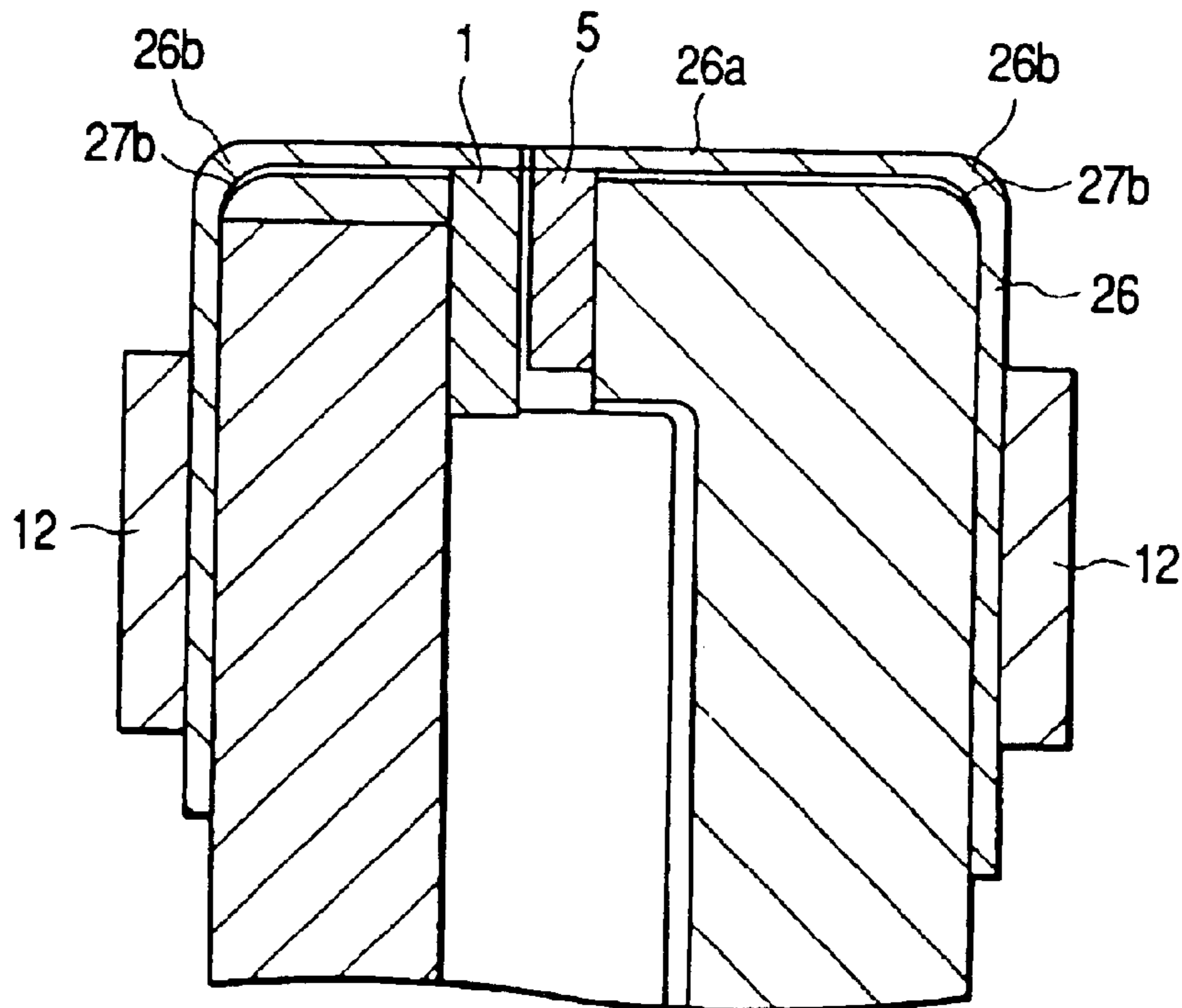
FIG. 21
