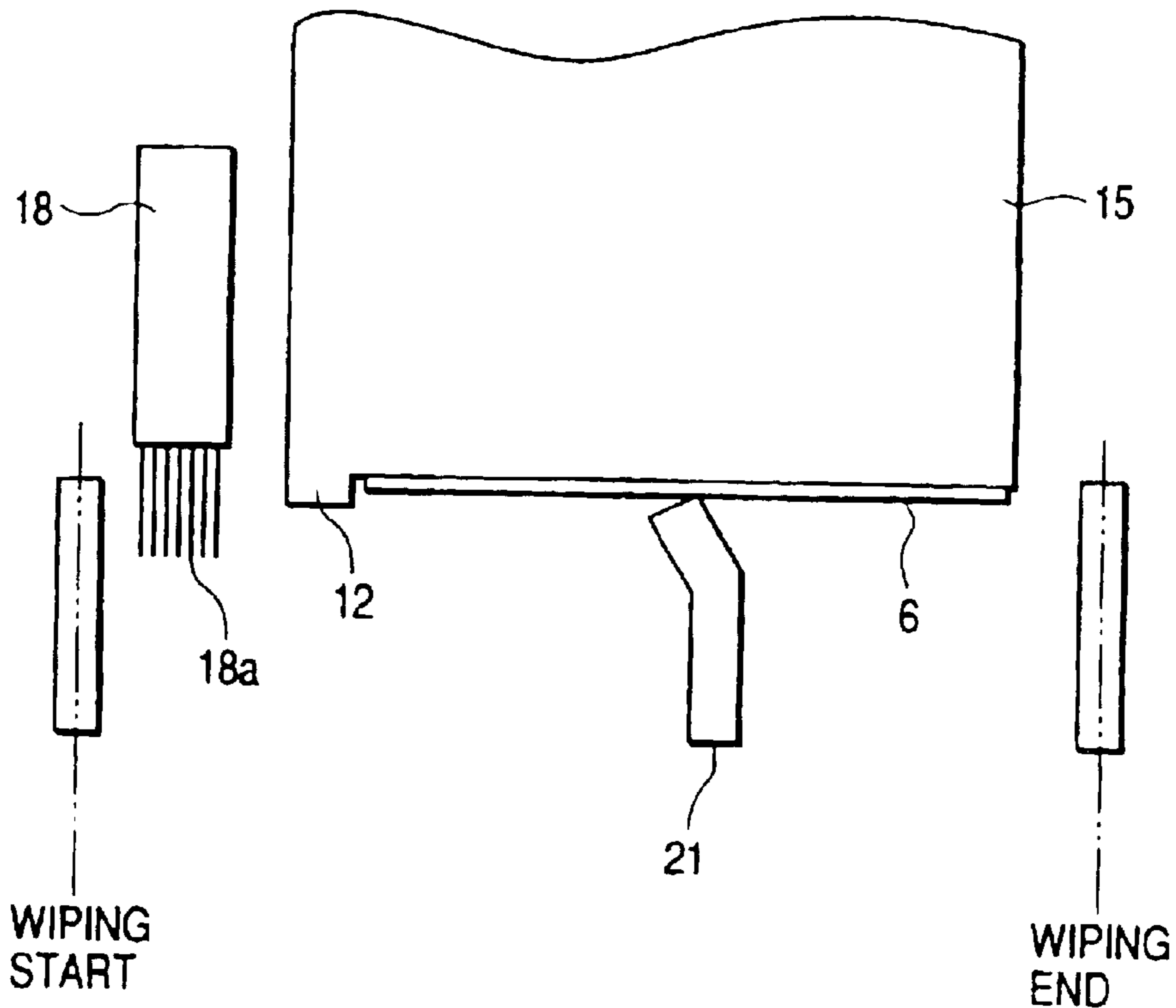
FIG. 65
