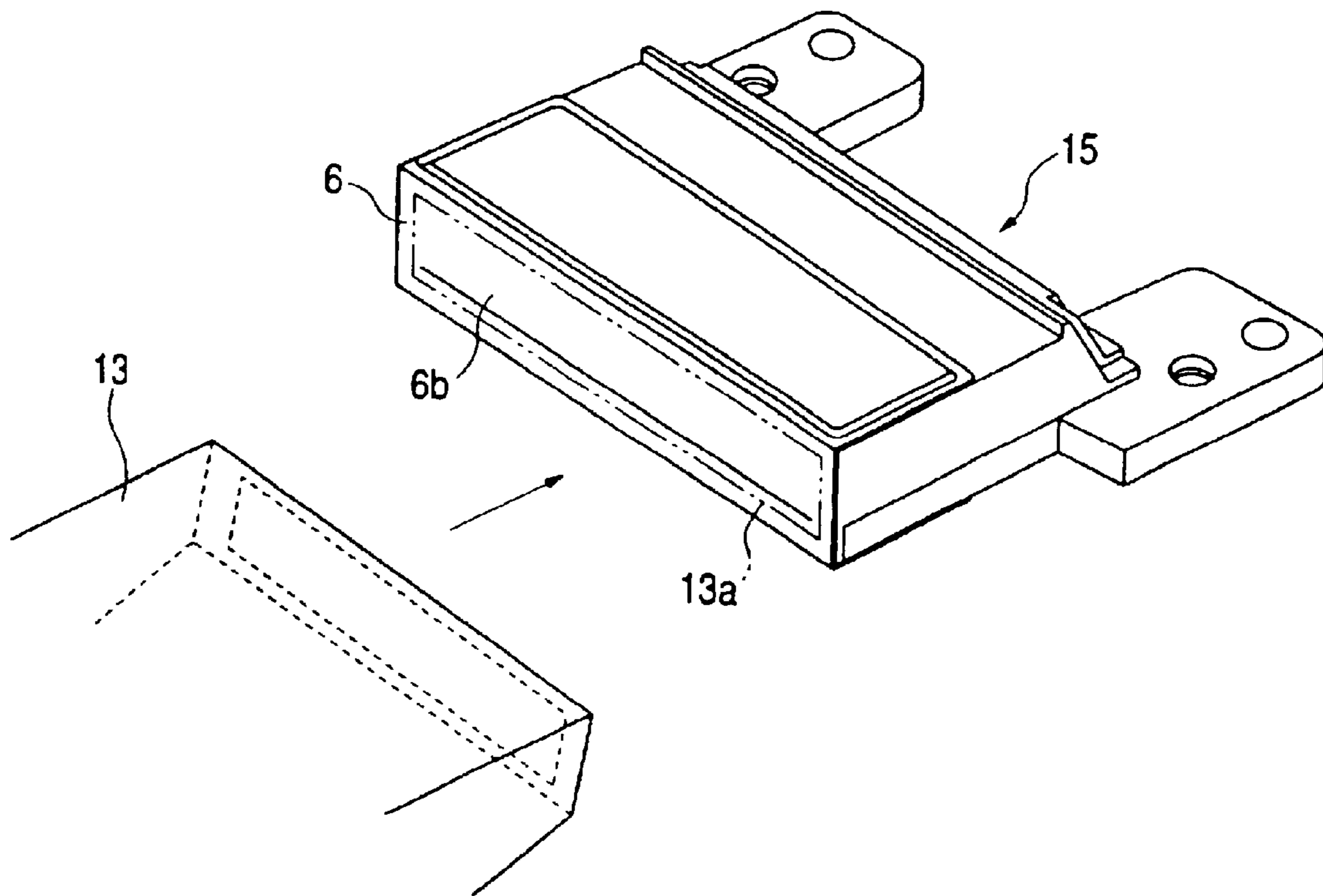
FIG. 34
