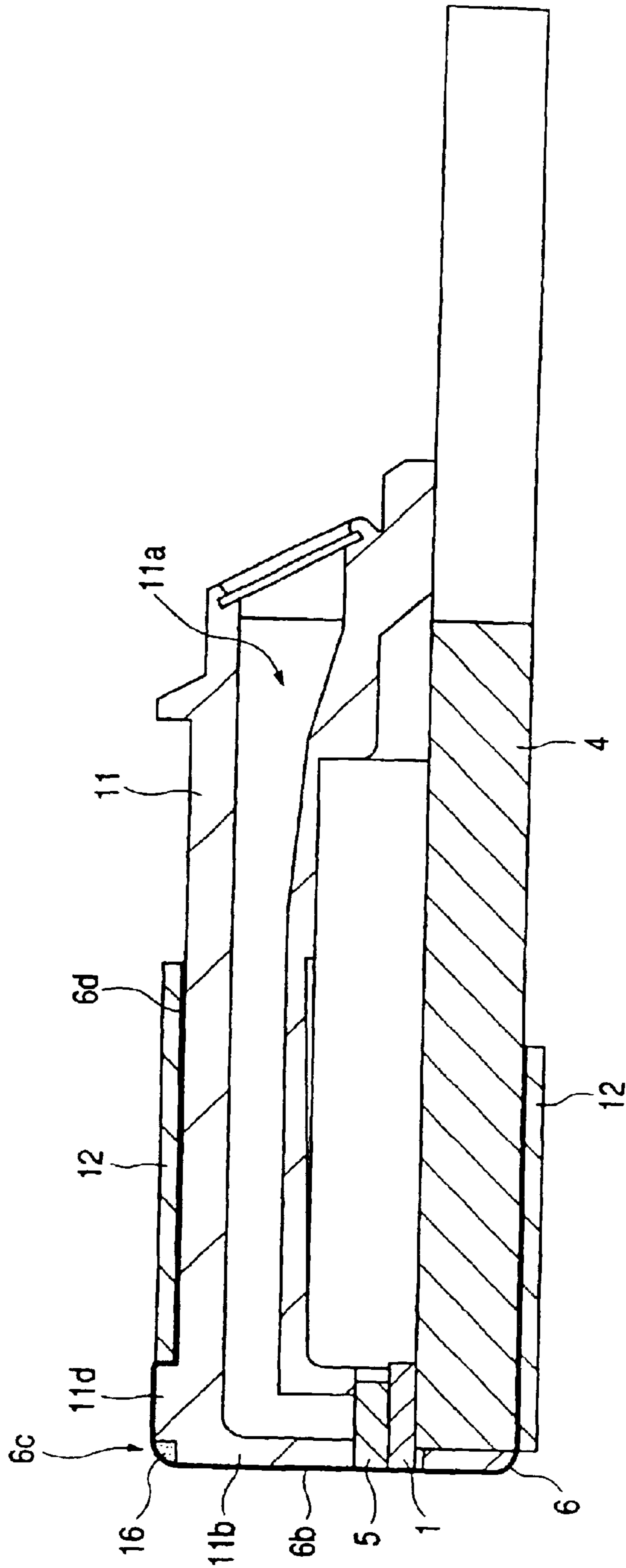
FIG. 17
