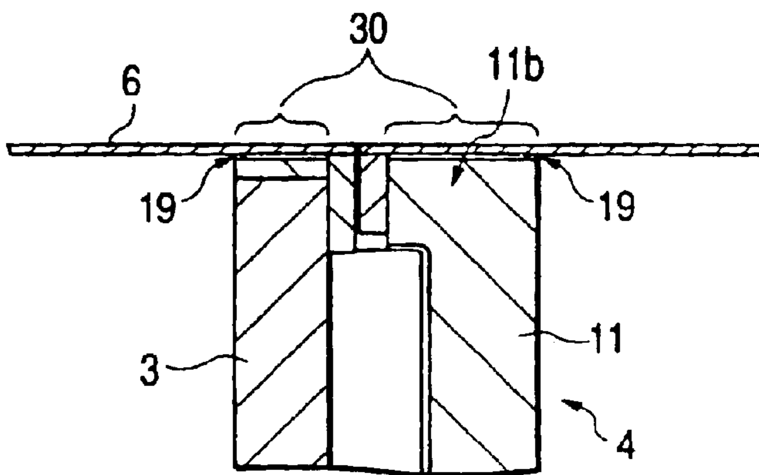
FIG. 54B
