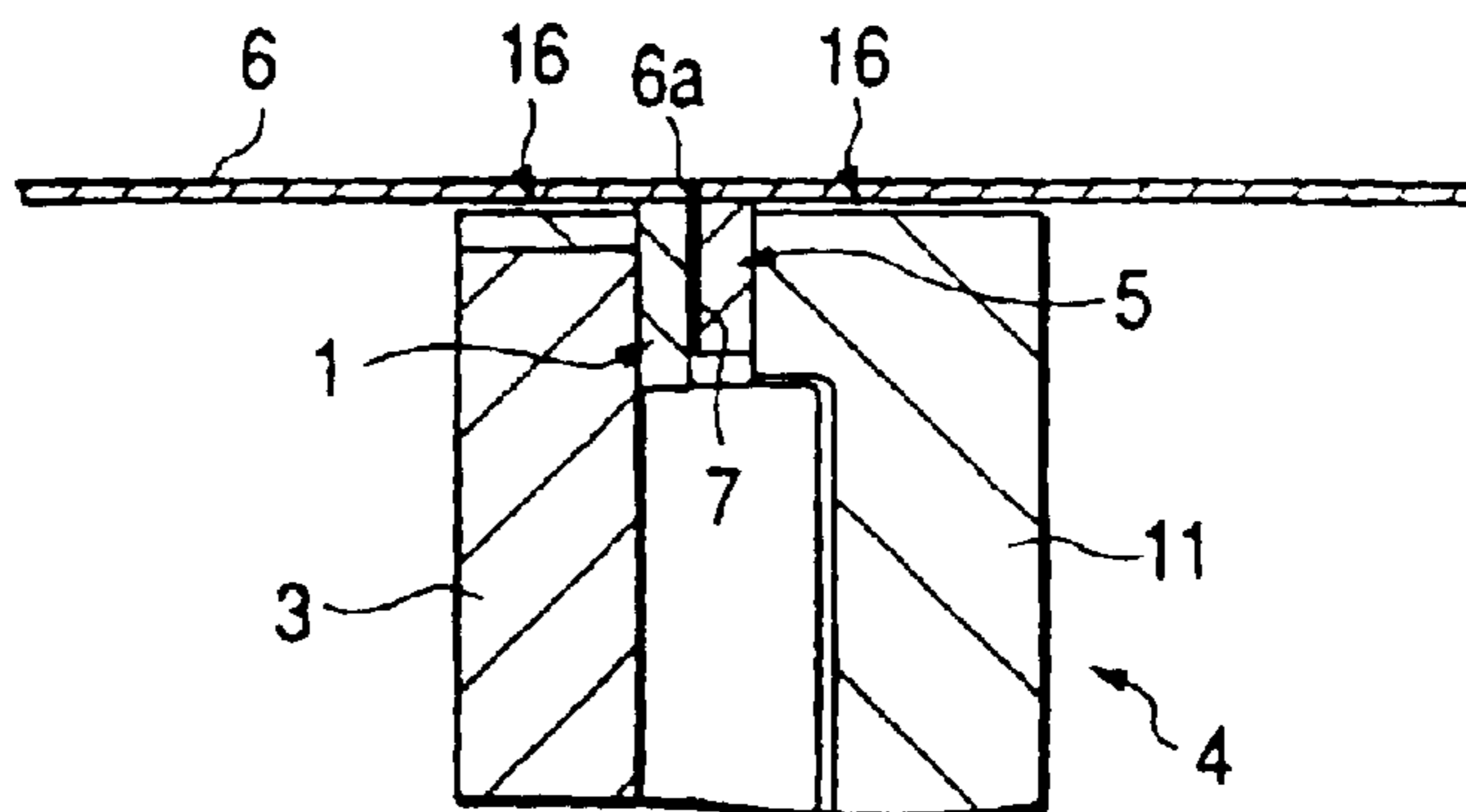
FIG. 54A
