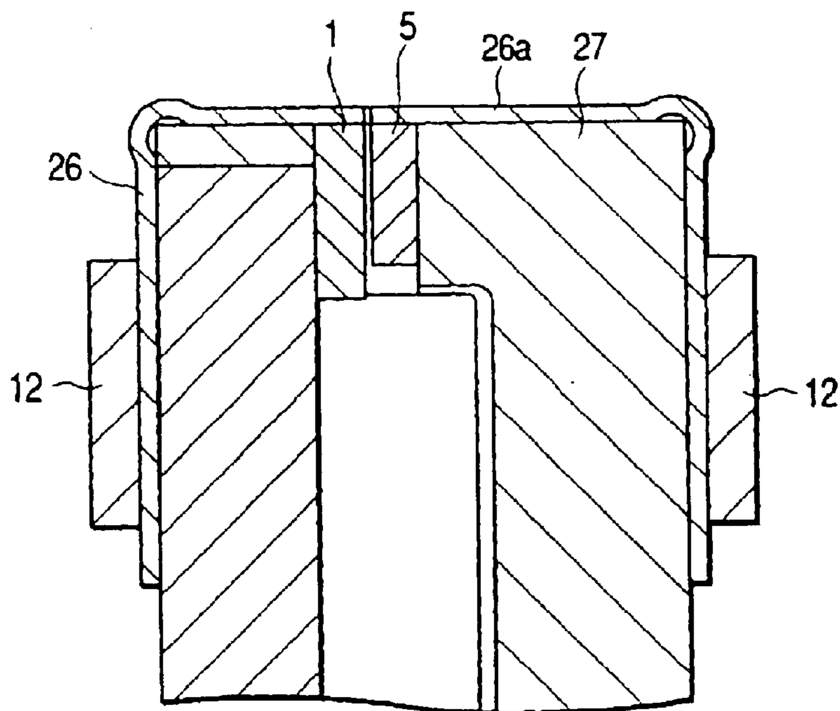
FIG. 19
