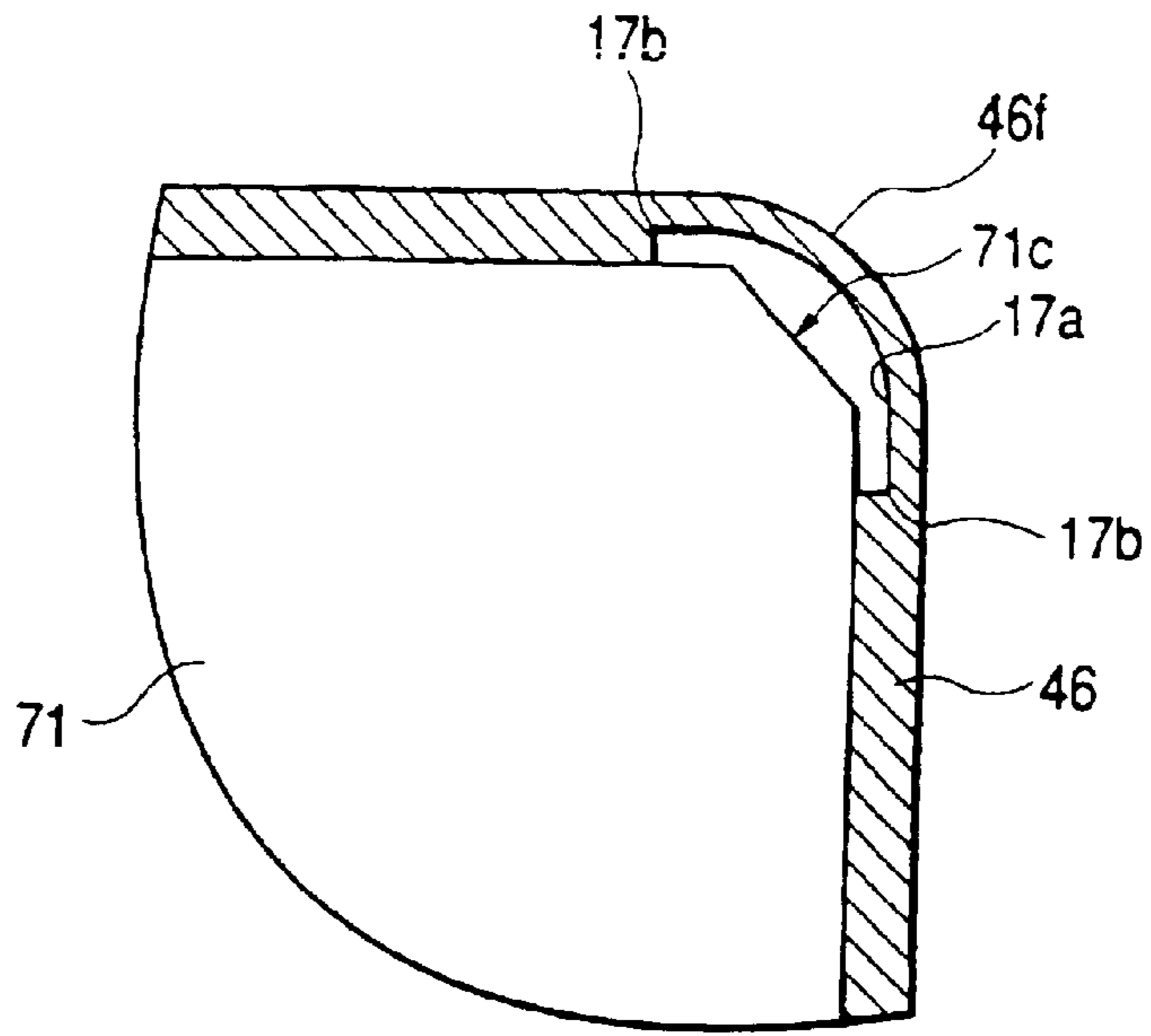
FIG. 46
