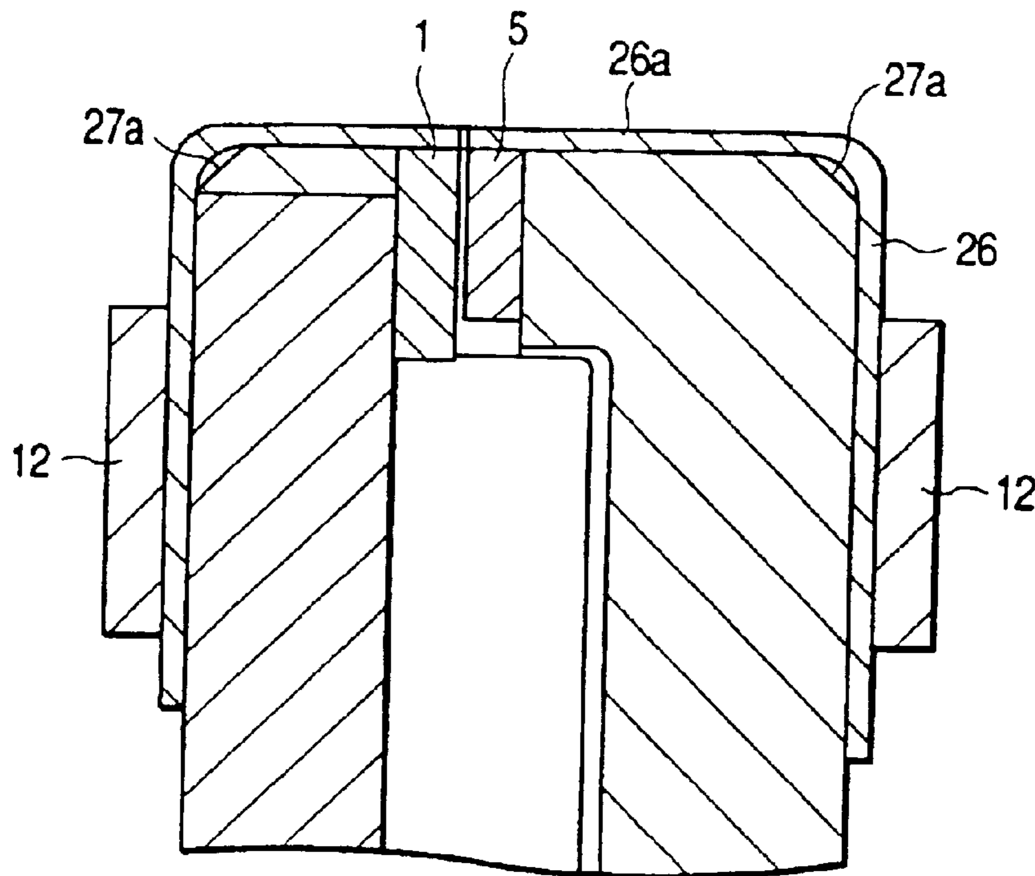
FIG. 20
