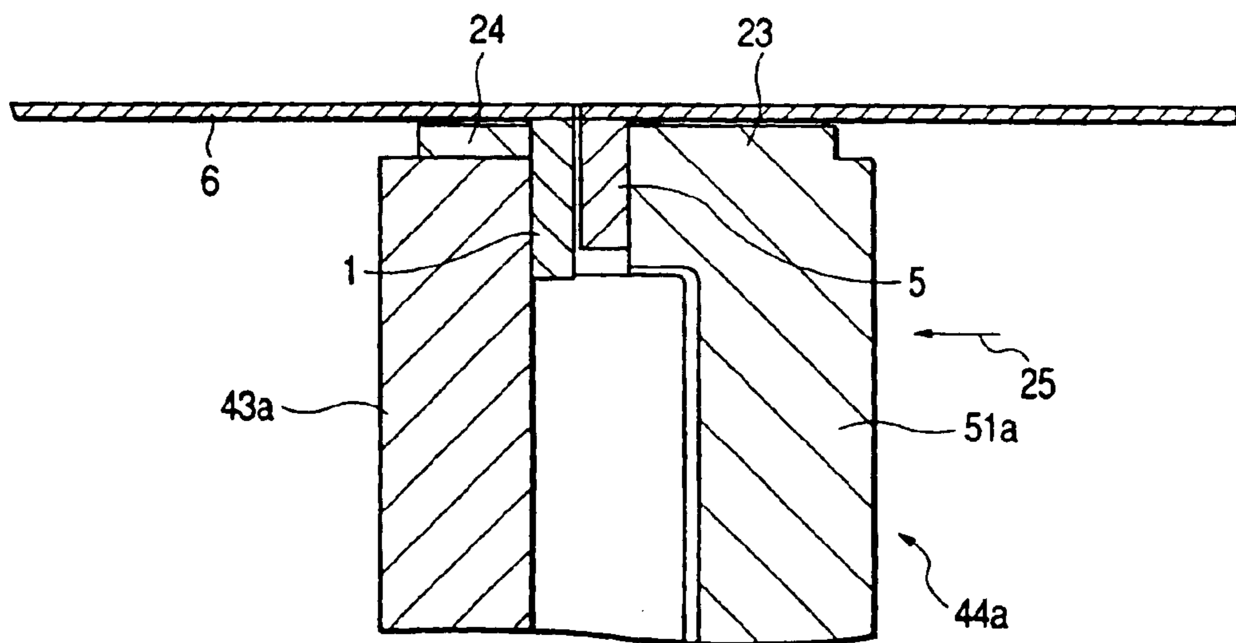
FIG. 39
