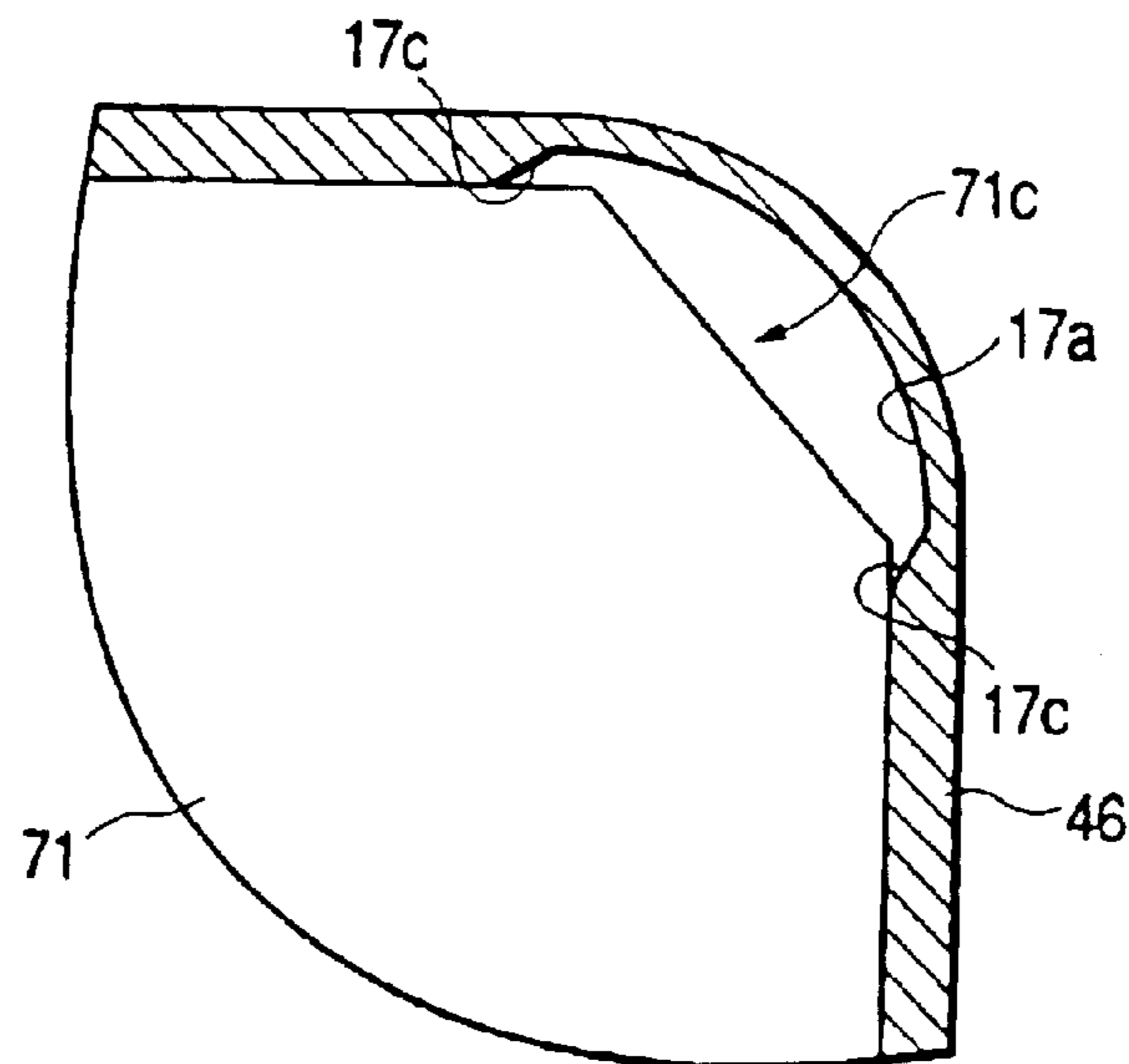
FIG. 49
