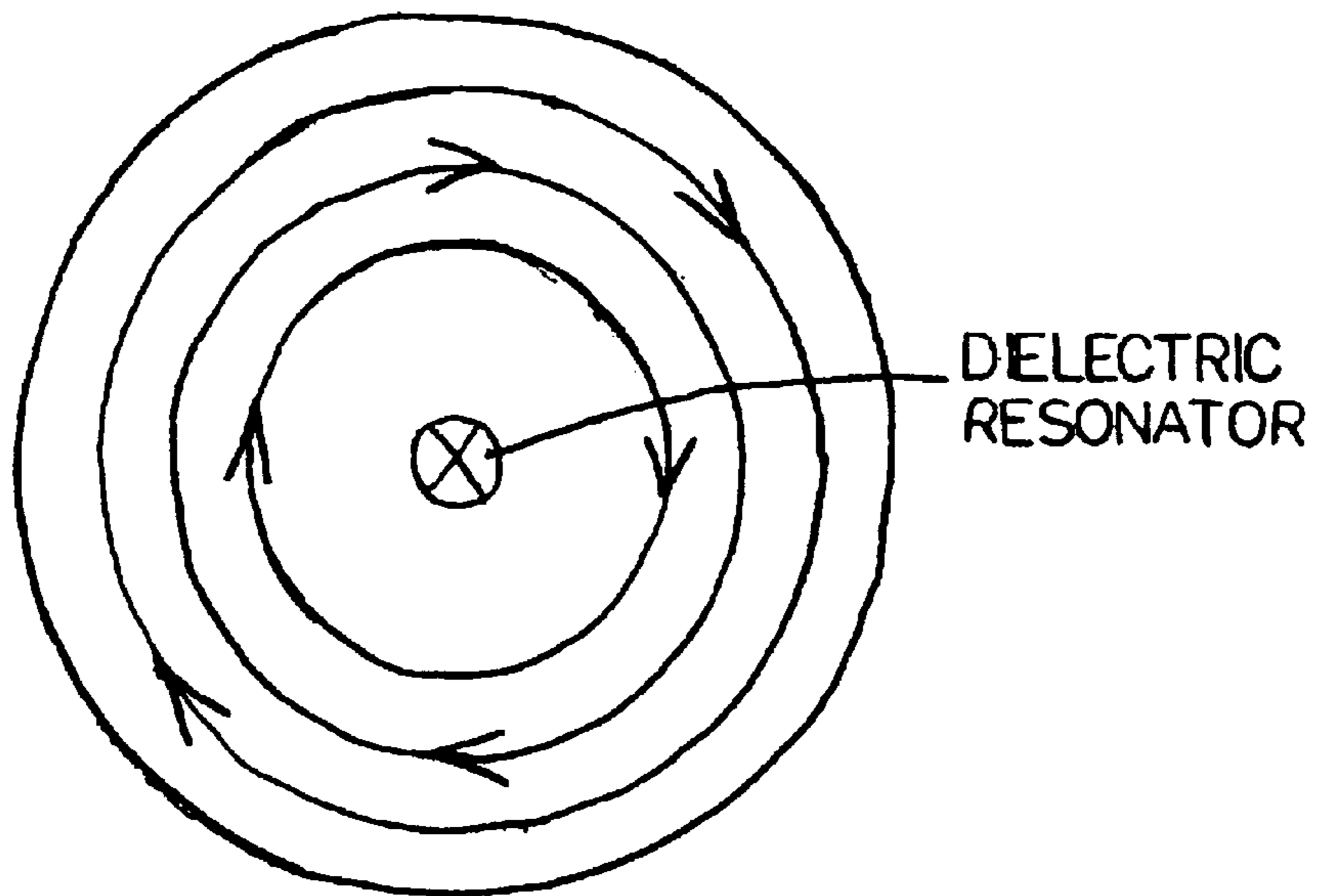
DIELECTRIC RESONATOR : D > L FIG. 1
