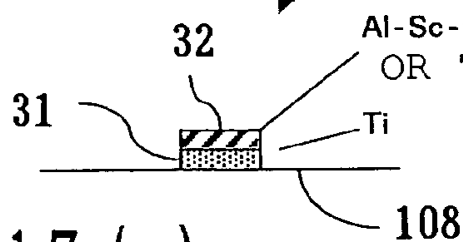
Fig. 17 (b)
