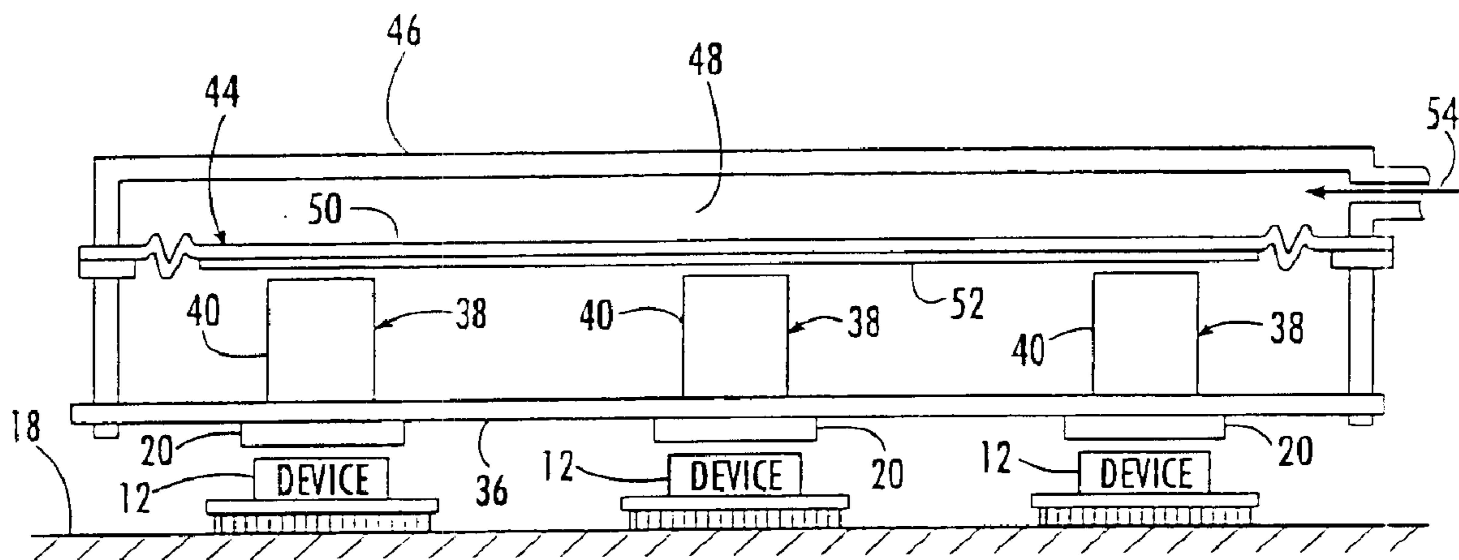
FIG. 2A.
