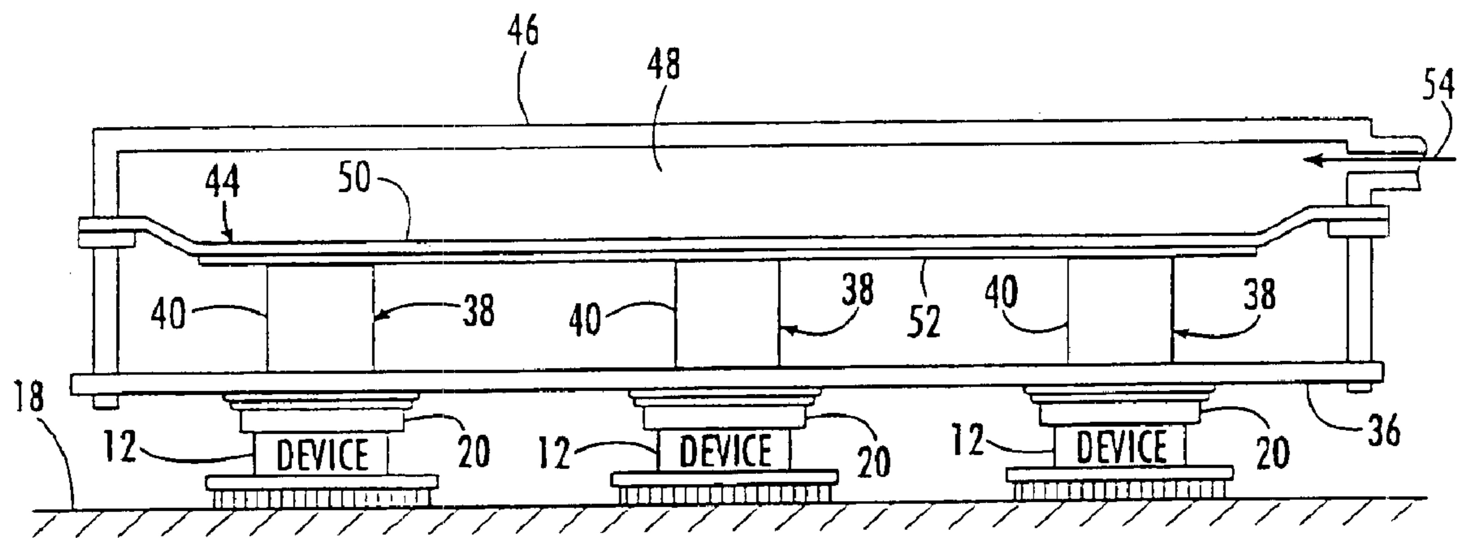
FIG. 2B.
