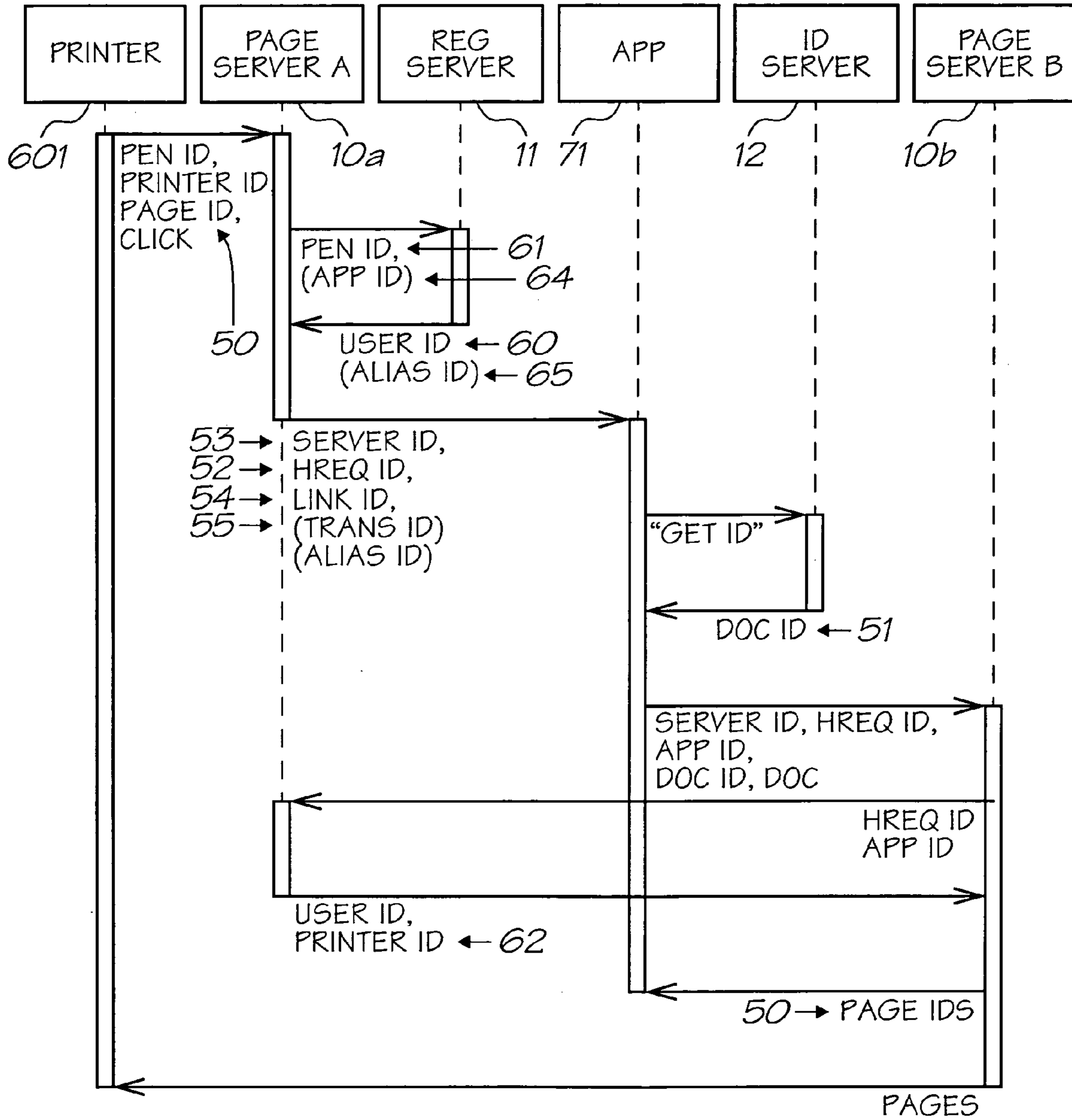
FIG. 42
