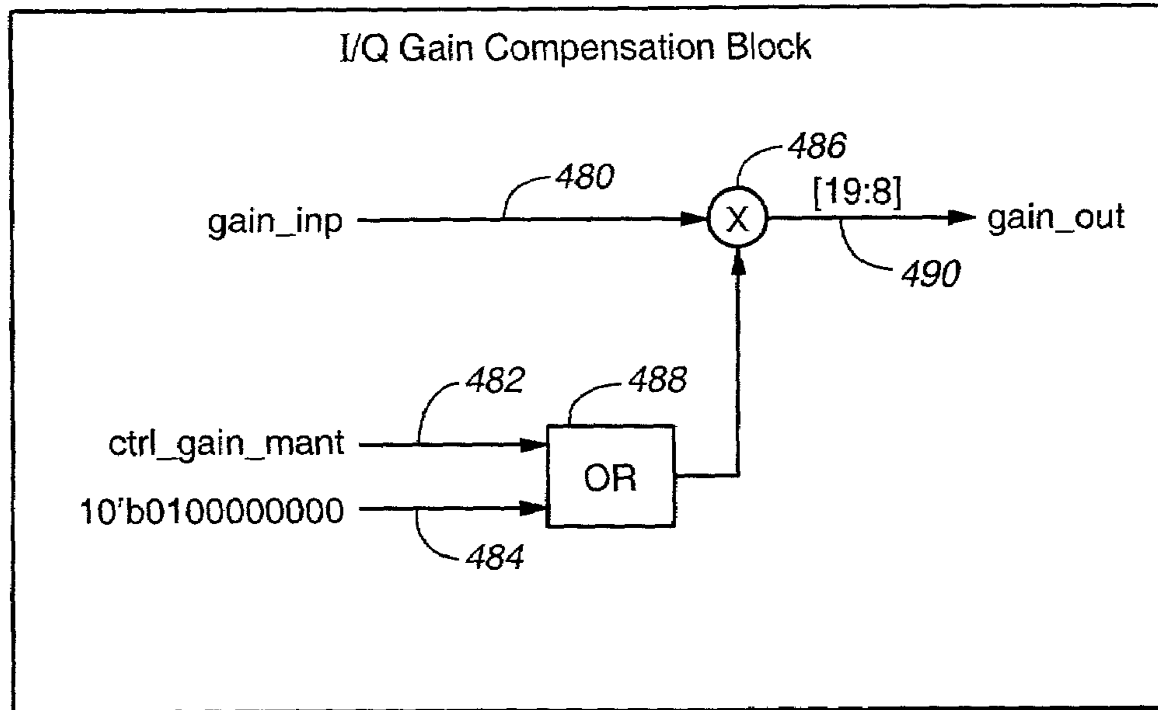
FIG. 17
