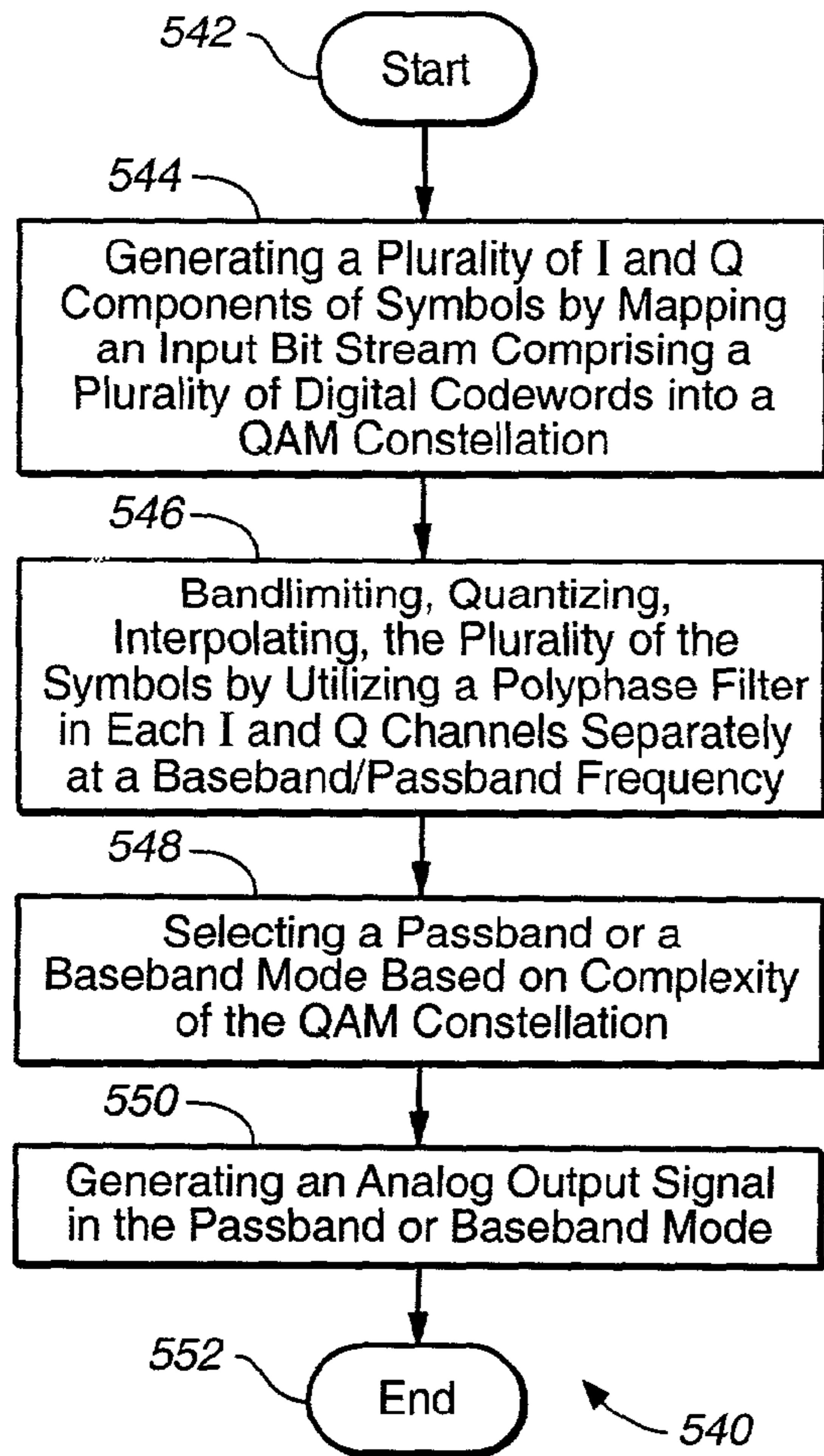
FIG. 23
