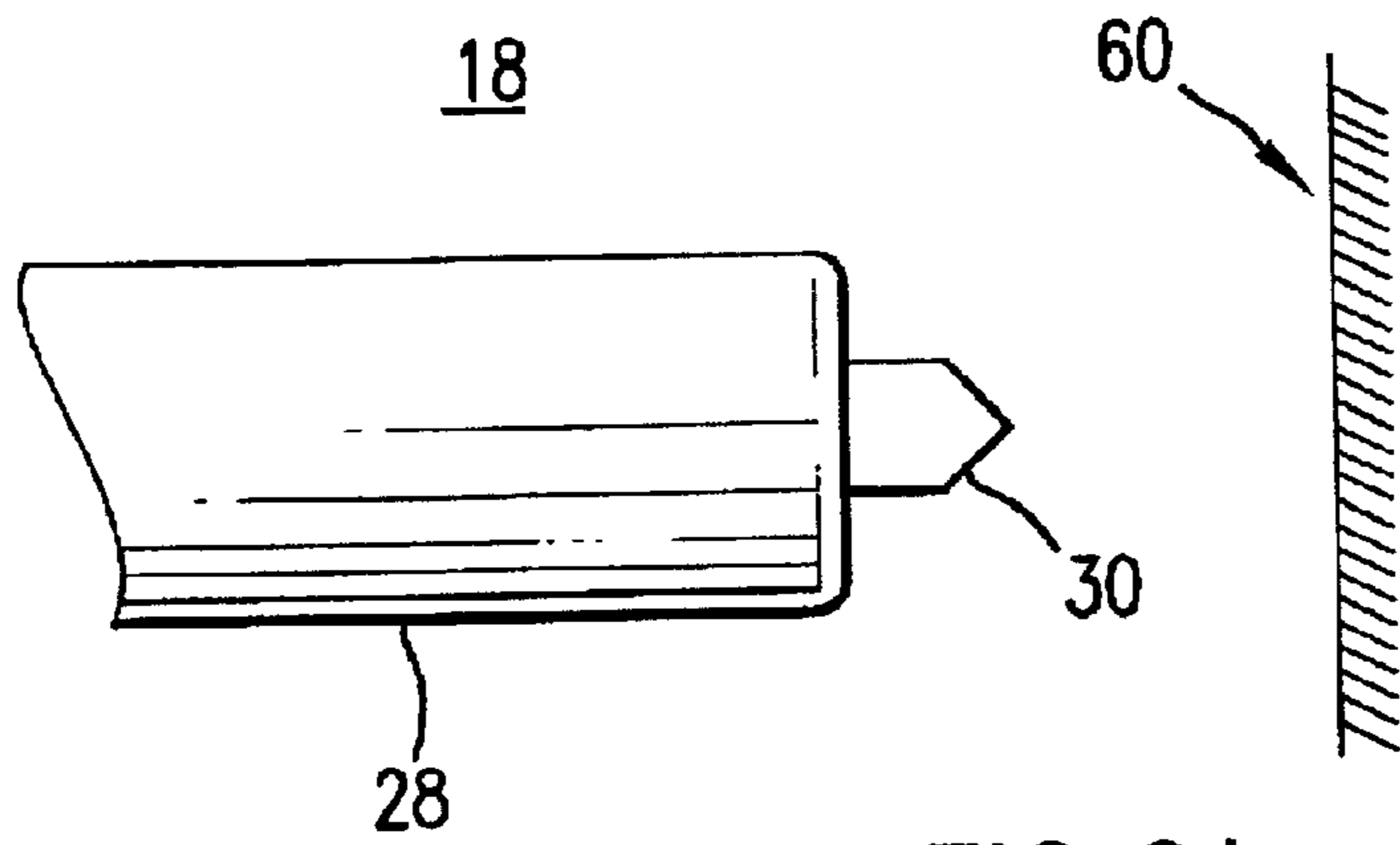
FIG. 6A
