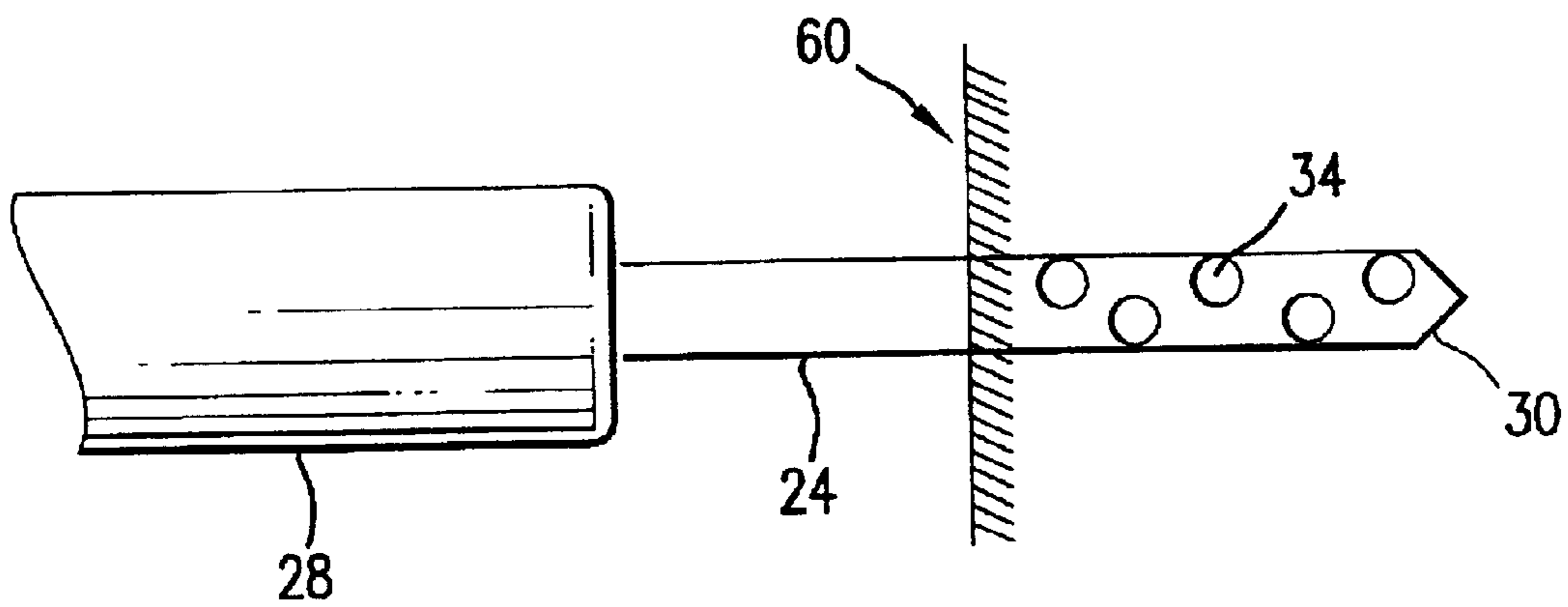
FIG. 6B
