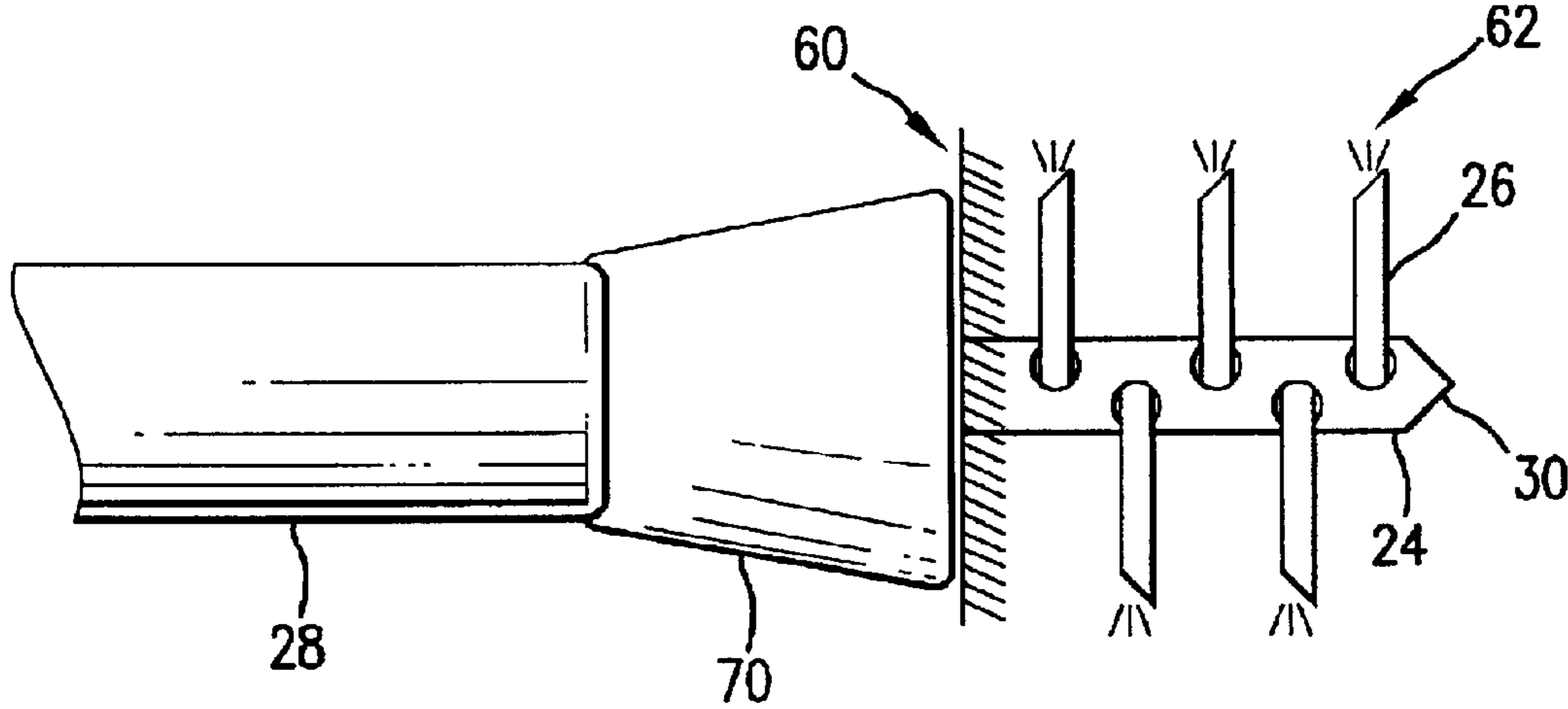
FIG. 7C
