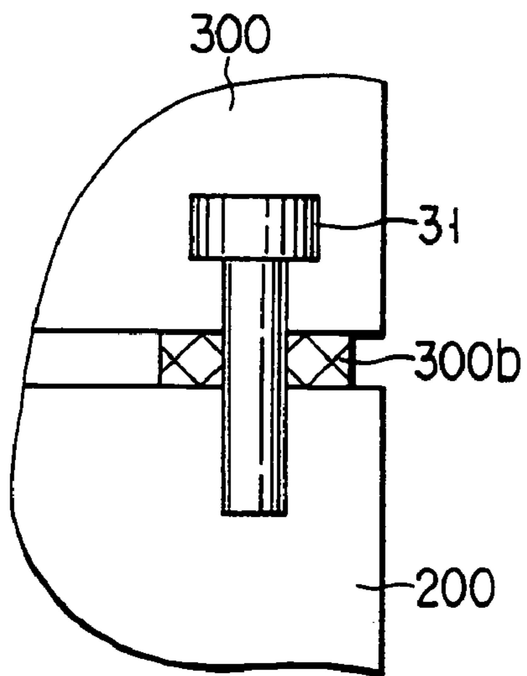
FIG. 27A
