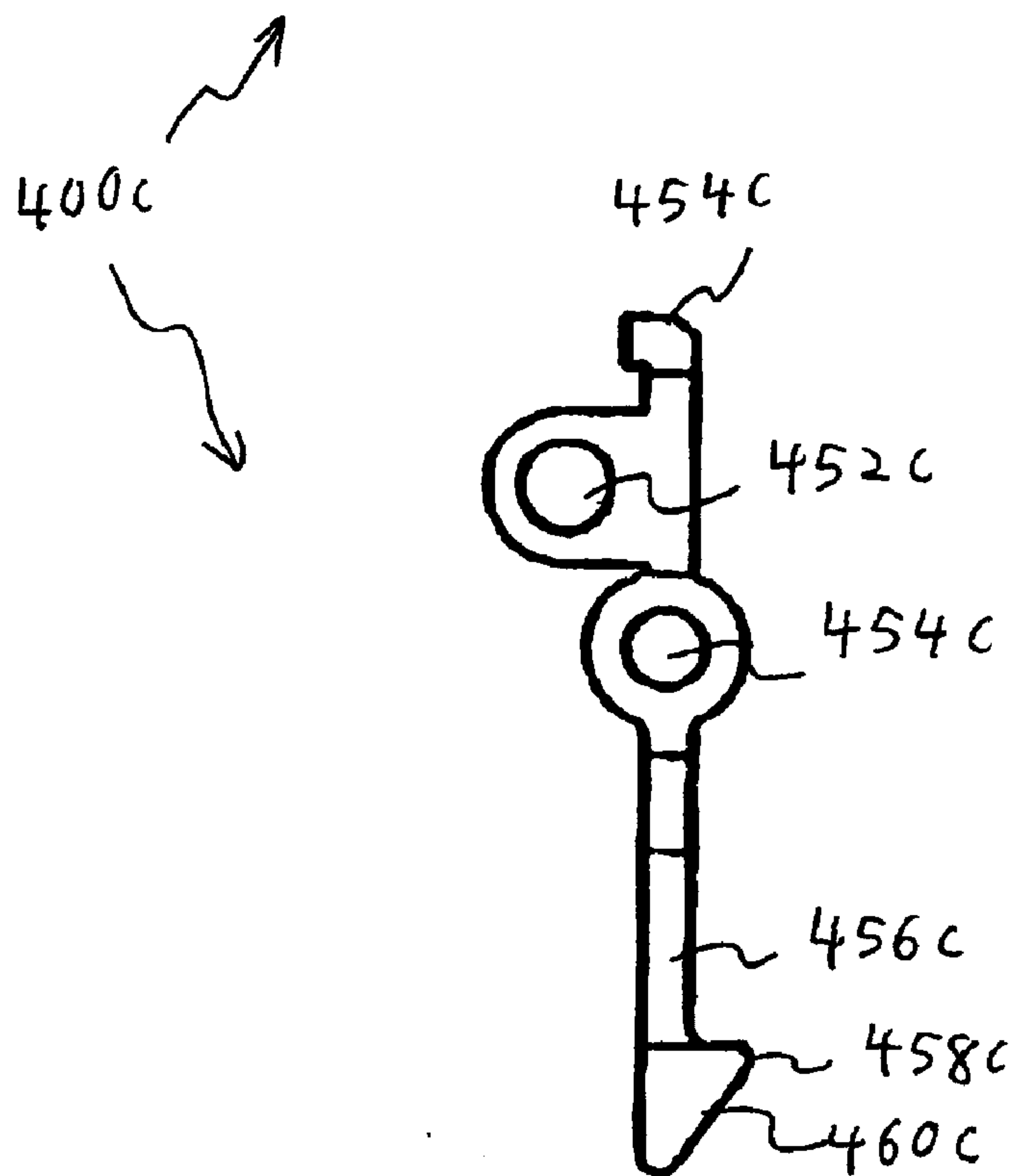
FIG. 52
