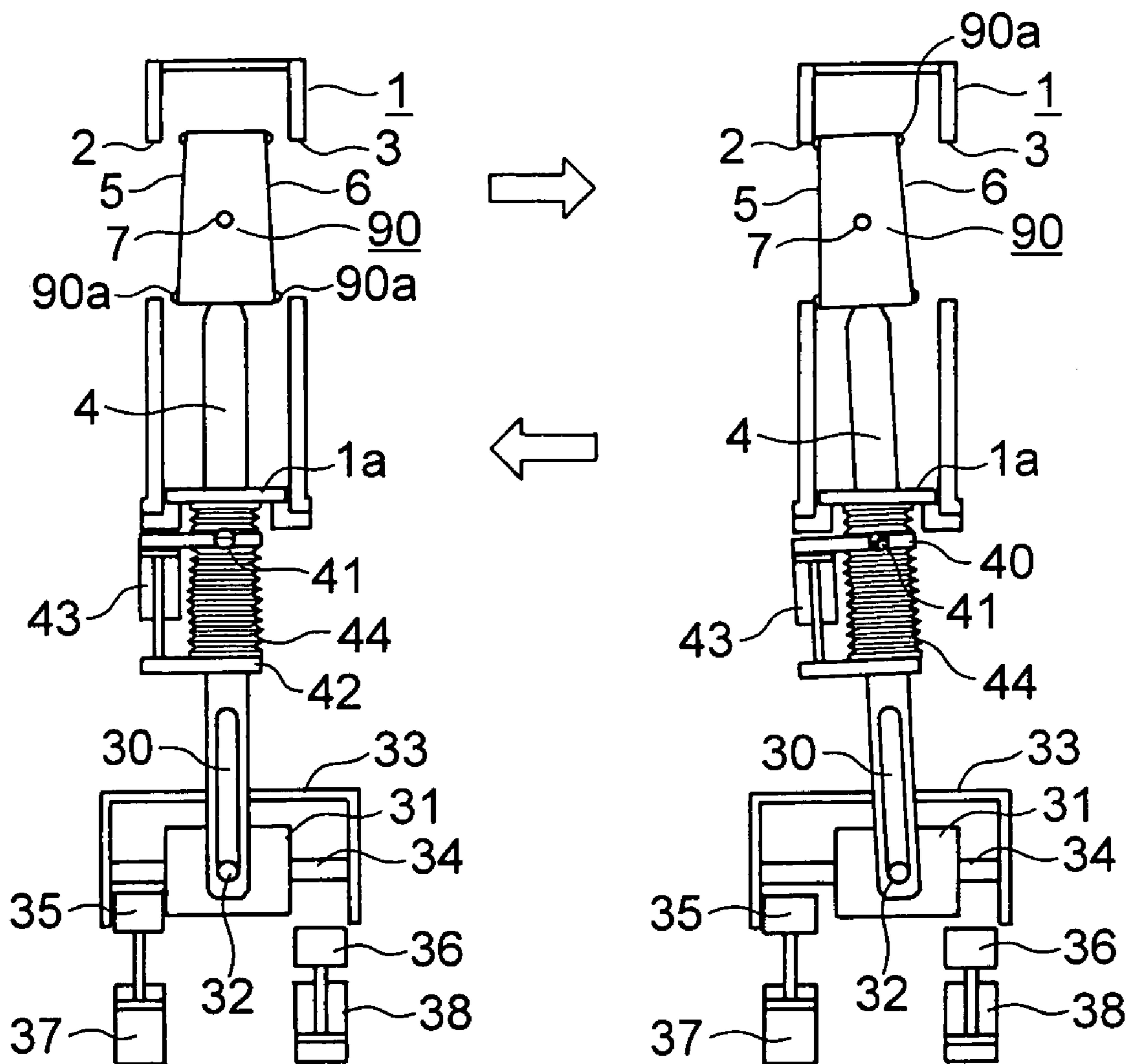
FIG. 2C
