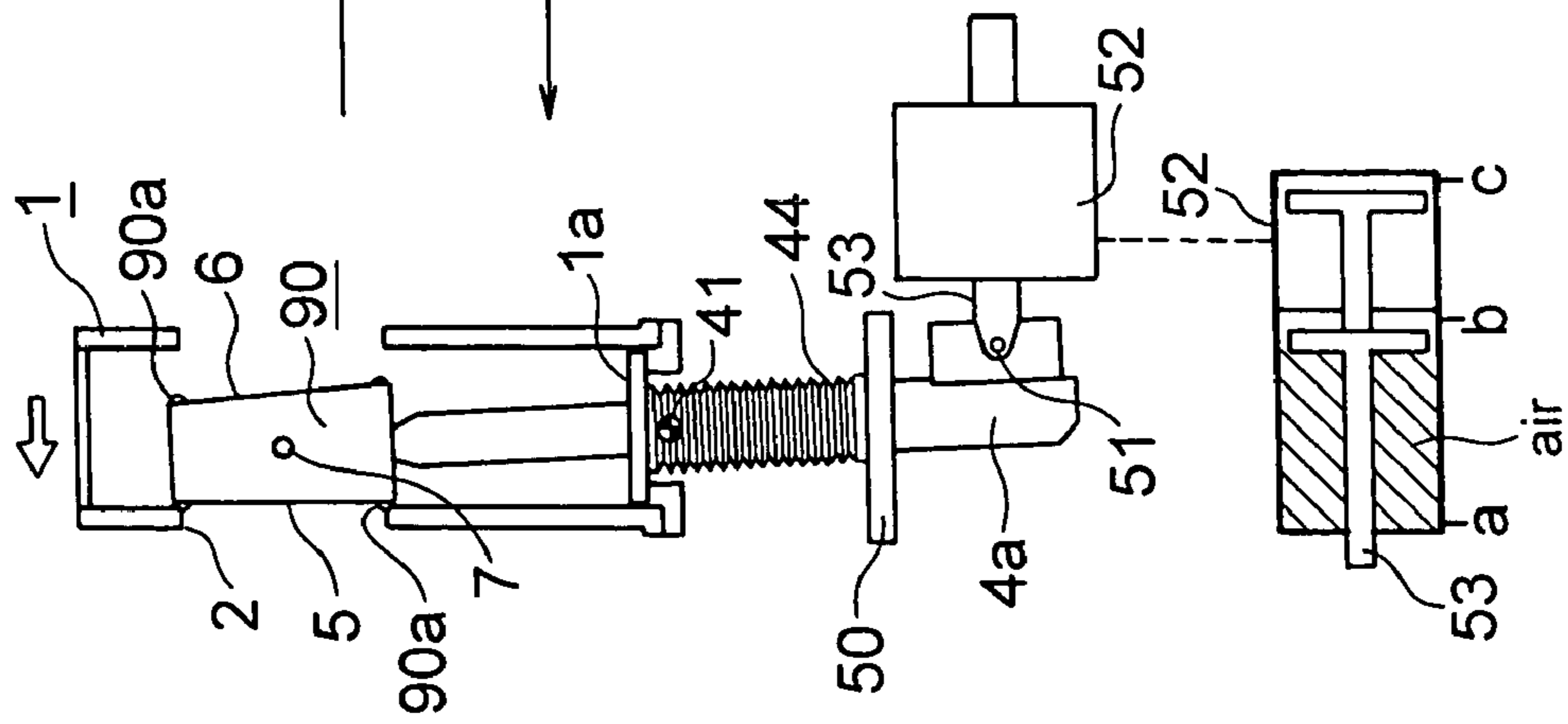
FIG. 4A
