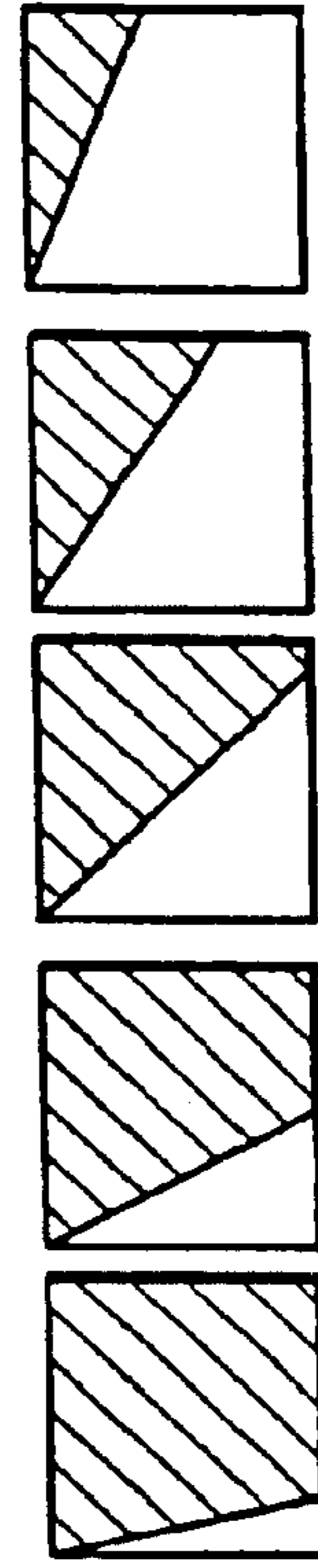
M=4
