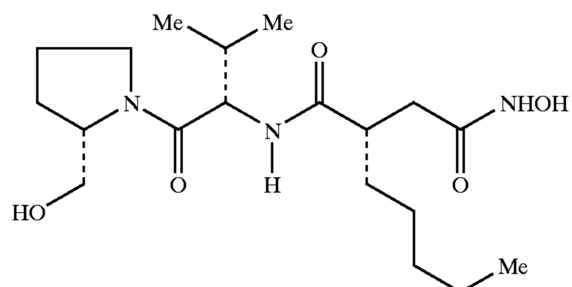
Epiactinonin
