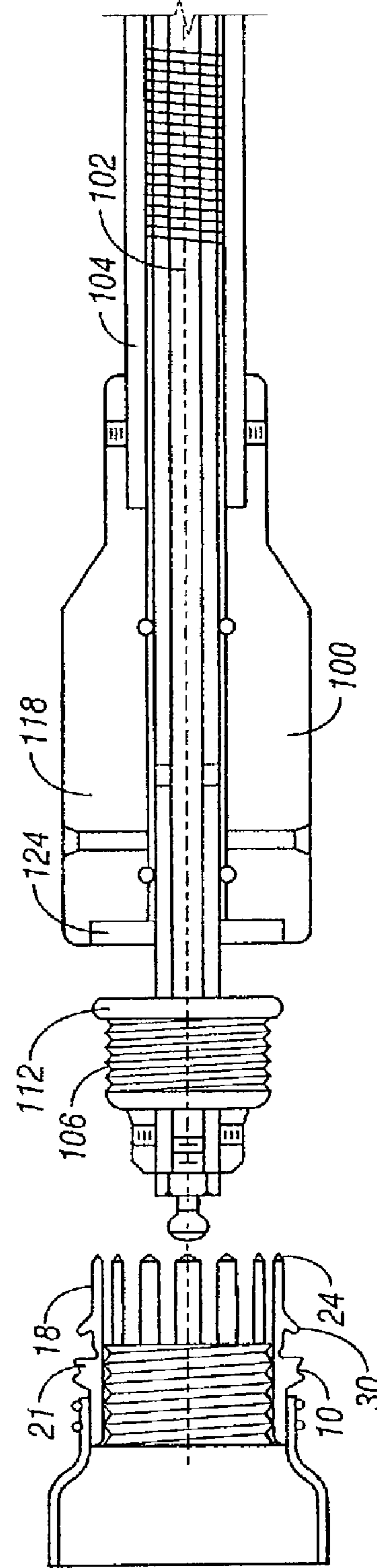
FIG. 9
