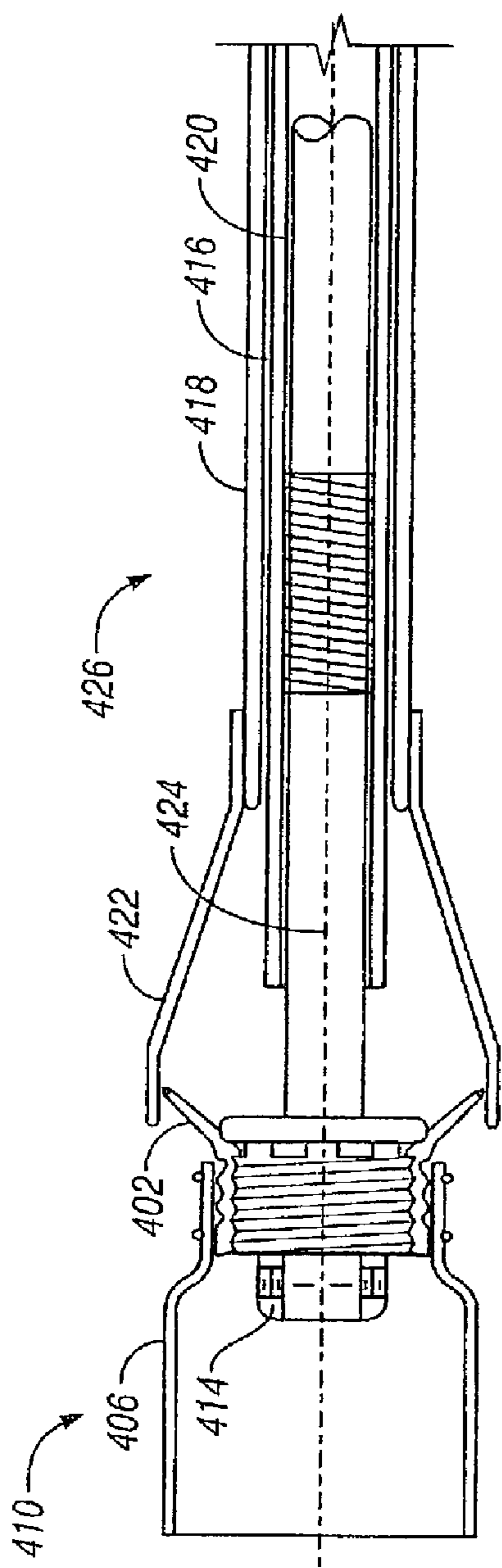
FIG. 18
