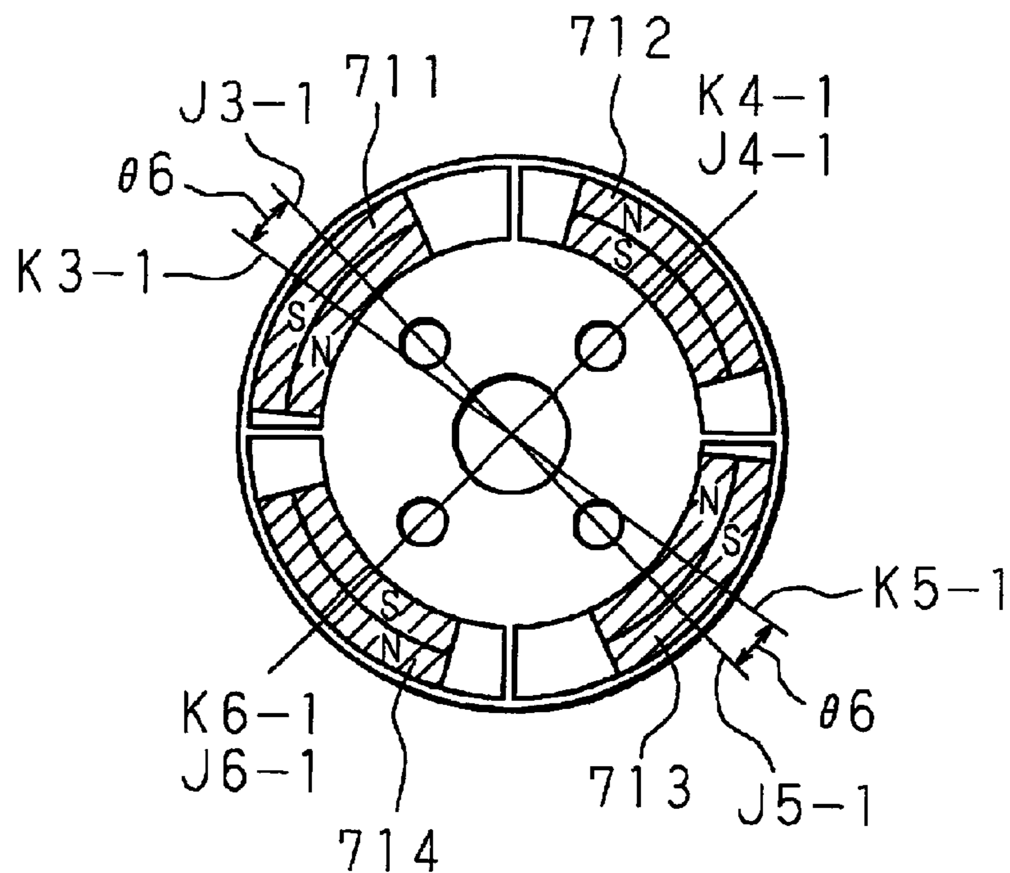
FIG. 20A
