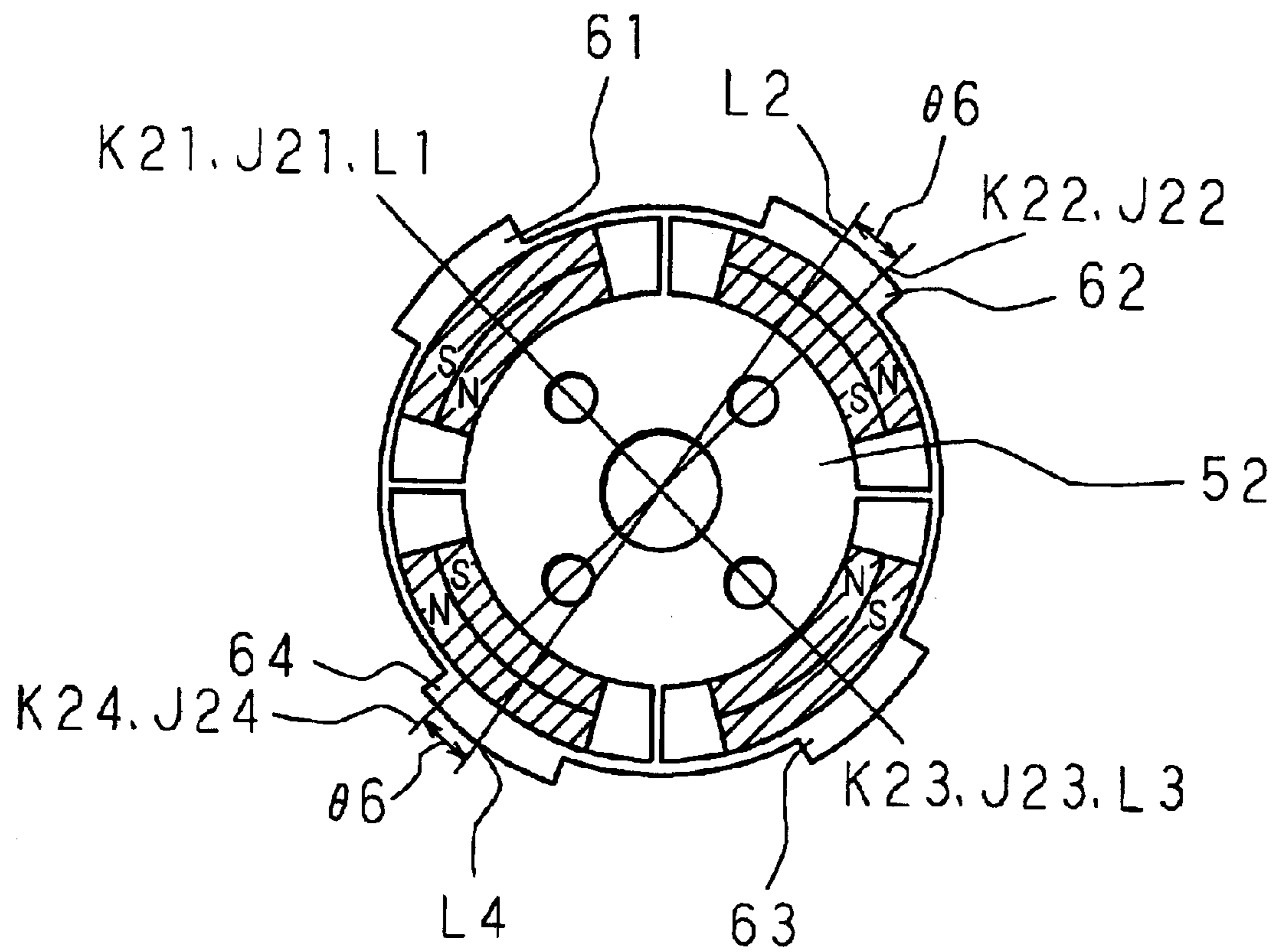
FIG. 24
