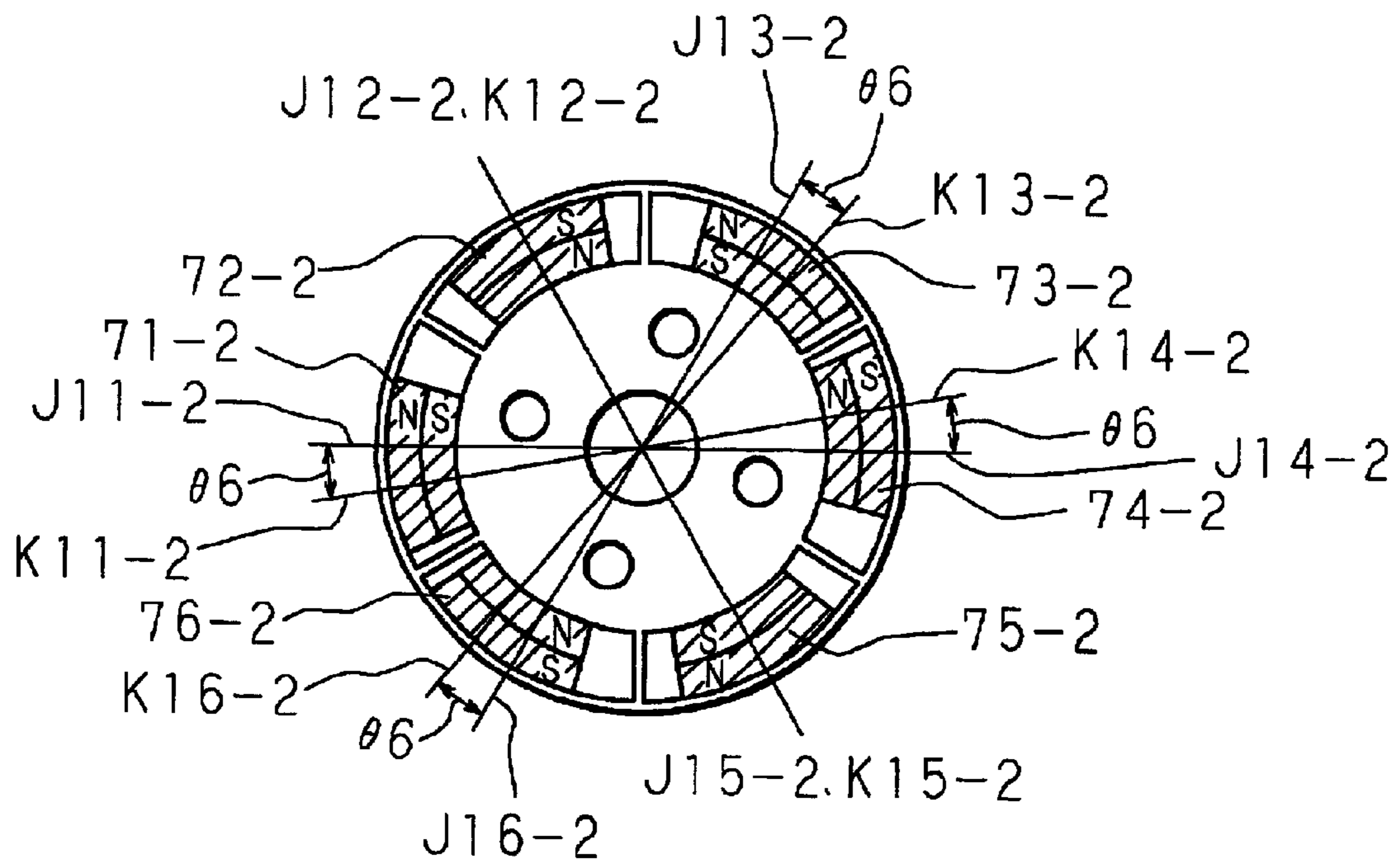
FIG. 23B
