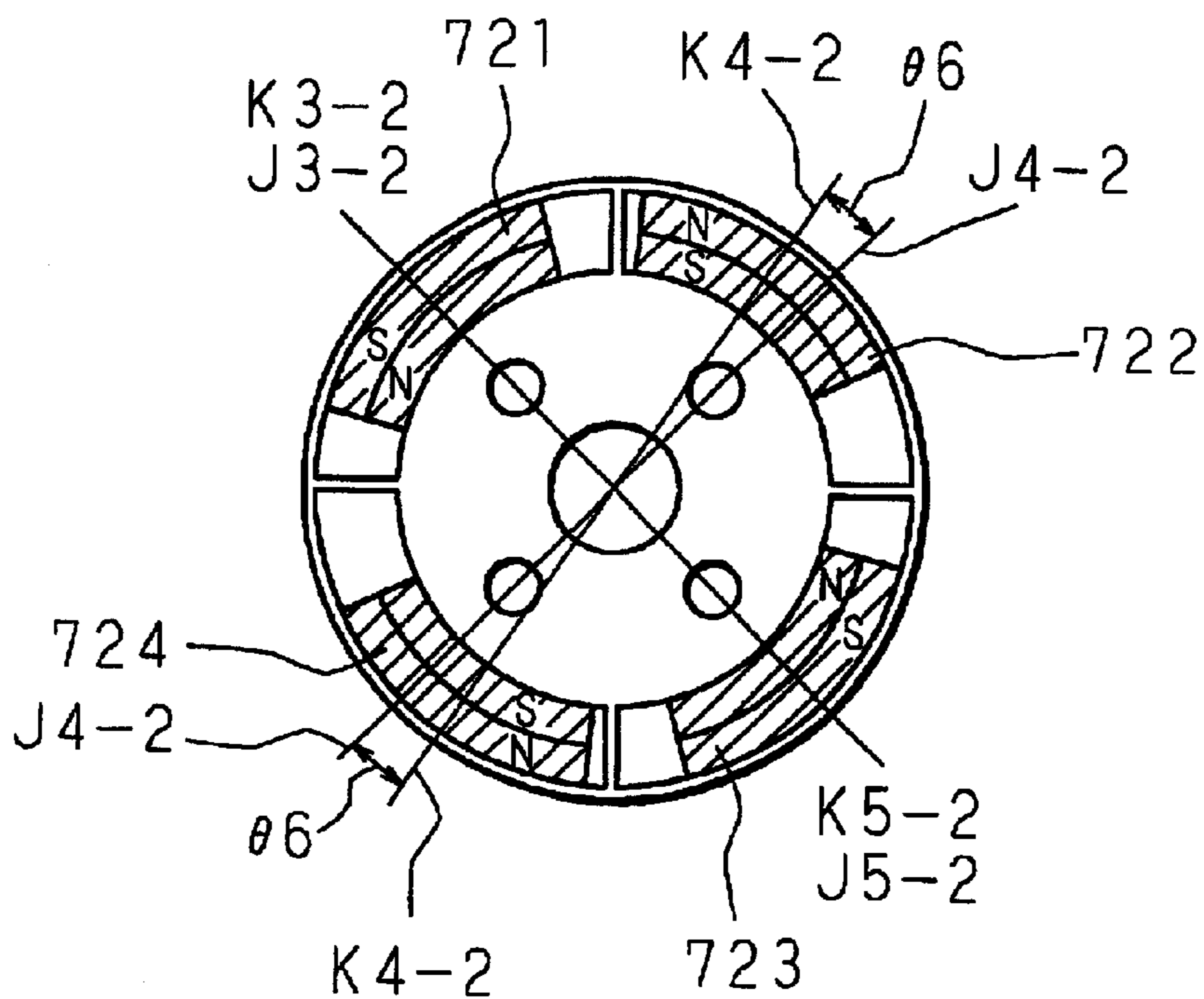
FIG. 20B
