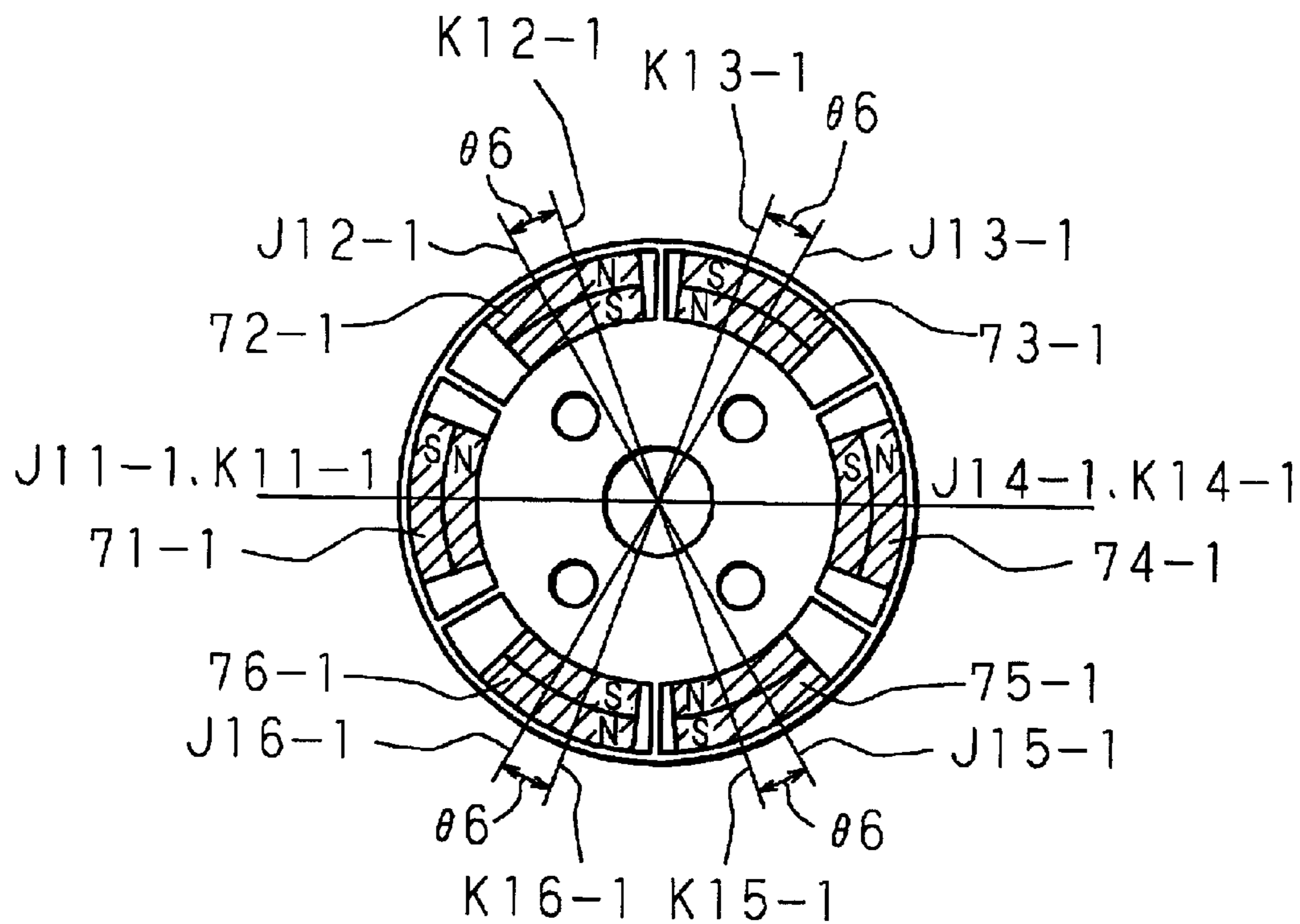
FIG. 23A
