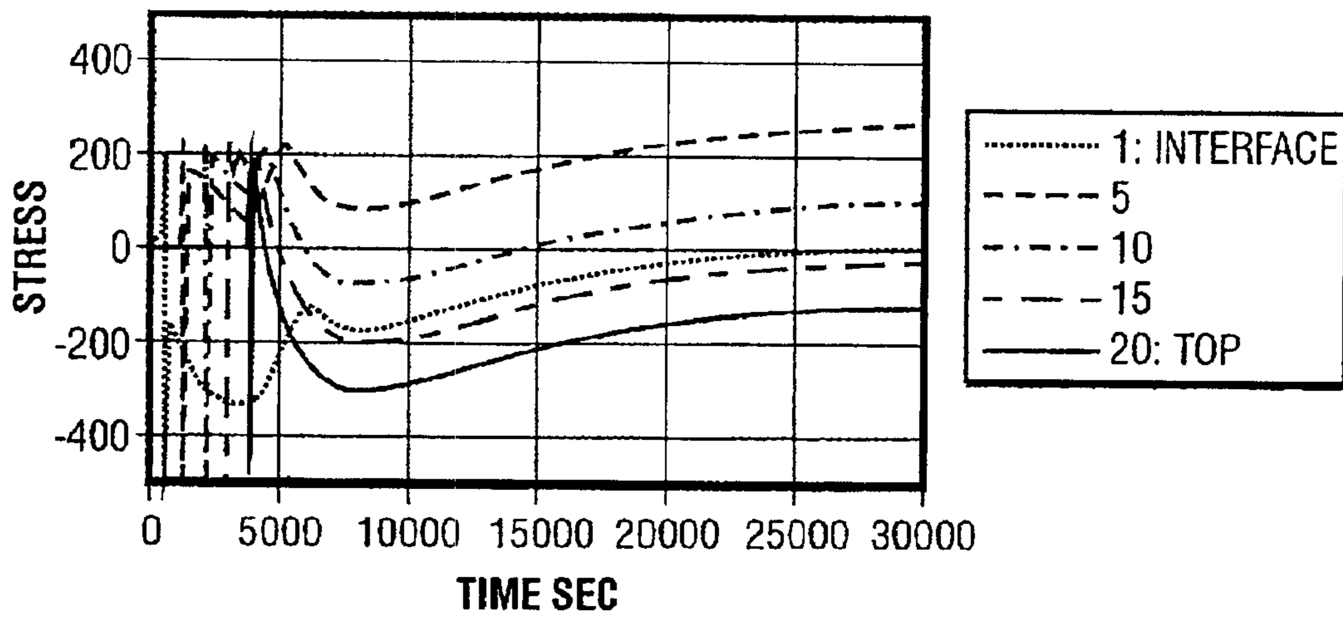
In-Plane Stress FIG. 16
