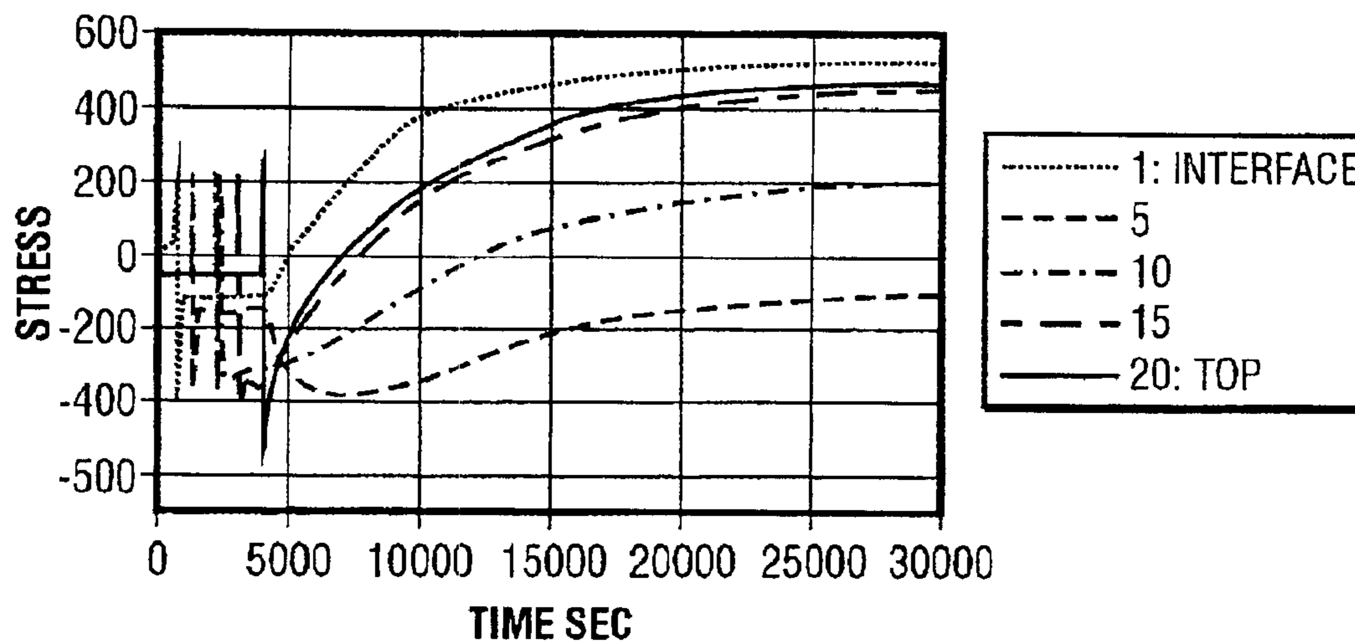
In-Plane Stress FIG. 11
