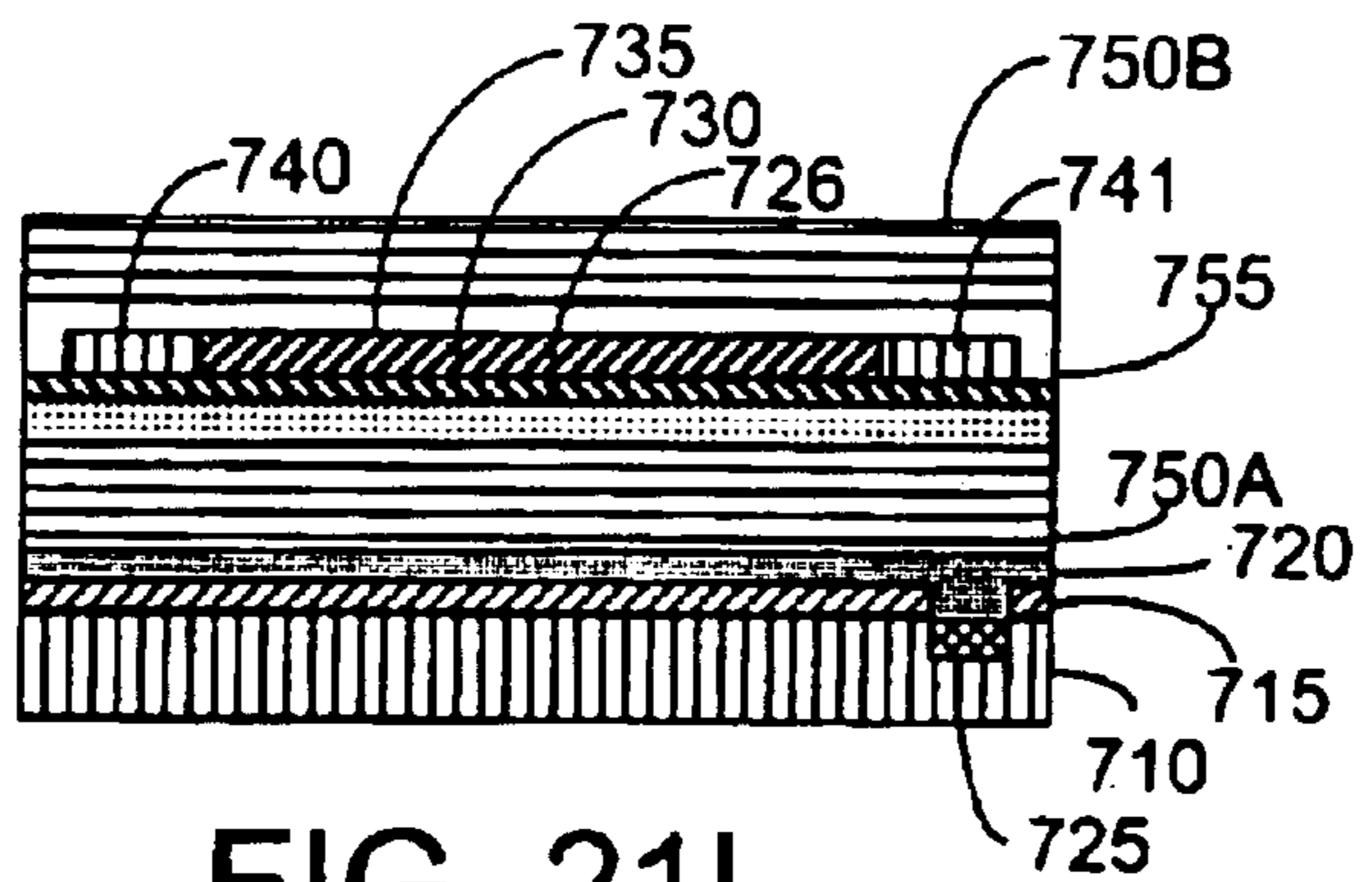
FIG. 21K SECTION B-B
