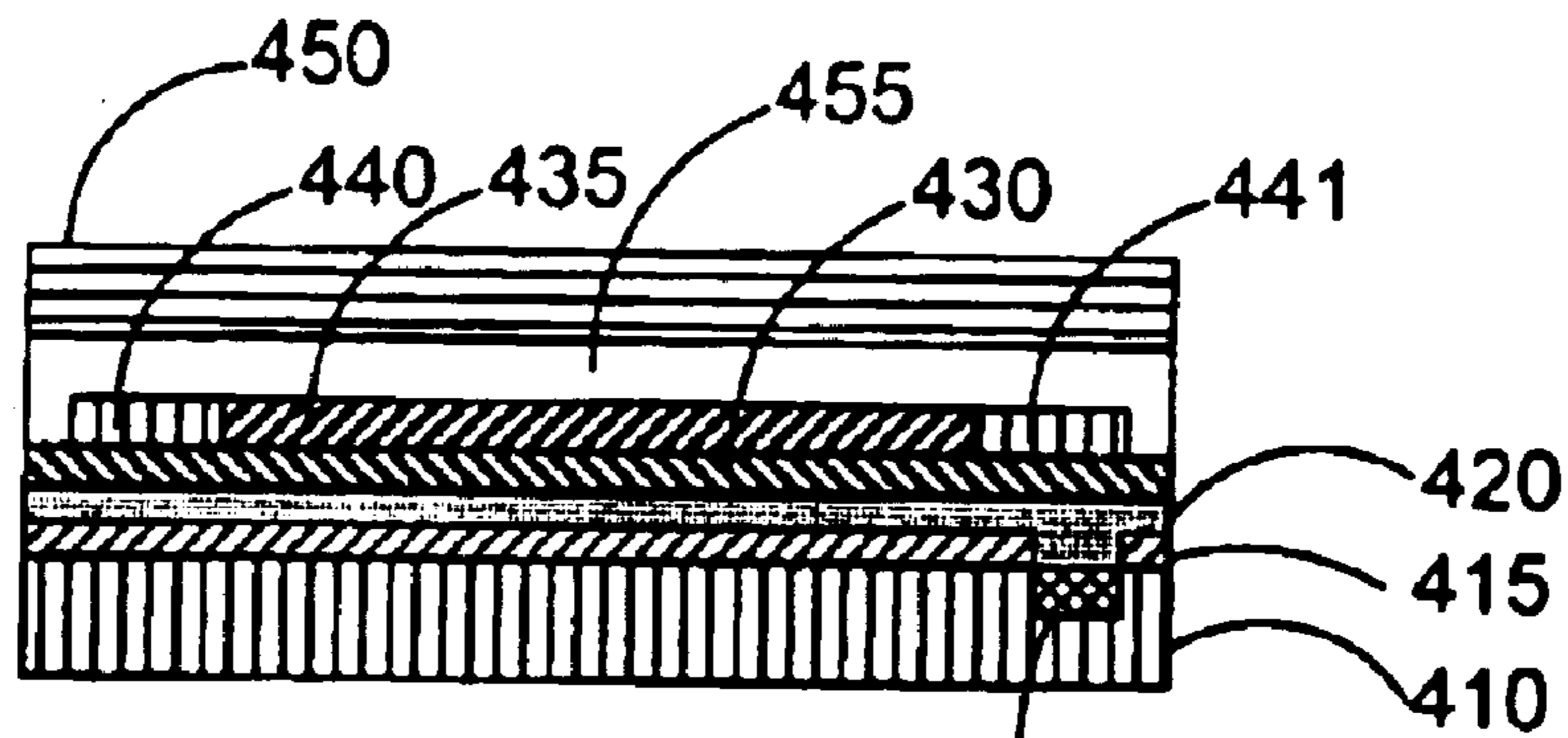
FIG. 12H SECTION B-B
