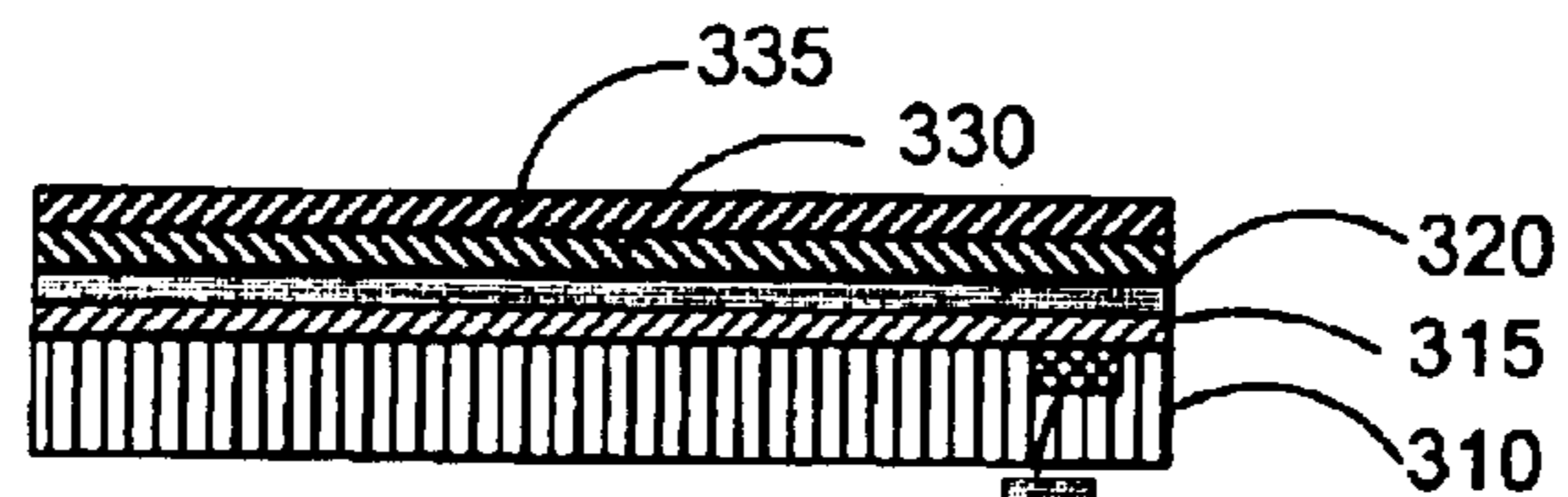
FIG. 9C SECTION B-B
