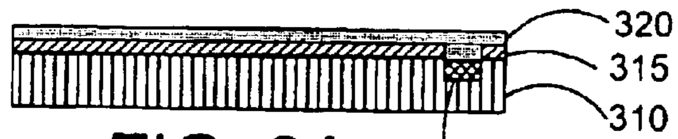
FIG. 9A SECTION B-B
