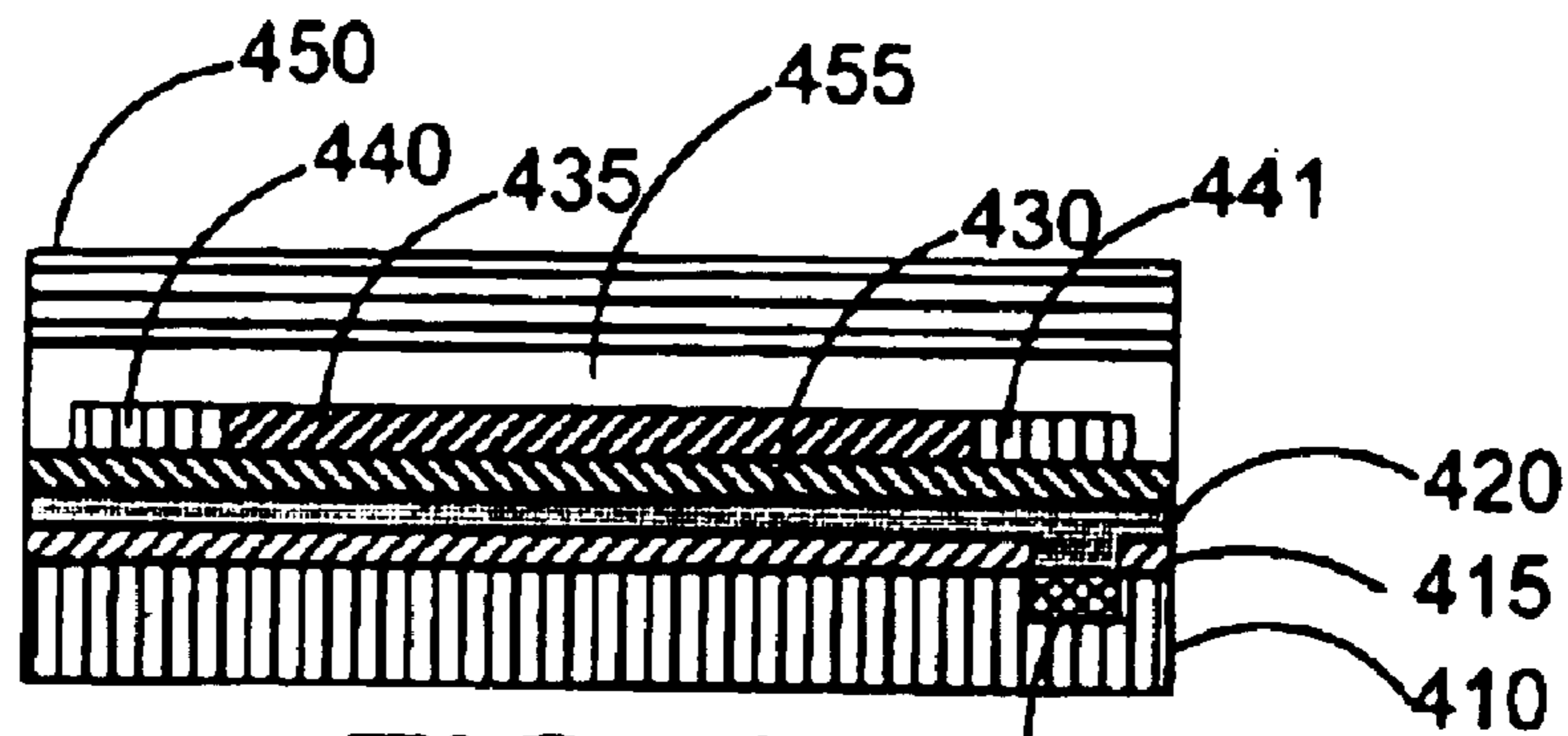
FIG. 12I SECTION B-B
