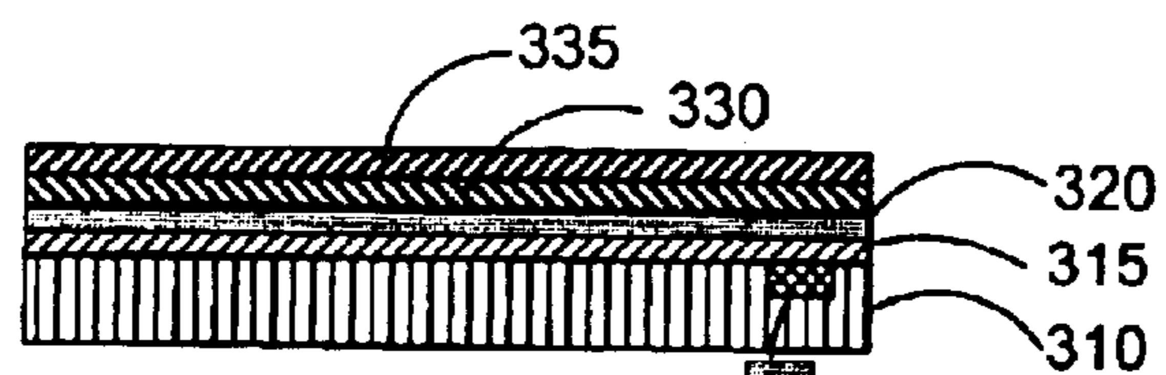
FIG. 9C SECTION B-B
