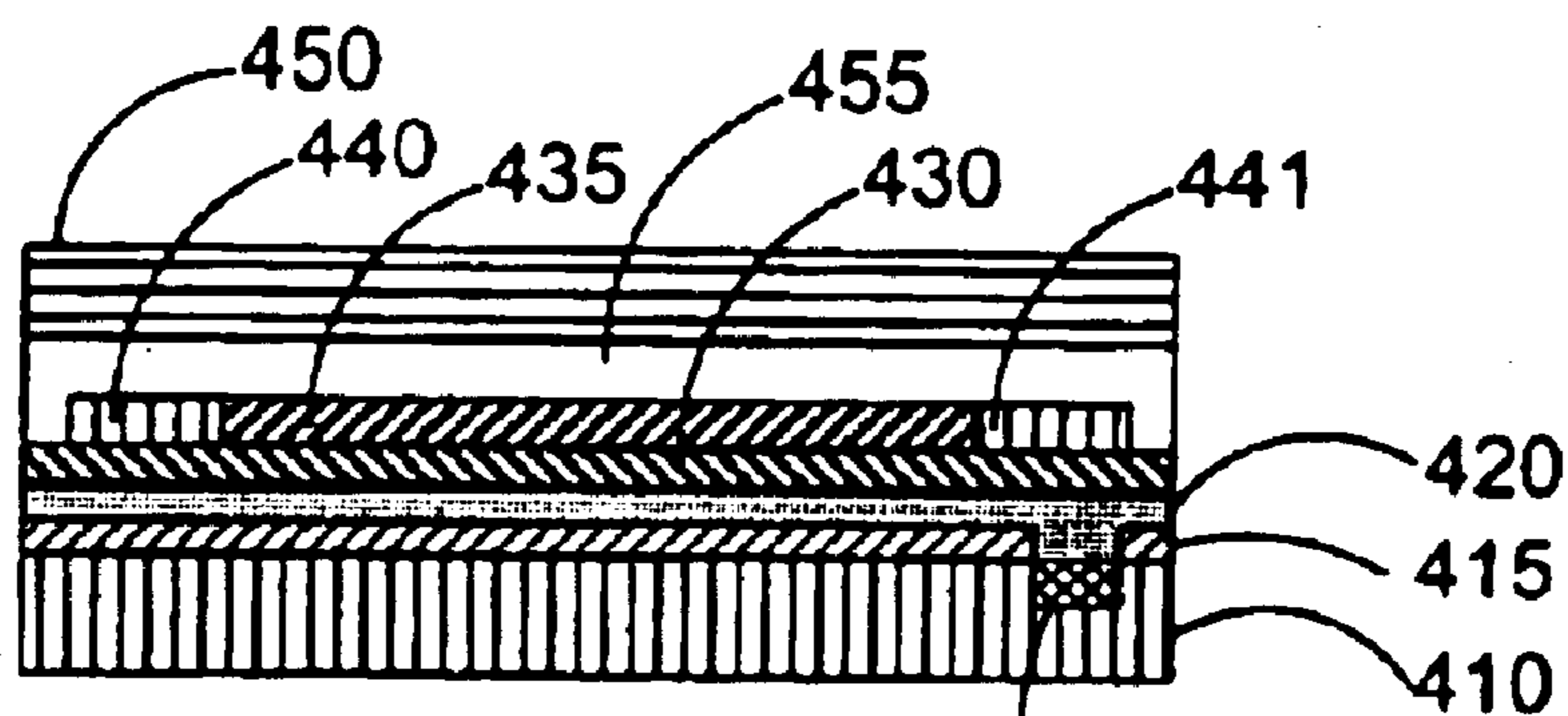
FIG. 12J SECTION B-B
