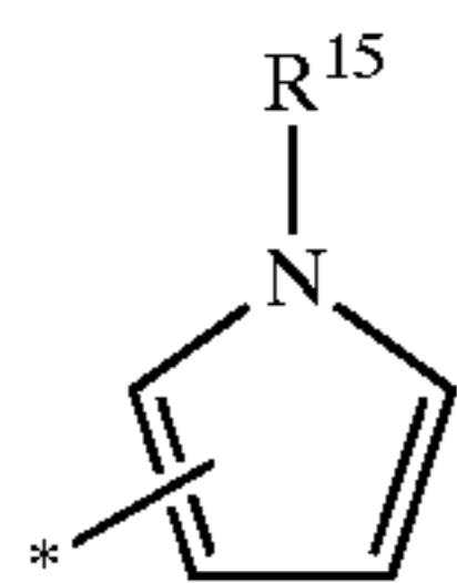
pyrrolyl
