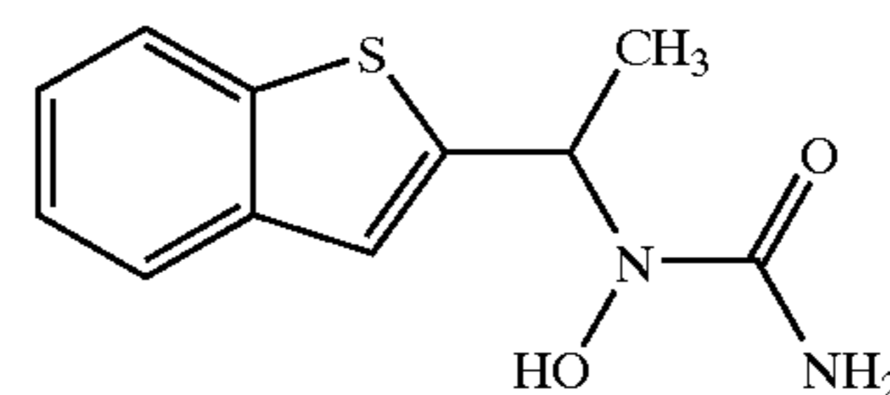
ZYFLO® Zileuton
