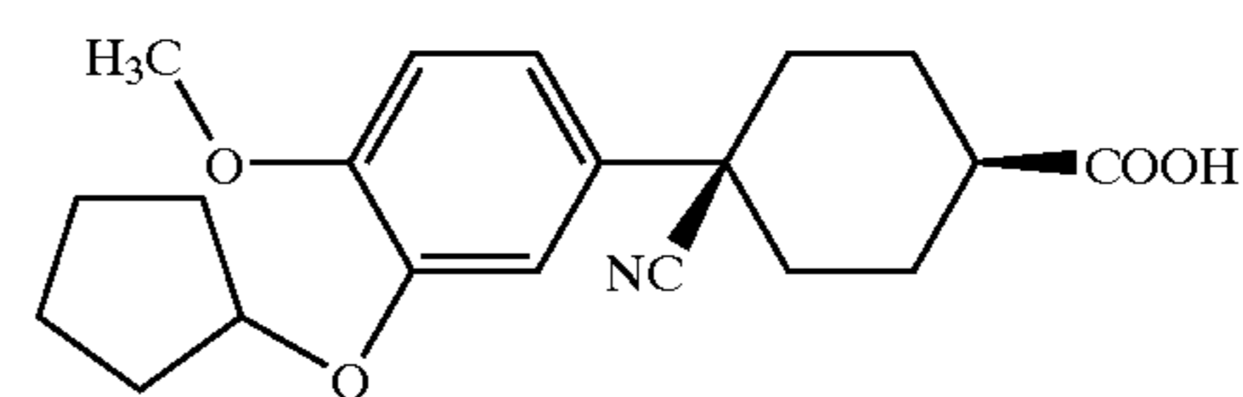
SB-207,499
