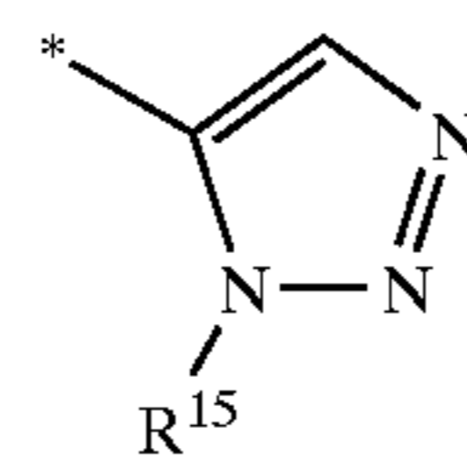
1,2,3-triazol-5-yl
