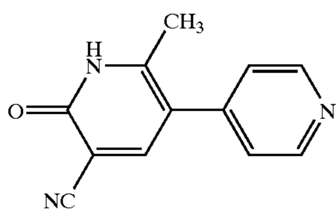
Milrinone
