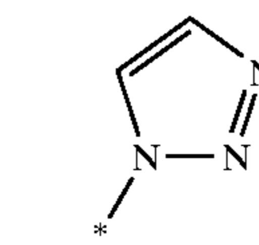
1H-1,2,3-triazol-1-yl
