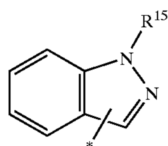
1H-indazolyl
