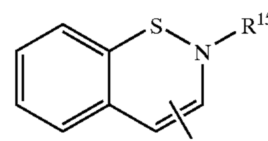
2H-1,2-benzothiazinyl
