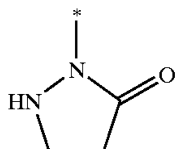
pyrazol-5-on-1-yl
