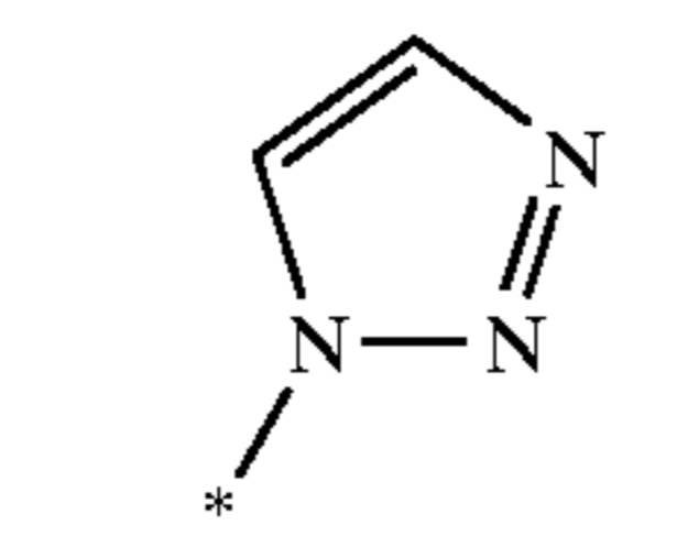
1H-1,2,3-triazol-1-yl
