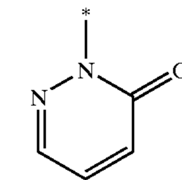
pyridazin-3-on-2-yl
