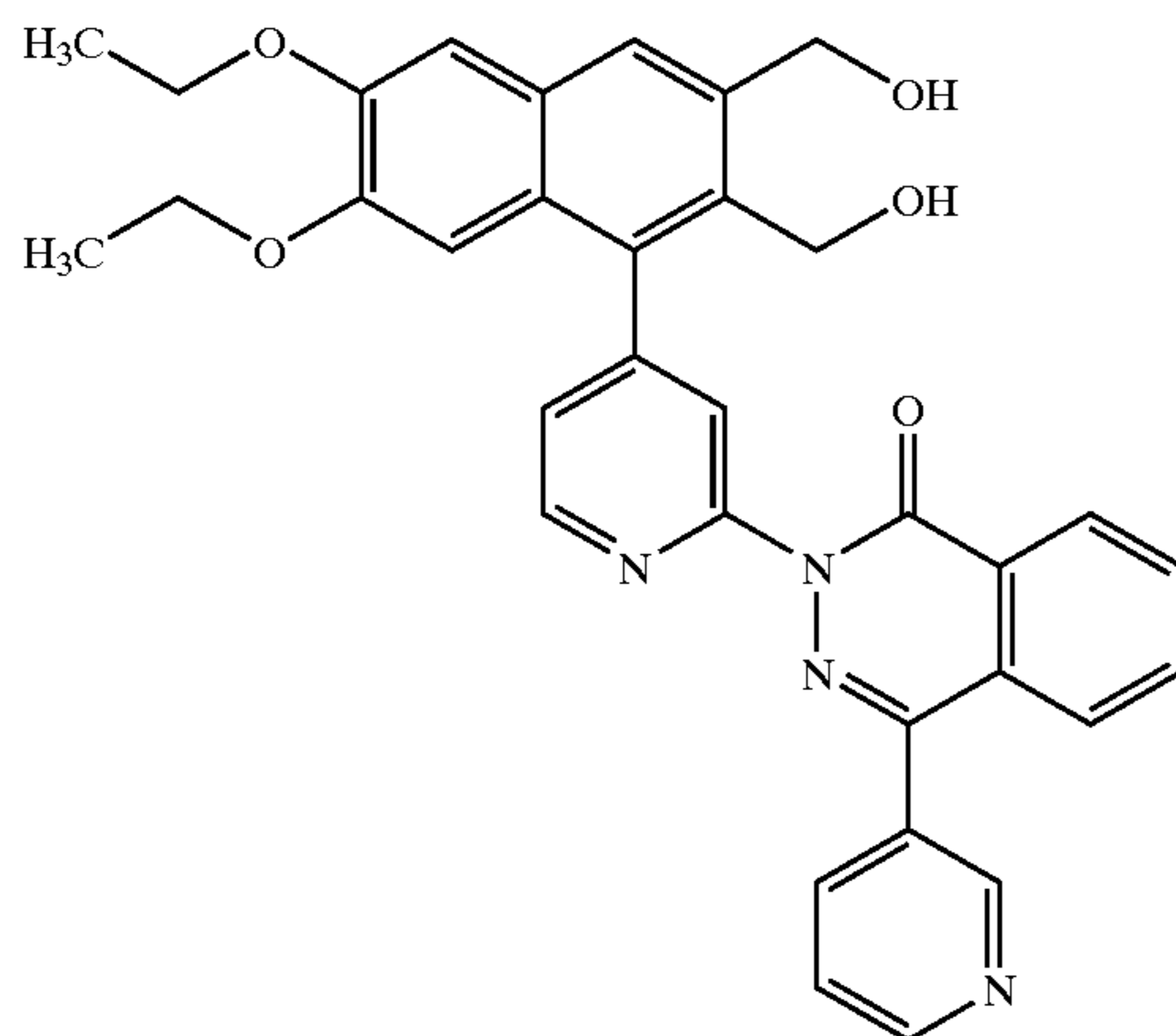
T-2585
