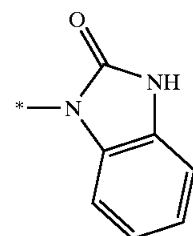
1H-benzimidazol-2- on-3-yl
