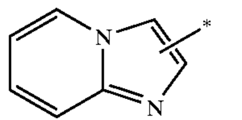
imidazo-[1,2-a]- pyridinyl
