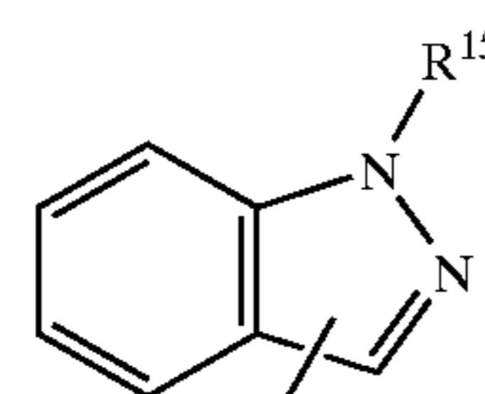
1H-indazolyl
