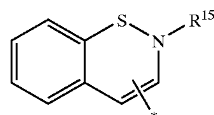
2H-1,2-benzothiazinyl
