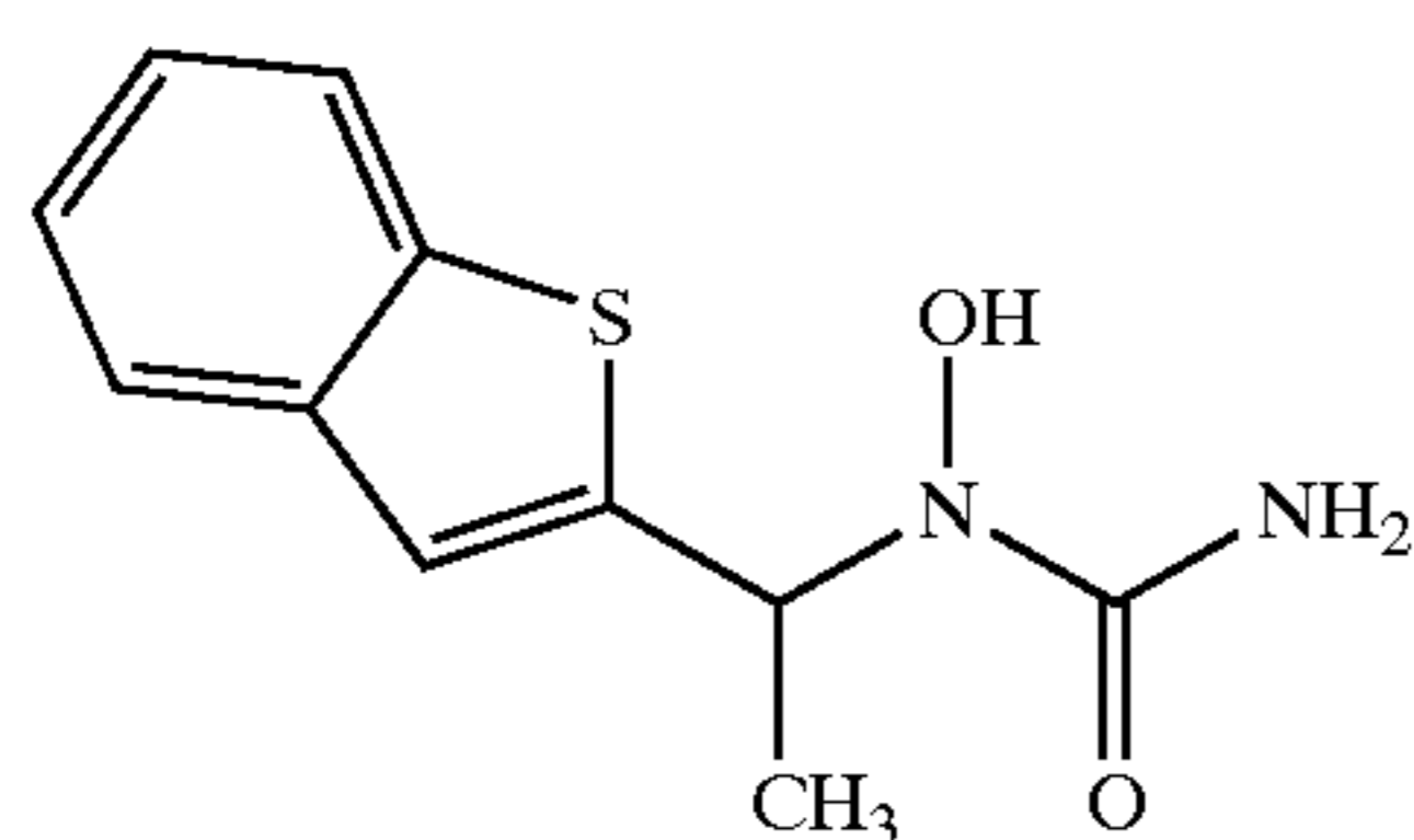
Zileuton
