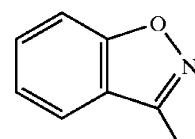
benzisoxazolyl
