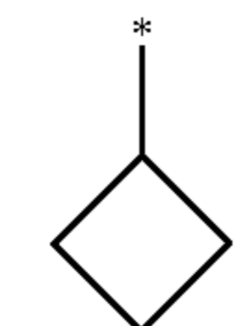
cyclobutyl
