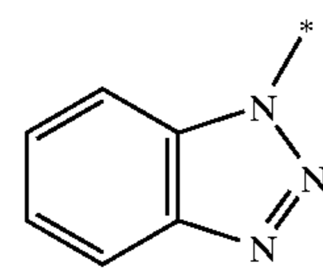
benzotriazolyl
