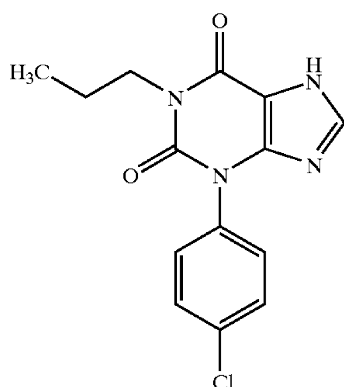
Arofylline (LAS-31025)
