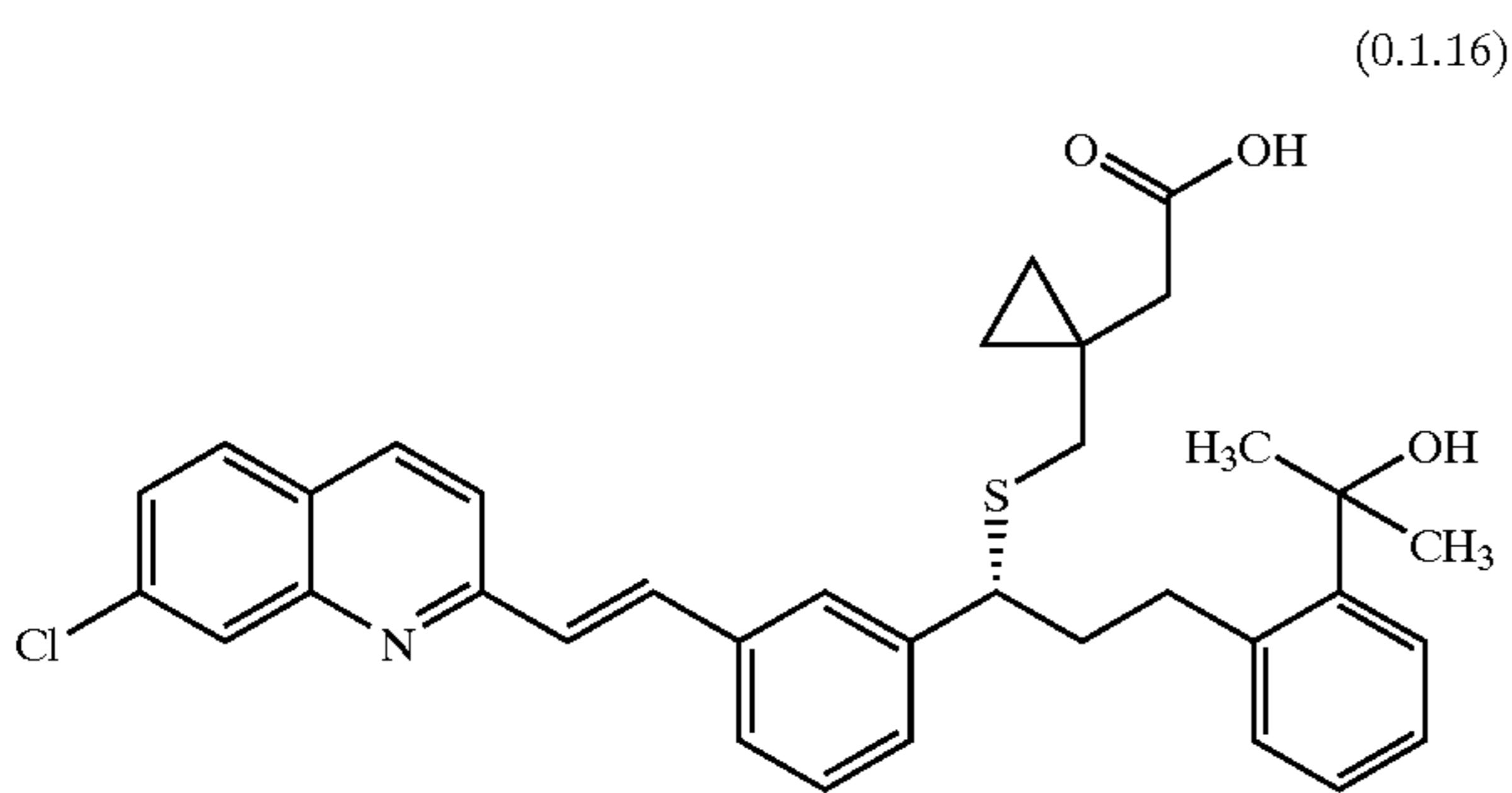
SINGULAIR® Montelukast
