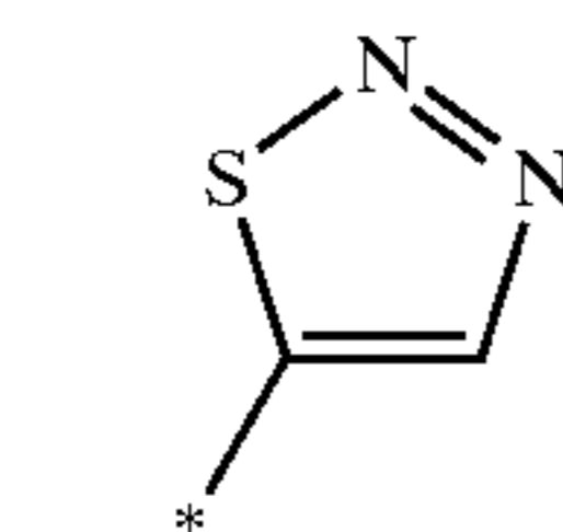
1,2,3-thiadiazol-5-yl
