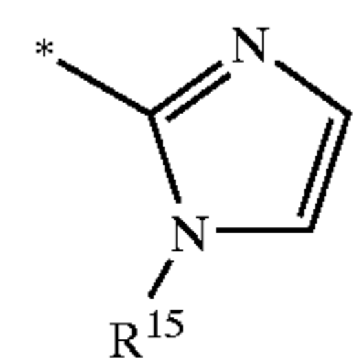
imidazol-2-yl
