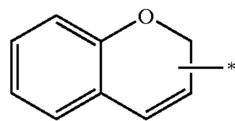
2H-1-benzopyranyl
