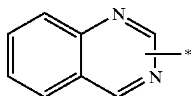
quinazoliny
