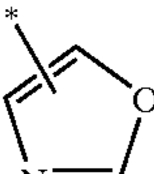
oxazolyl
