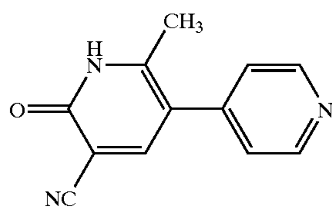
Milrinone
