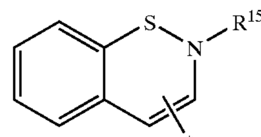
2H-1,2-benzothiazinyl
