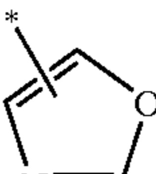
oxazolyl
