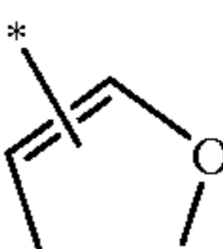
isoxazolyl
