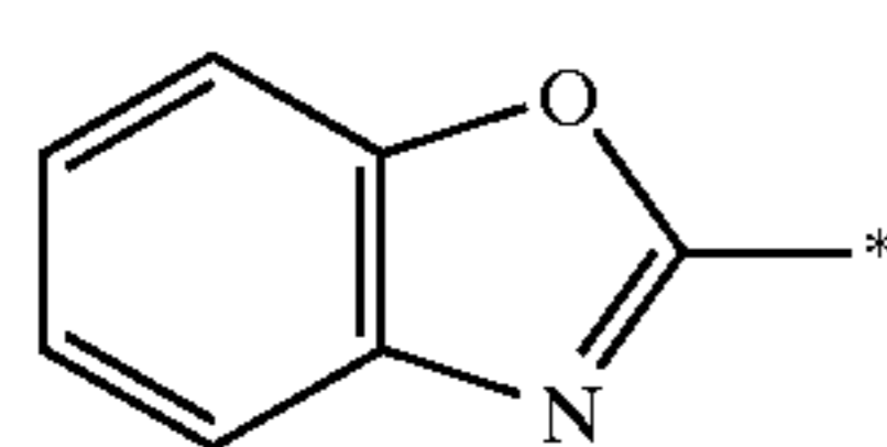
benzoxazolyl
