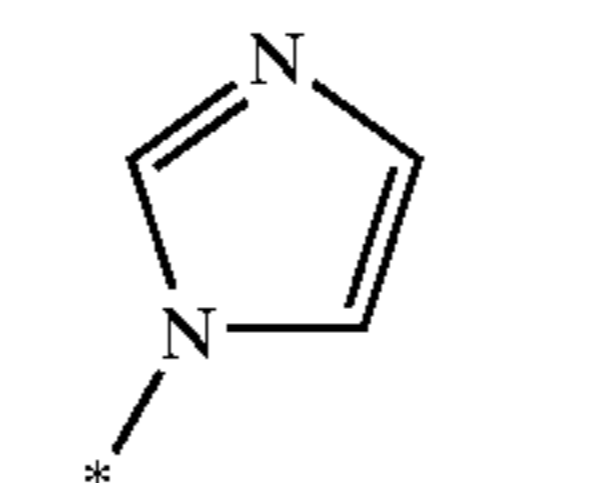
imidazol-1-yl
