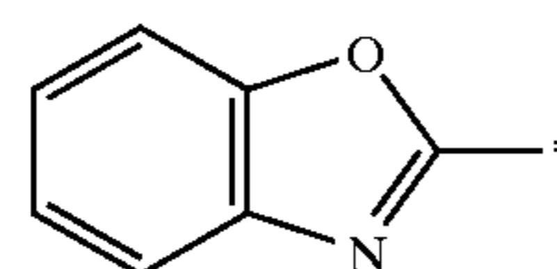
benzoxazolyl
