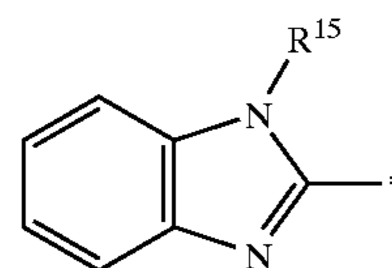
benzimidazolyl
