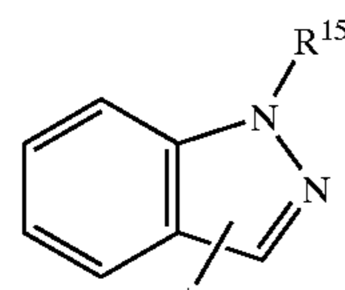
1H-indazolyl
