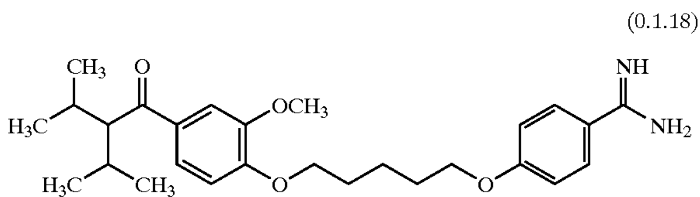
CGS-25019c
