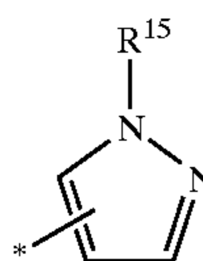
pyrazolyl
