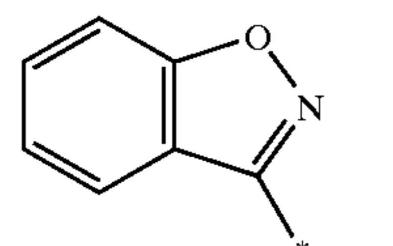
benzisoxazolyl
