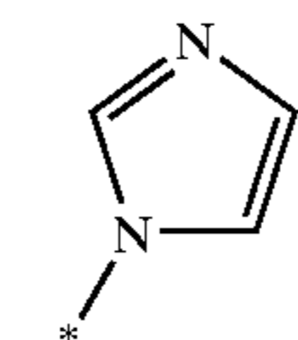
imidazol-1-yl
