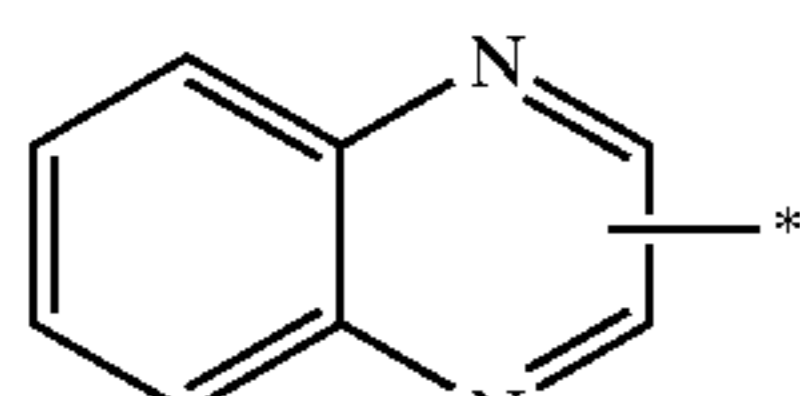
quinoxaliny
