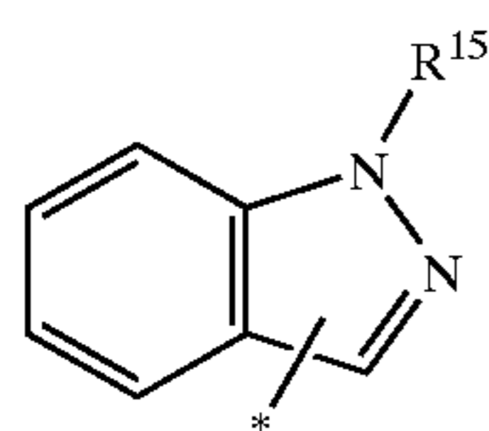
1H-indazolyl
