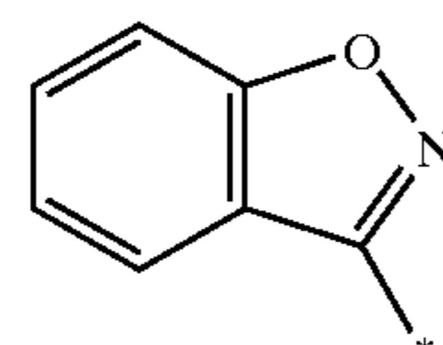
benzisoxazolyl
