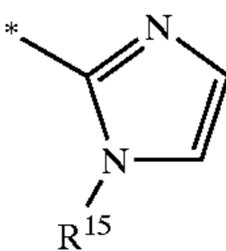
imidazol-2-yl
