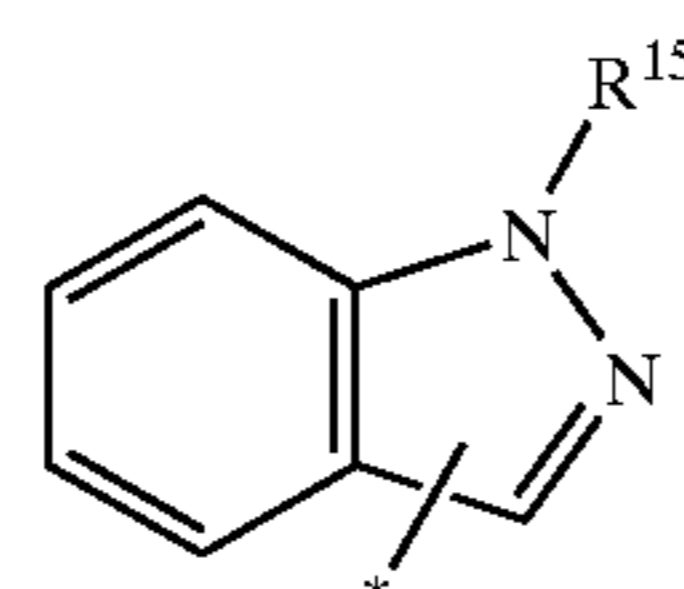
1H-indazolyl
