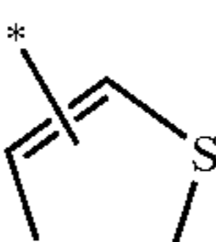
thiazolyl
