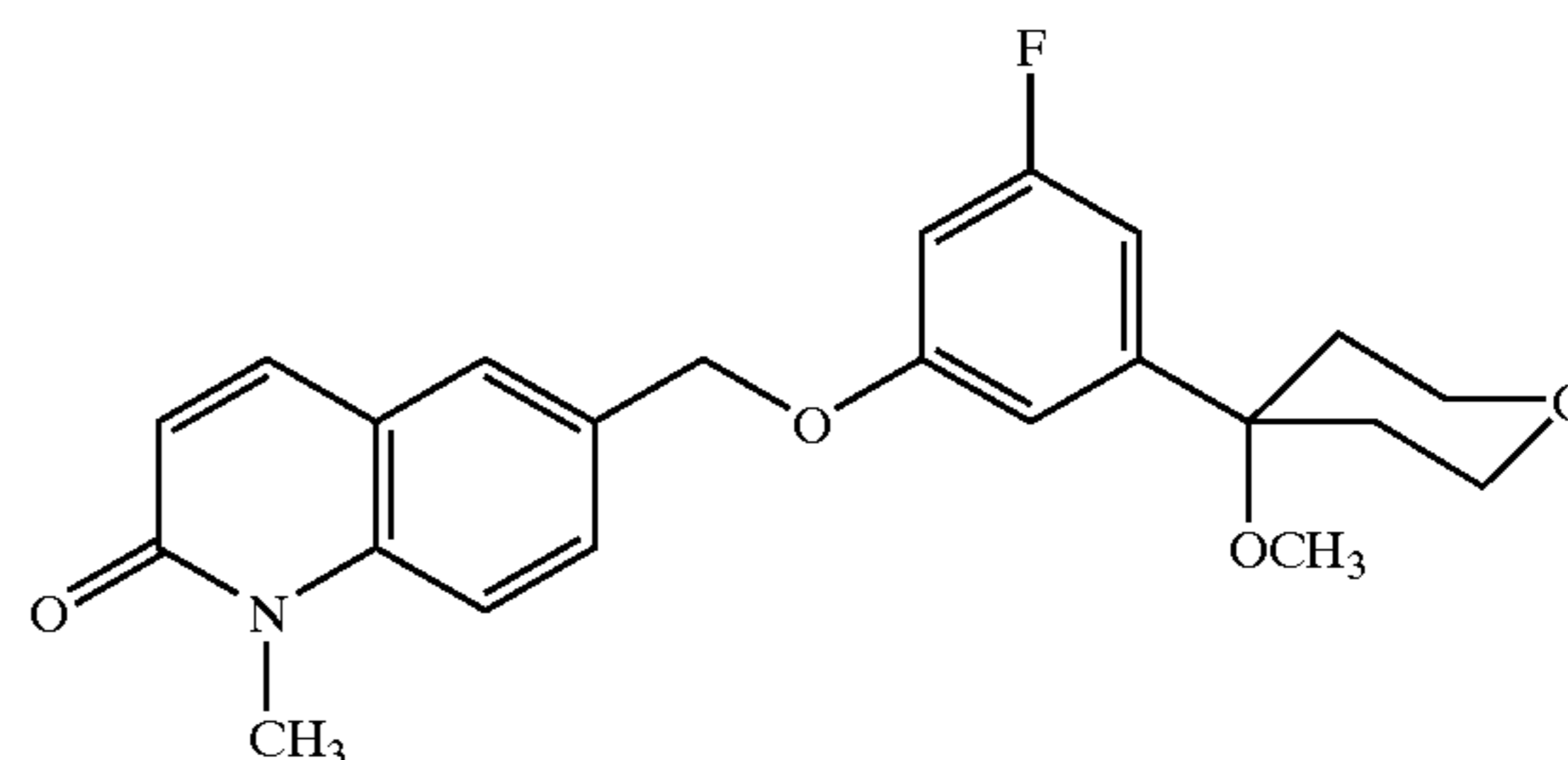
(5.2.11)
