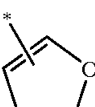
isoxazolyl
