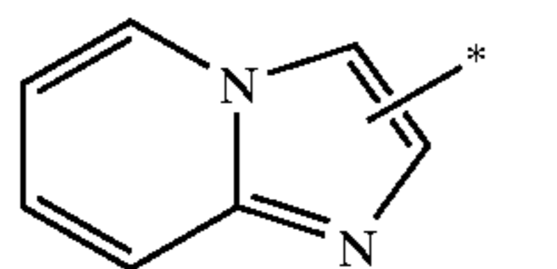
imidazo-[1,2-a]- pyridinyl
