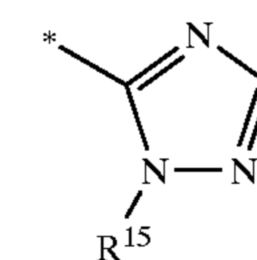
1,2,4-triazol-3-yl
