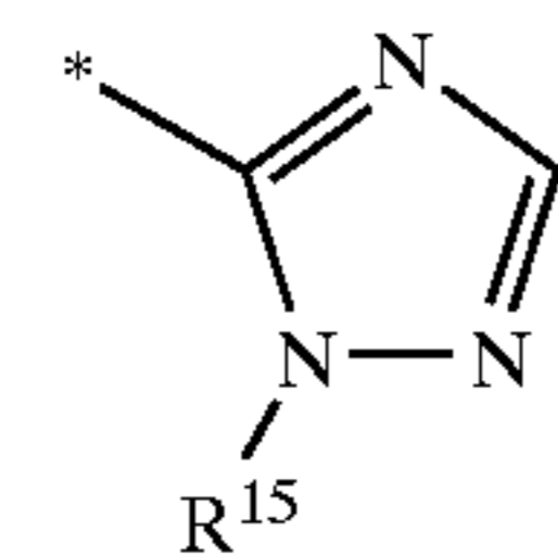
1,2,4-triazol-3-yl
