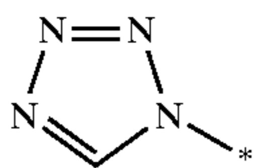
tetrazol-1-yl
