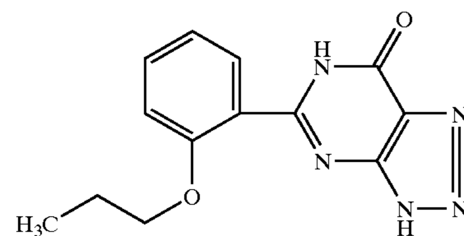
Zaprinast
