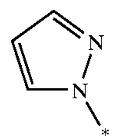
pyrazol-1-yl
