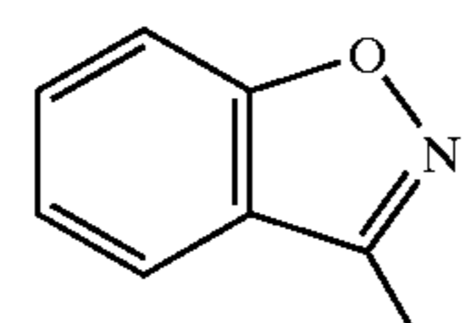
benzisoxazolyl
