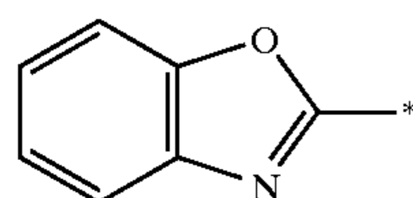
benzoxazolyl
