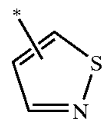
isothiazolyl
