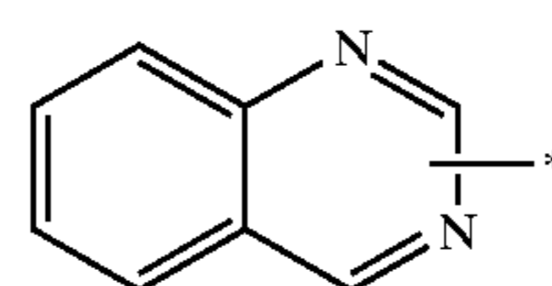
quinazoliny
