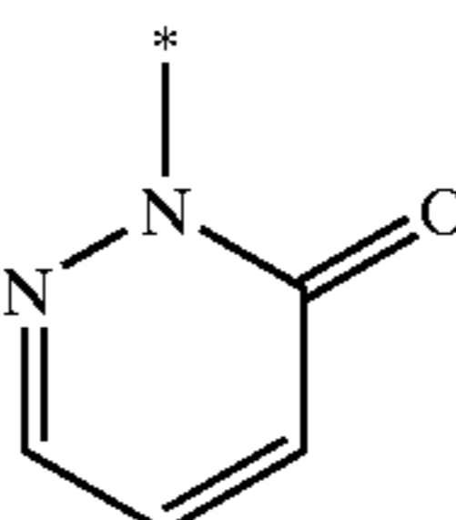
pyridazin-3-on-2-yl
