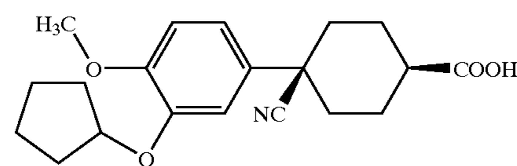
SB-207,499
