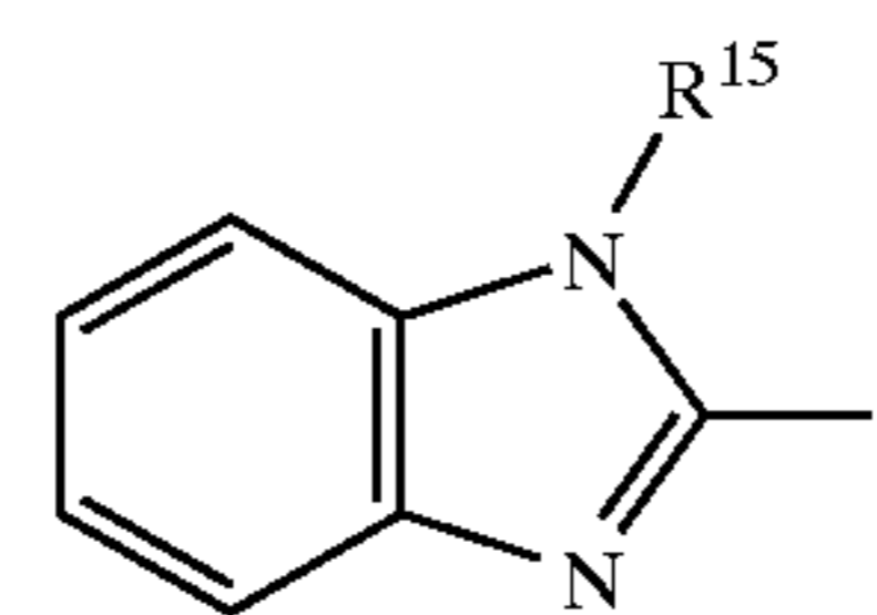
benzimidazolyl
