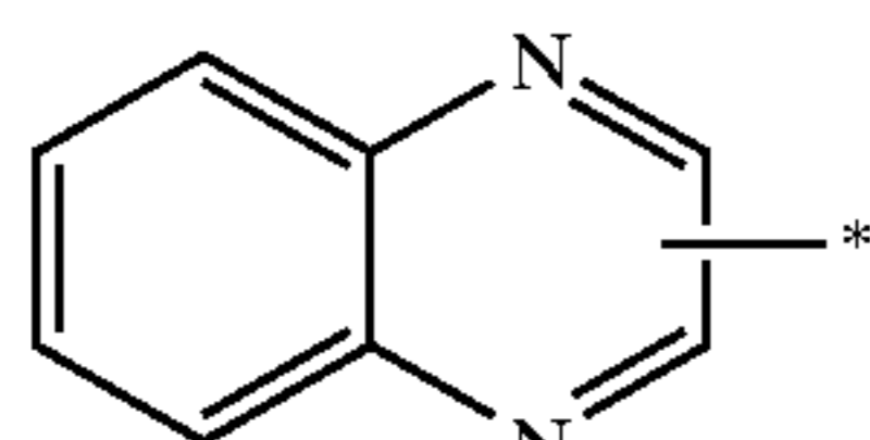
quinoxaliny
