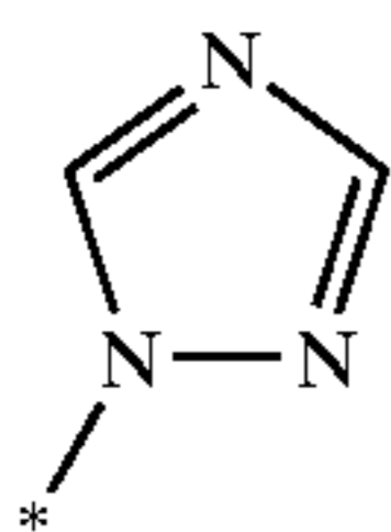
1H-1,2,4-triazol-1-yl
