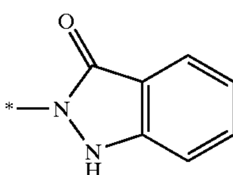
1H-indazol-3-on-2-yl
