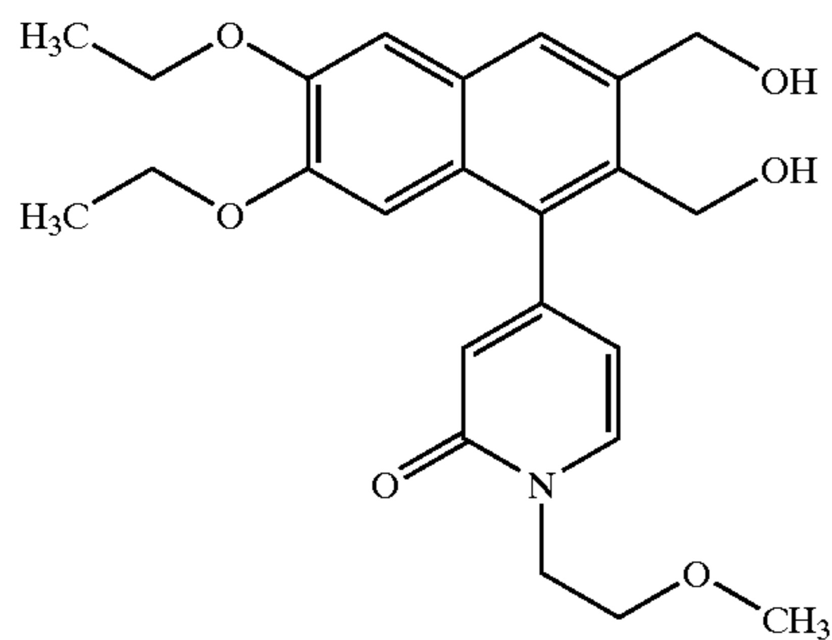
T-440
