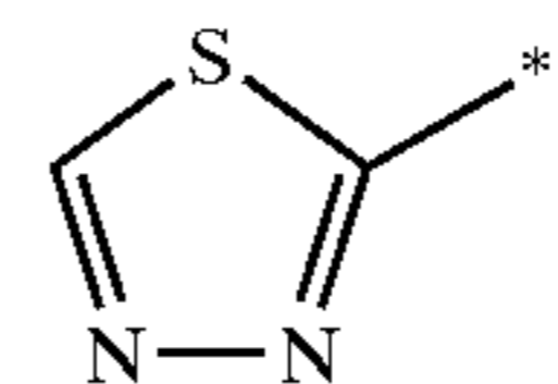
1,3,4-thiadiazolyl
