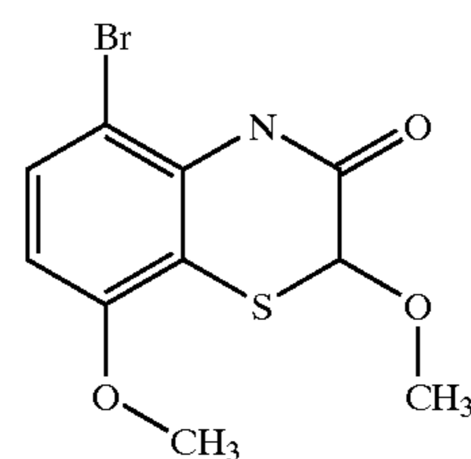
L-651,392
