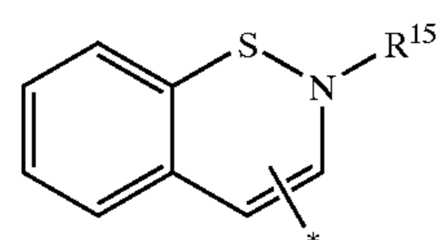
2H-1,2-benzothiazinyl
