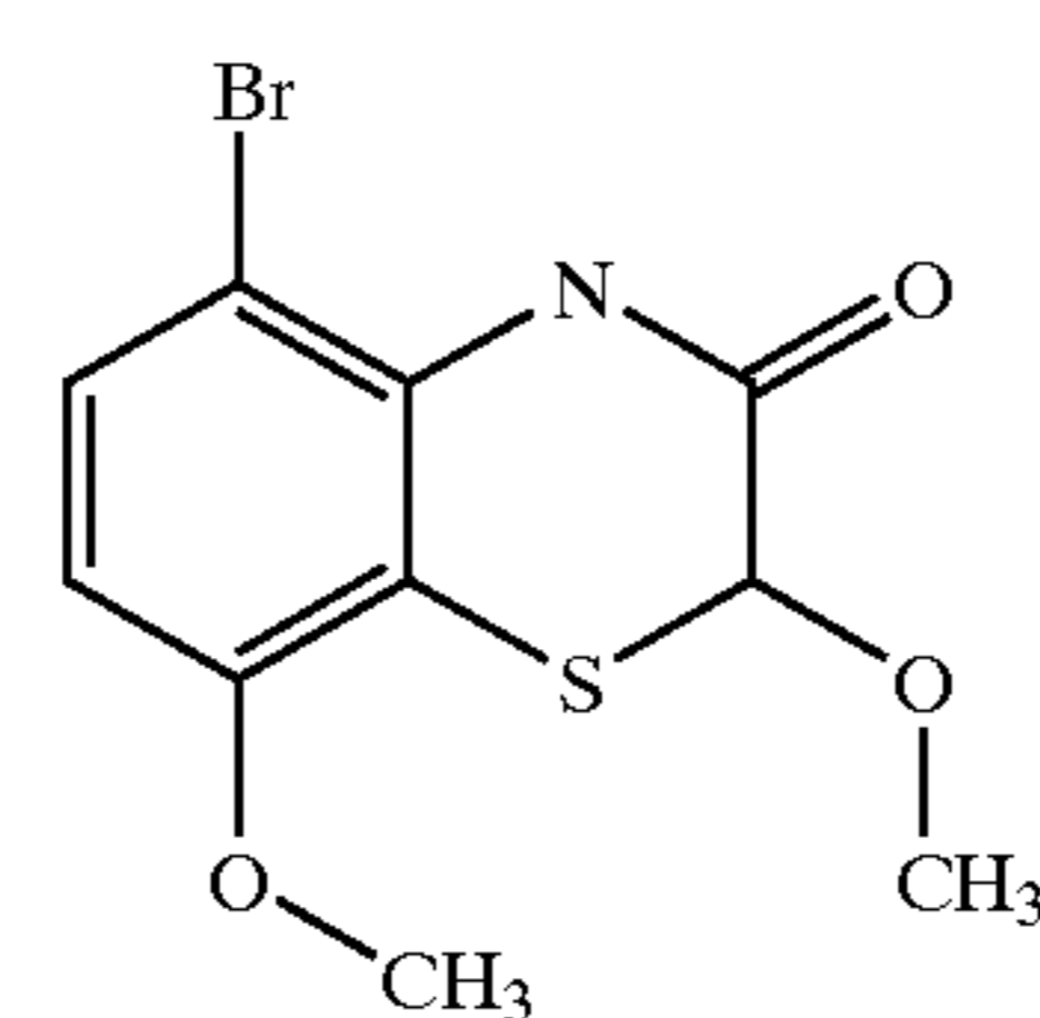
L-651,392
