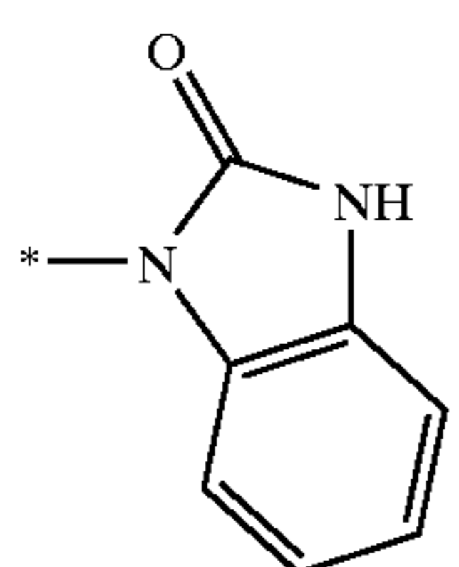
1H-benzimidazol-2-on-3-yl
