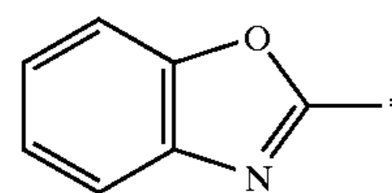
benzoxazolyl
