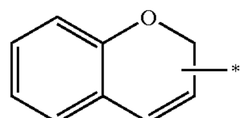
2H-1-benzopyranyl
