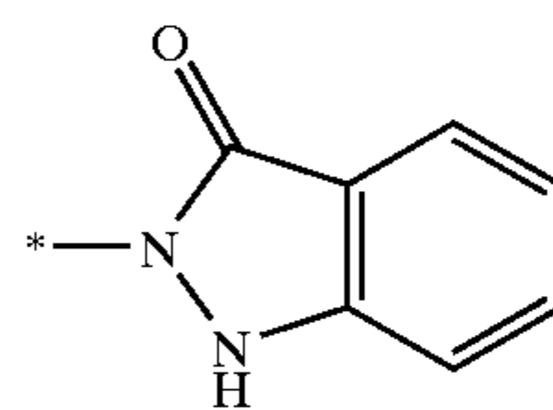
1H-indazol-3-on-2-yl
