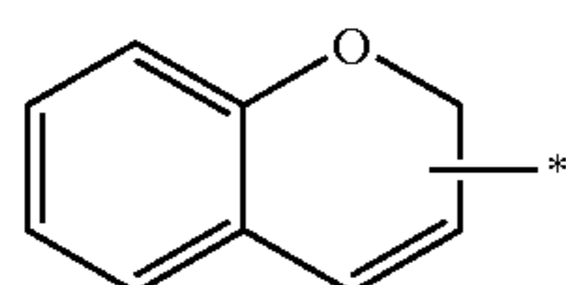
2H-1-benzopyranyl
