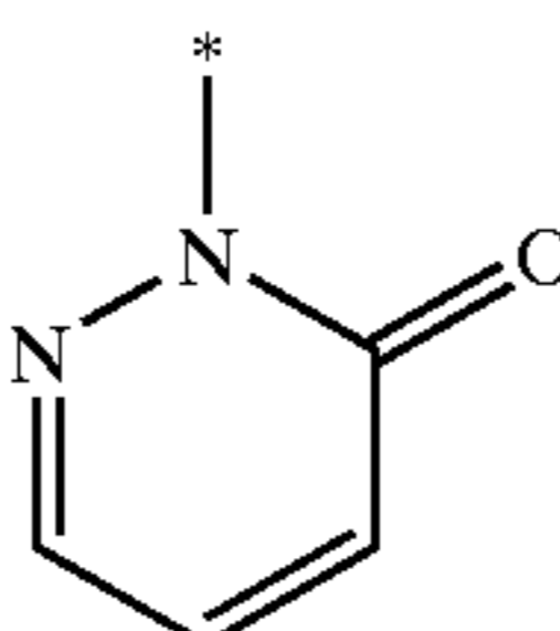
pyridazin-3-on-2-yl
