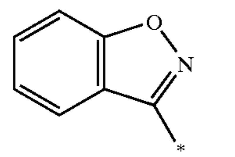
benzisoxazolyl
