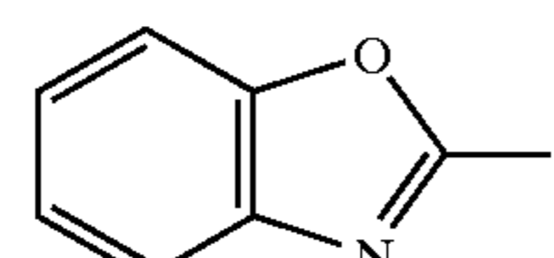
benzoxazolyl
