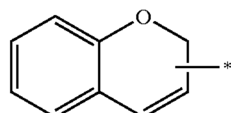
2H-1-benzopyranyl
