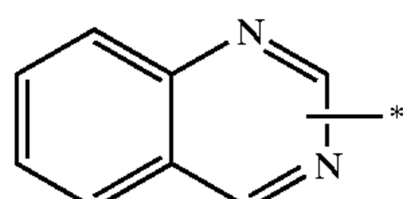
quinazoliny
