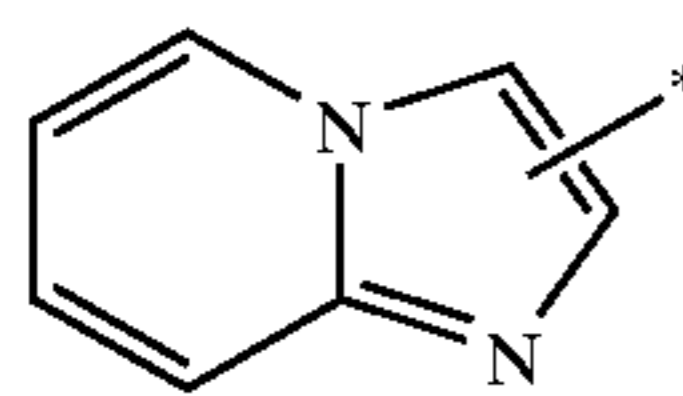
imidazo-[1,2-a]- pyridinyl
