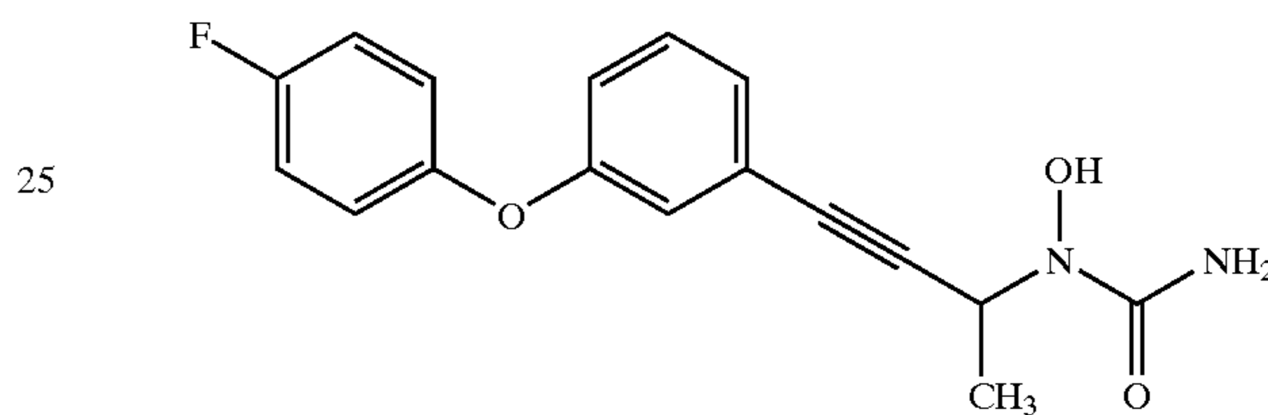
Fenleuton
