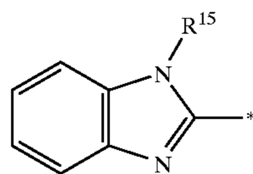
benzoimidazolyl
