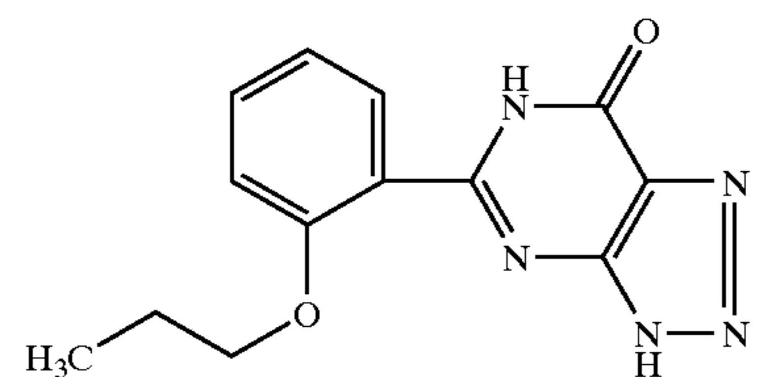
Zaprinast
