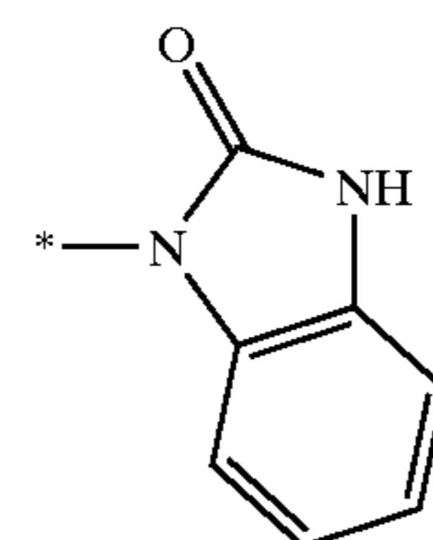
1H-benzimidazol-2- on-3-yl
