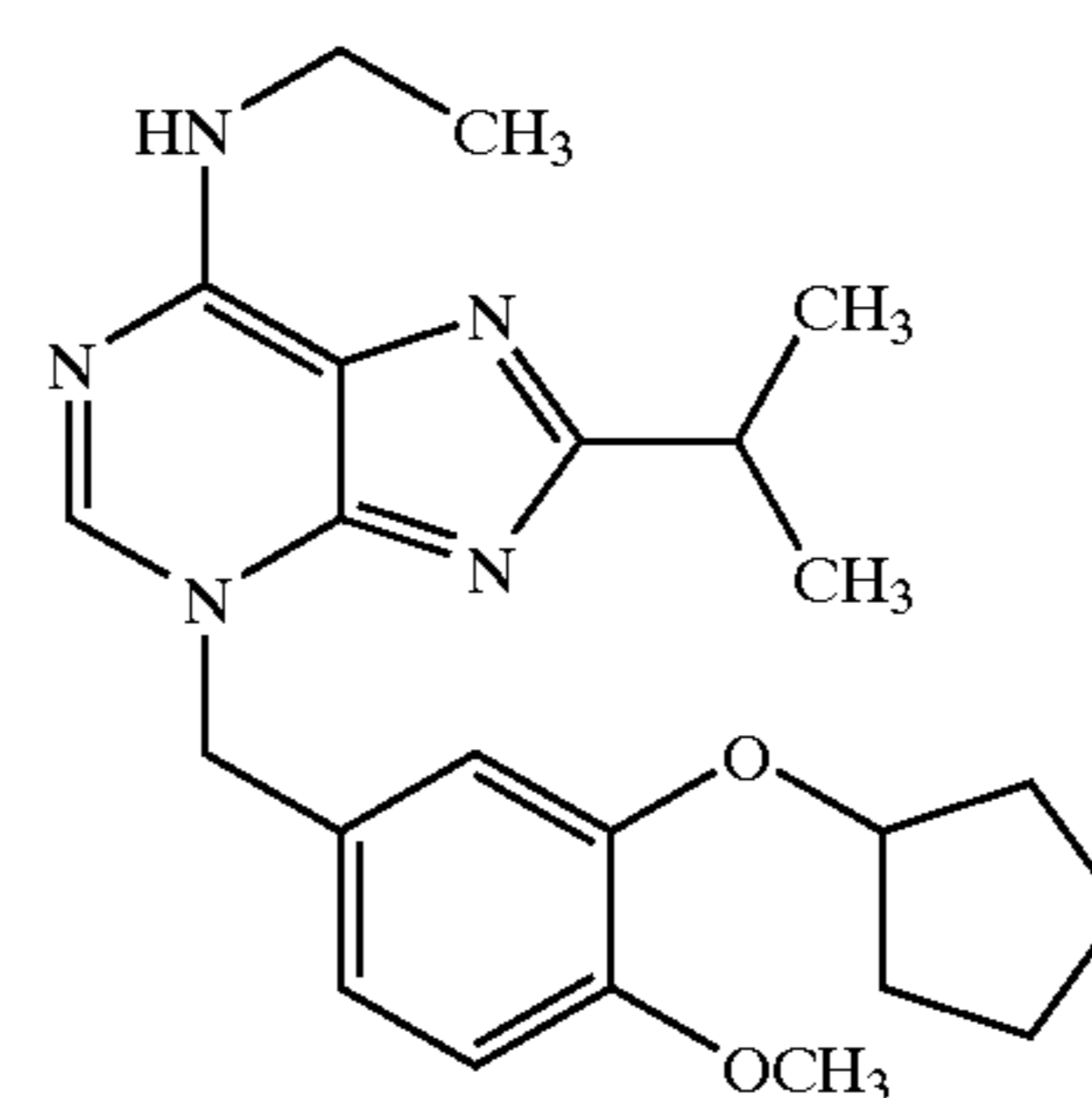
V-11294A
