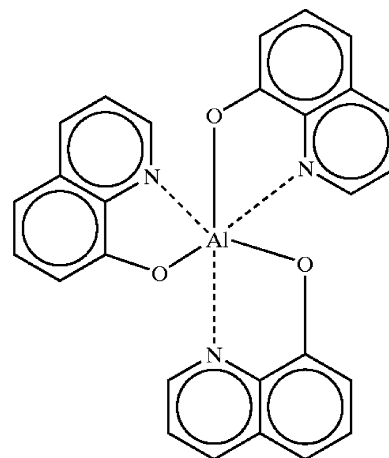
Alq3
