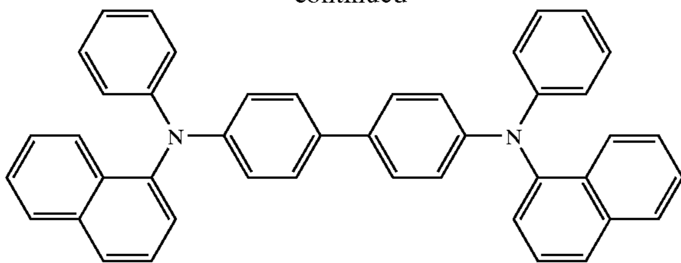
\alpha -NPD
