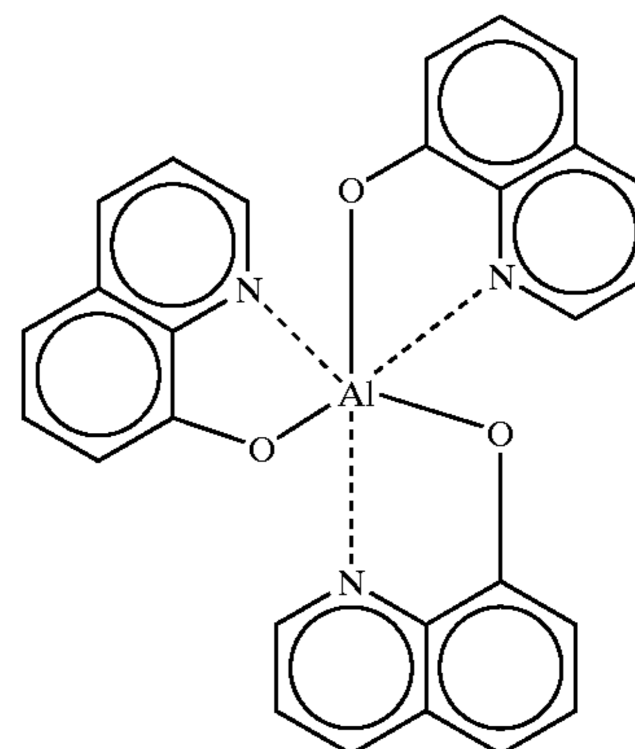
Alq3
