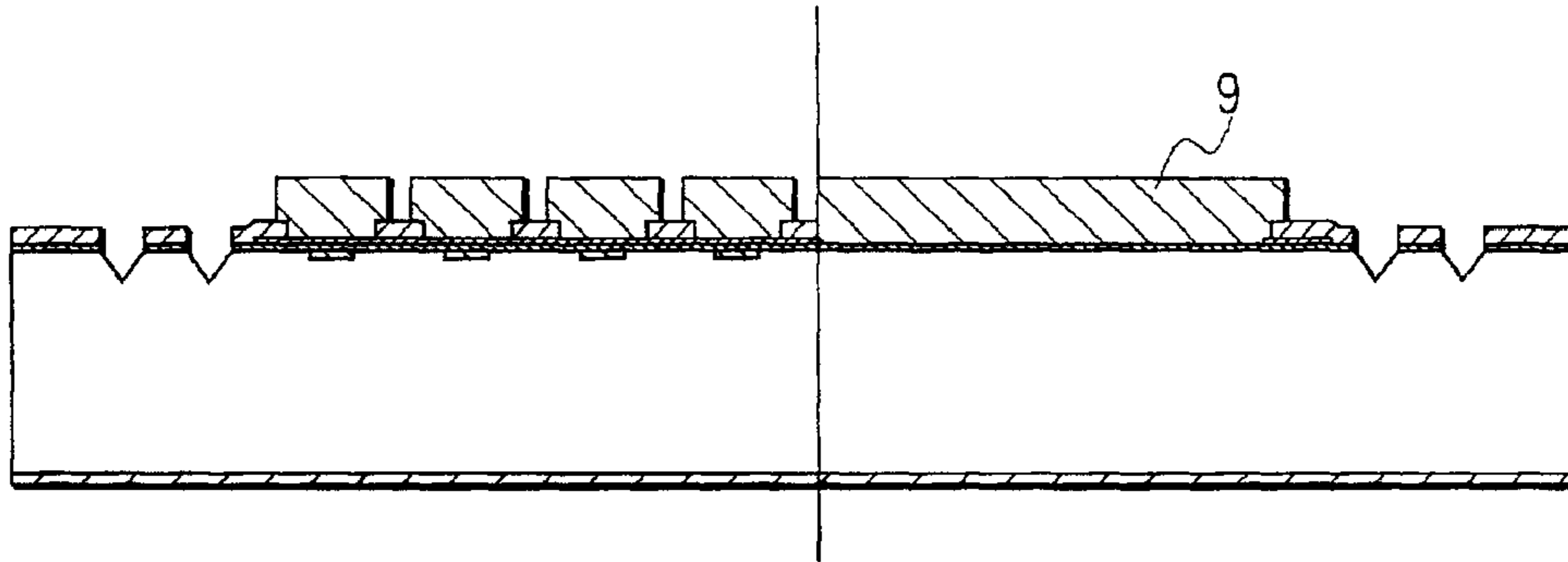
FIG. 3E
