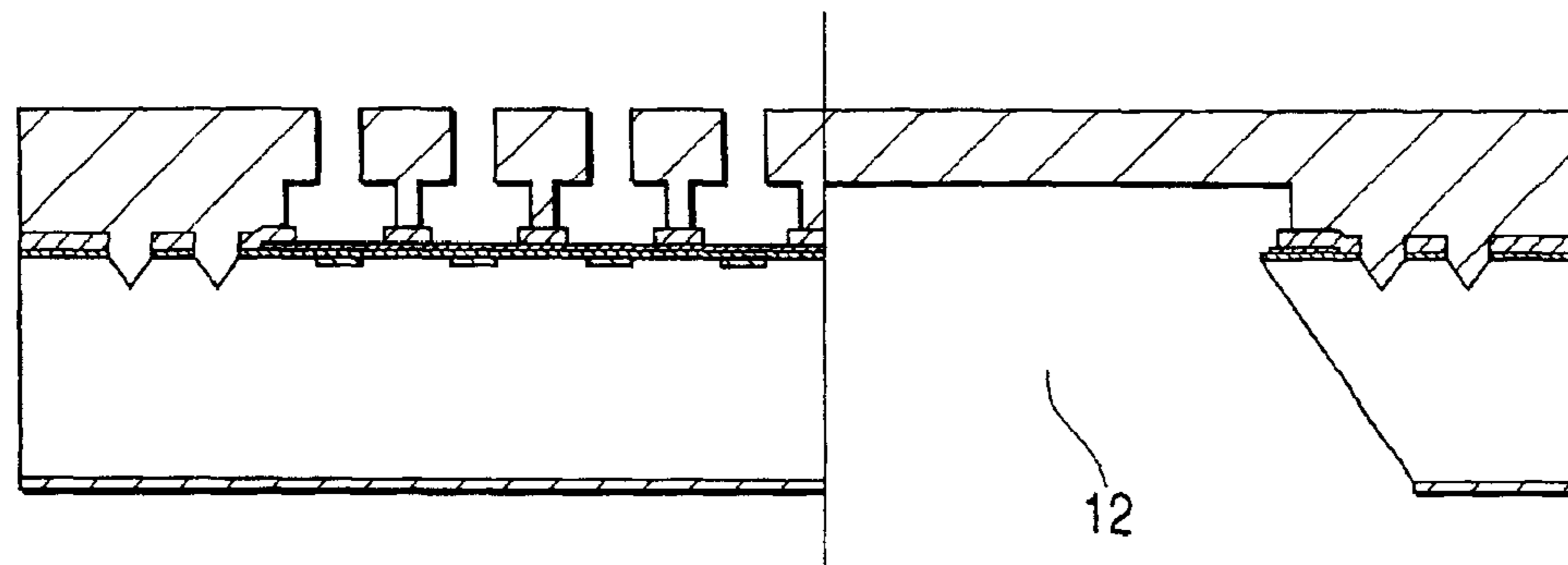
FIG. 3G
