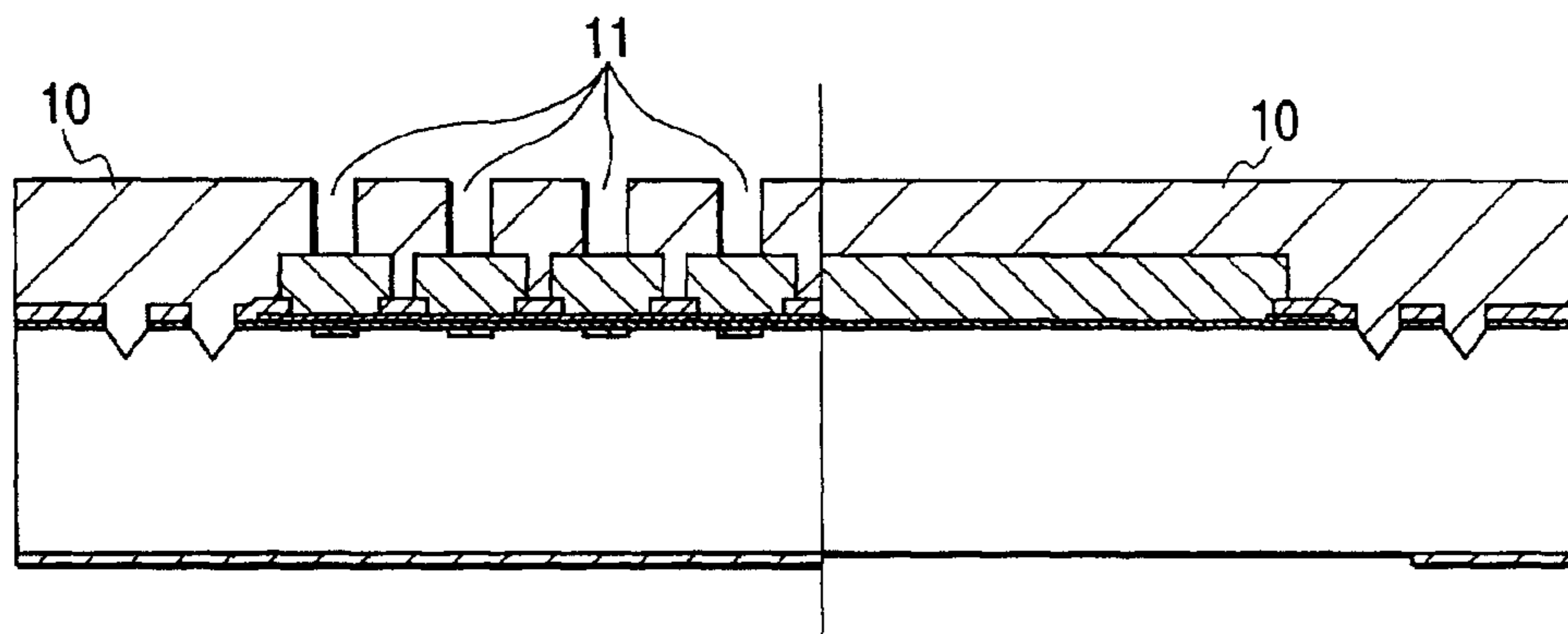
FIG. 3F
