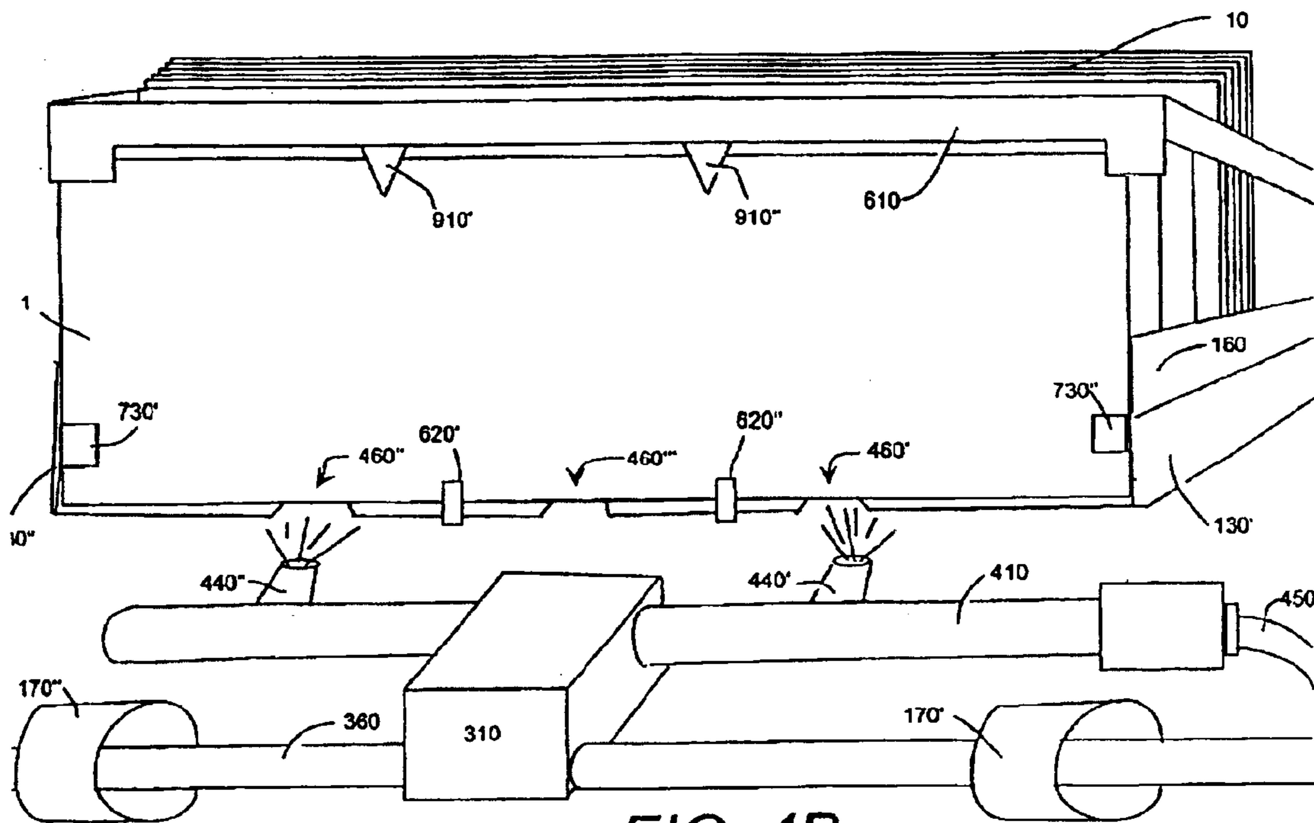
AIR JET FUNCTION FIG. 4B
