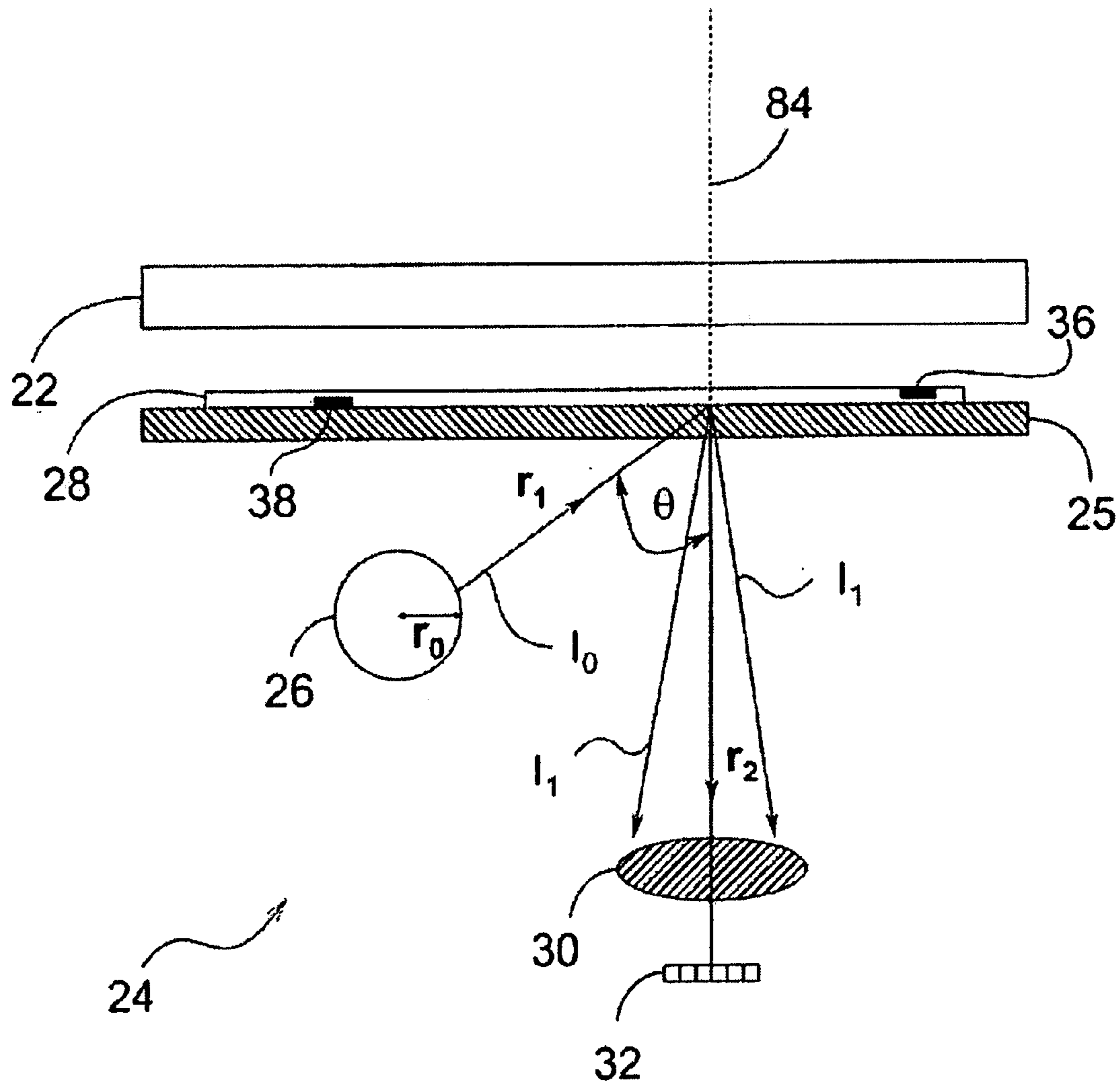
FIG. 2 -- PRIOR ART --
