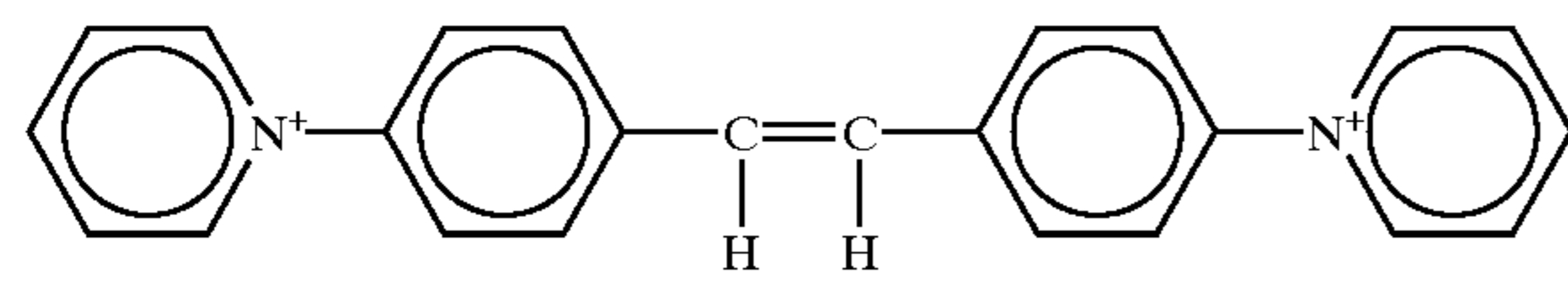
SN 18071
