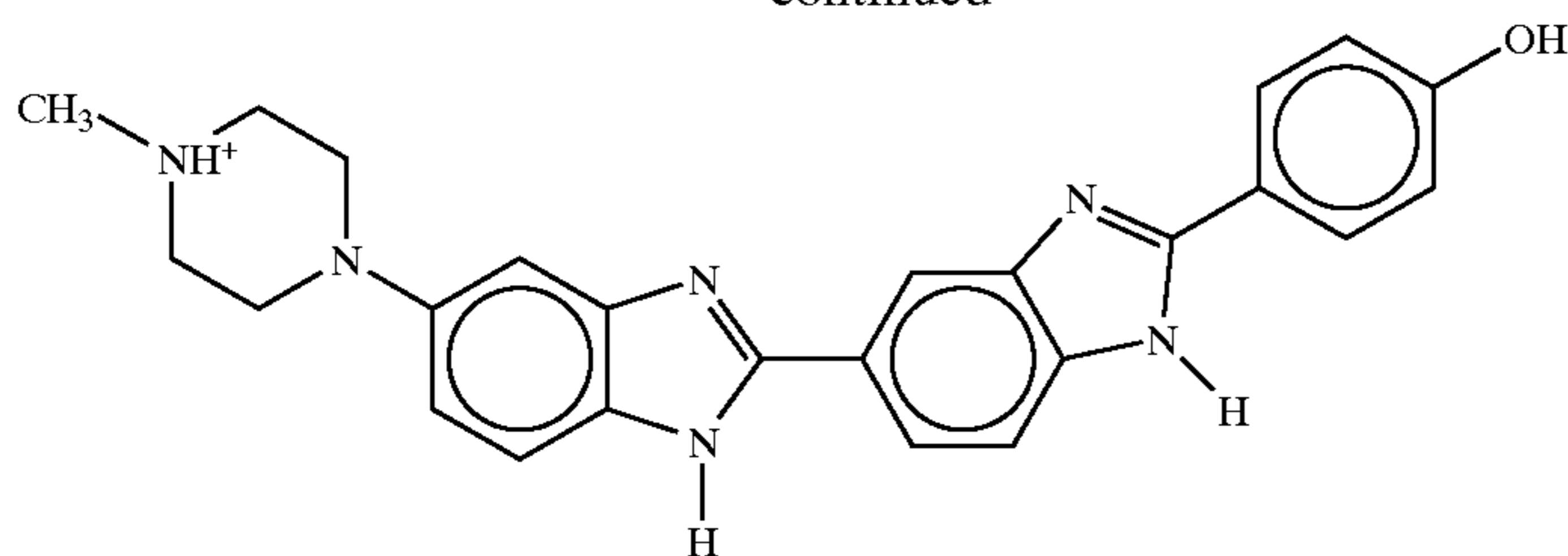
Hoechst 33258
