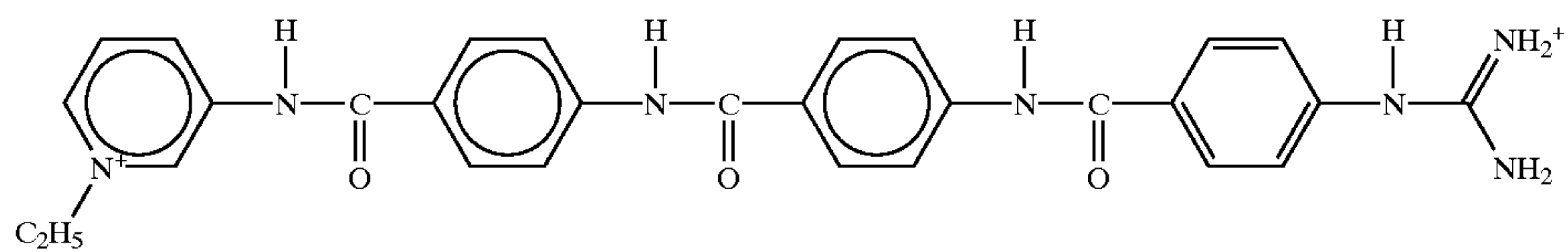
SN 6136
