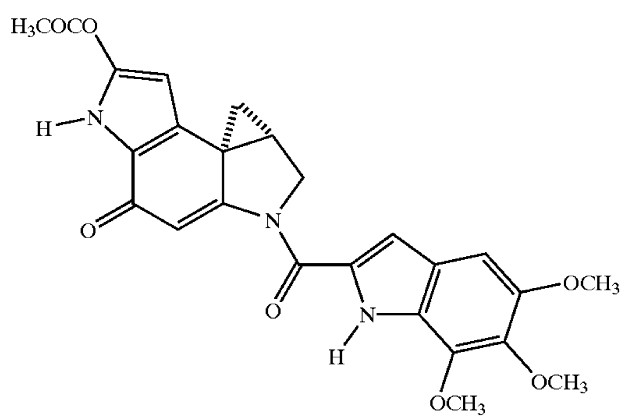
Duocarmycin SA
