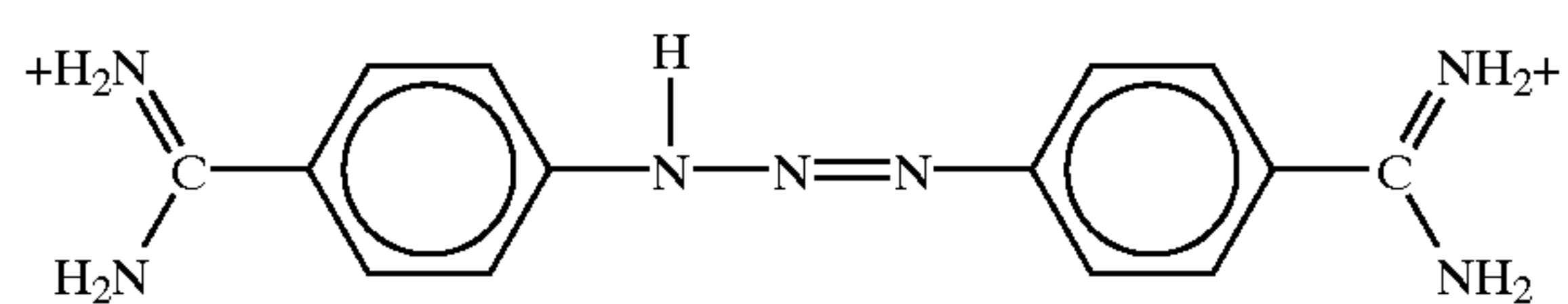
Berenil
