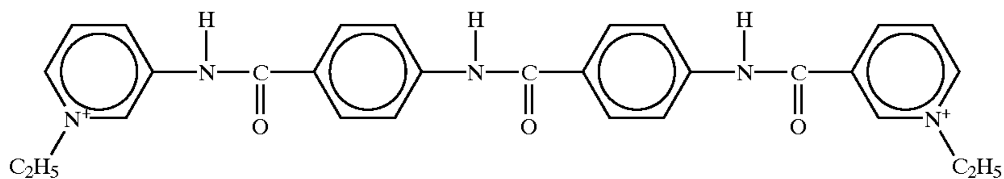
NSC 101327
