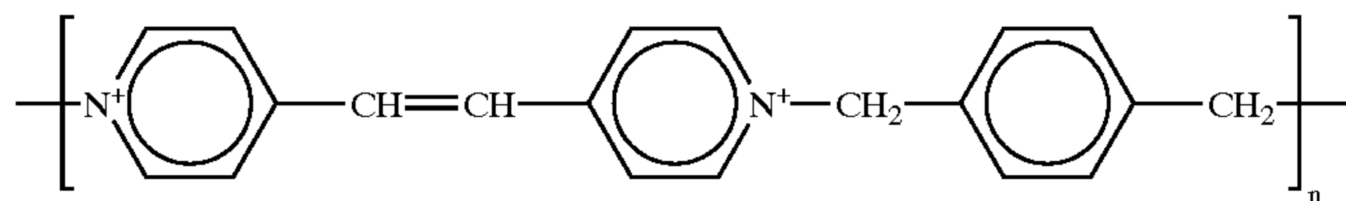
Ionen X
