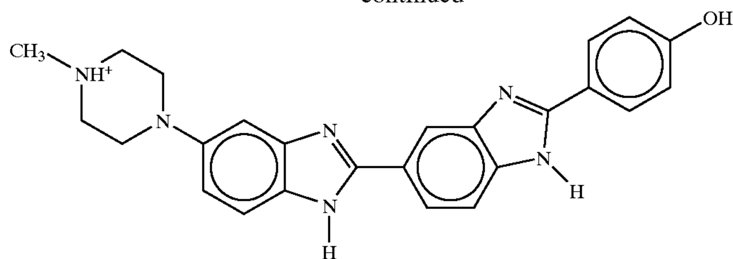
Hoechst 33258
