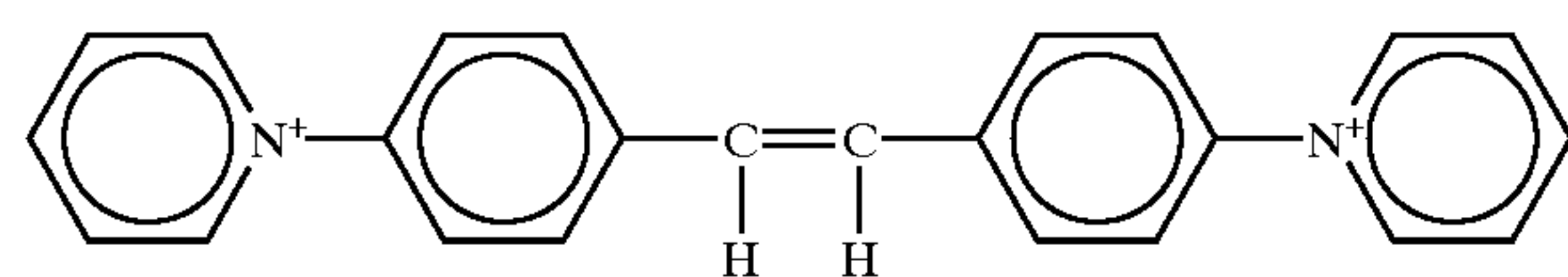
SN 18071
