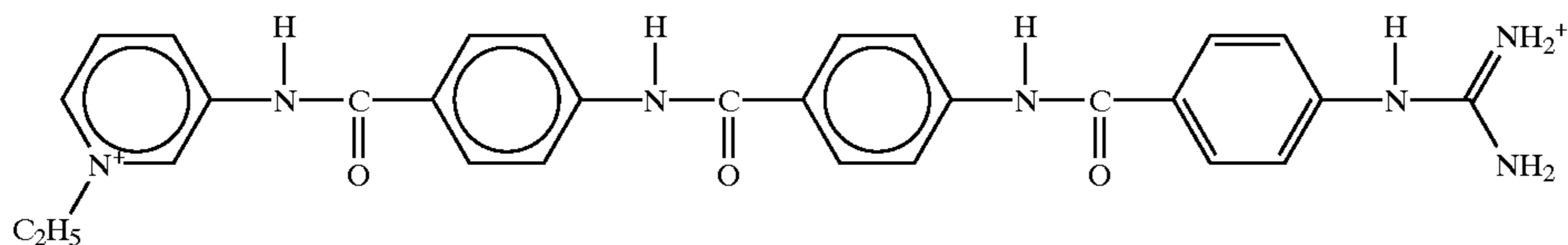
SN 6136
