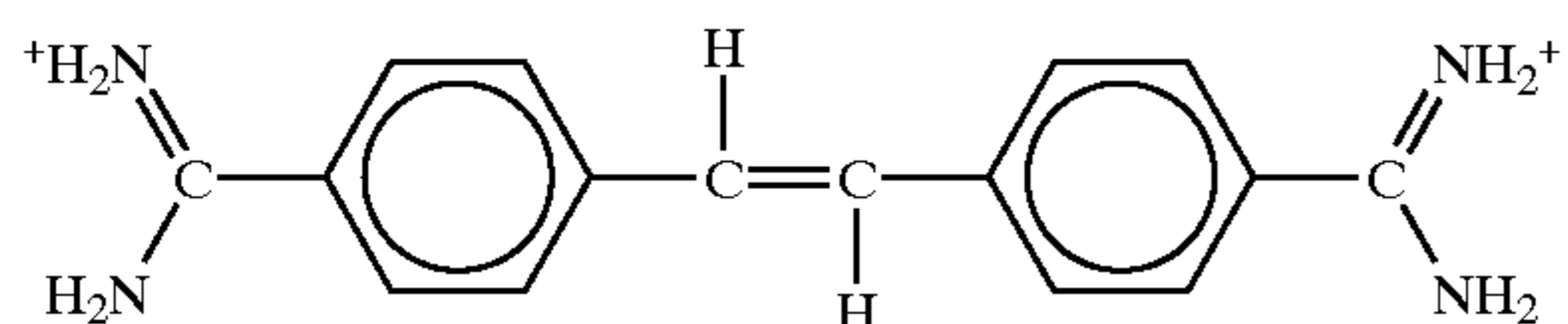
Stilbamidine
