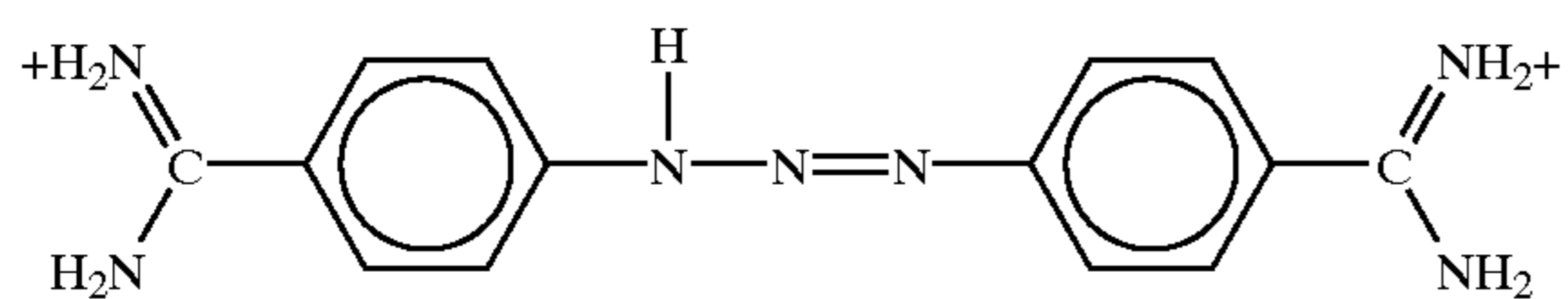
Berenil
