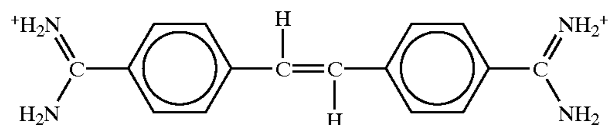
Stilbamidine
