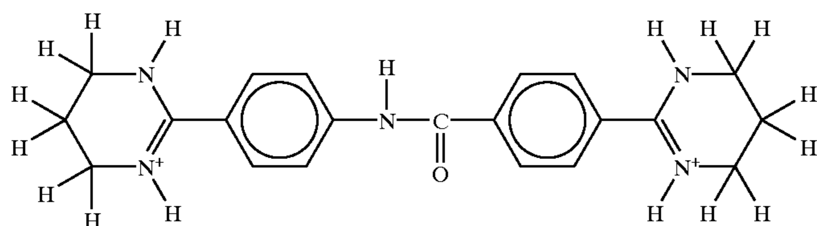
NSC 57153
