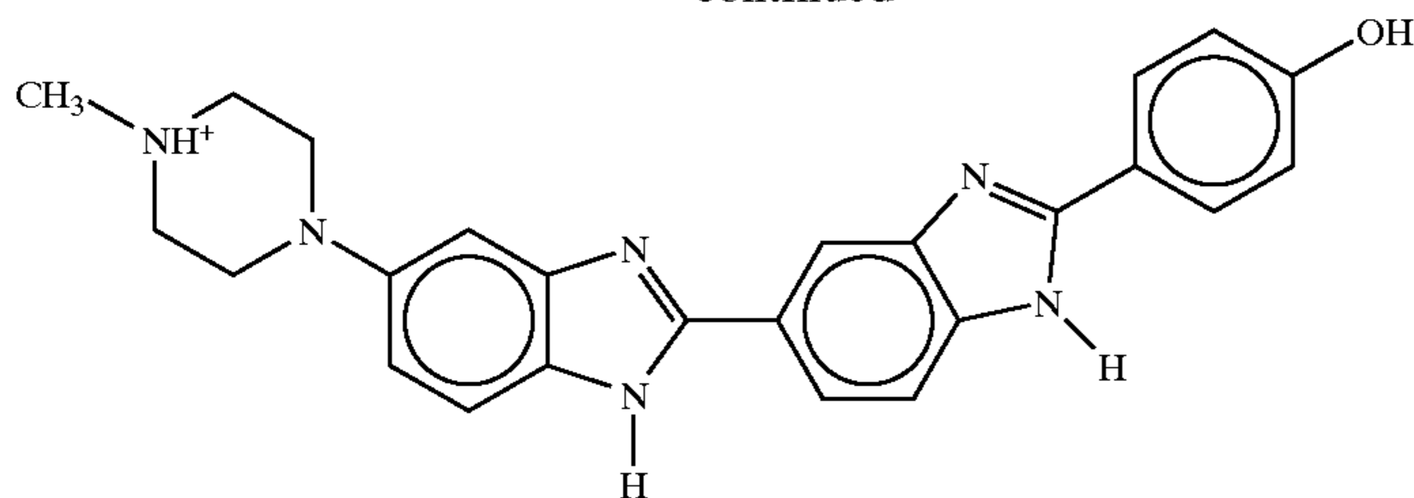
Hoechst 33258
