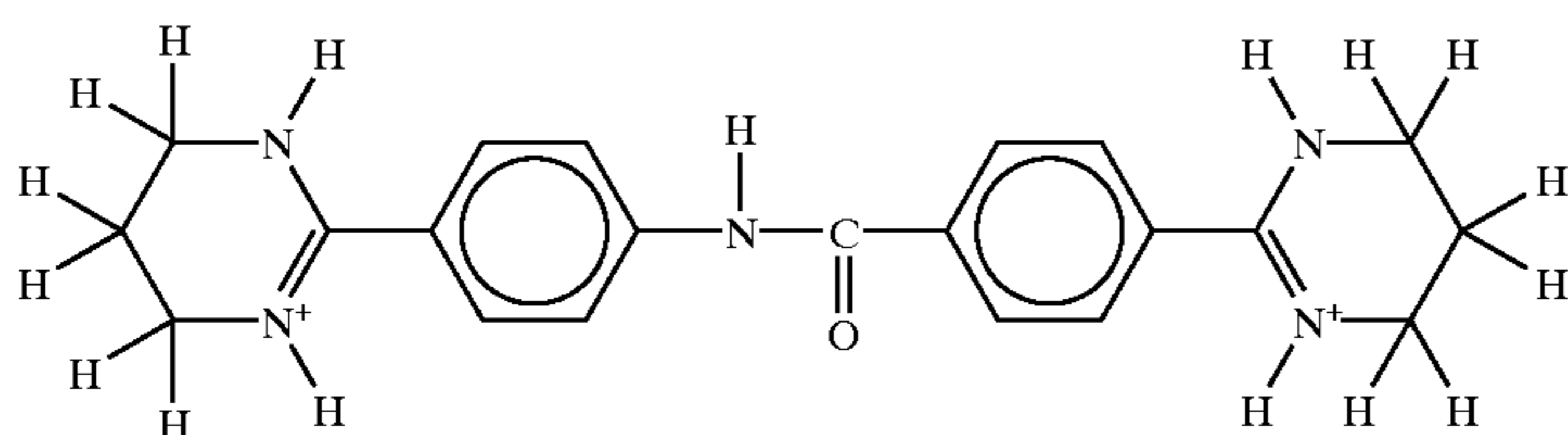
NSC 57153
