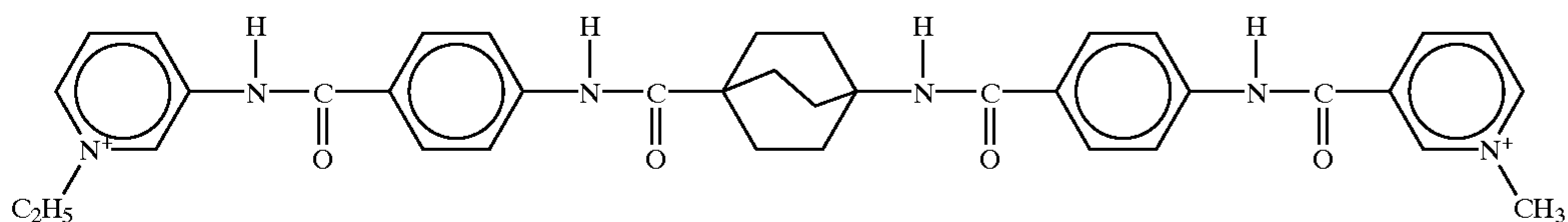
SN 16814
