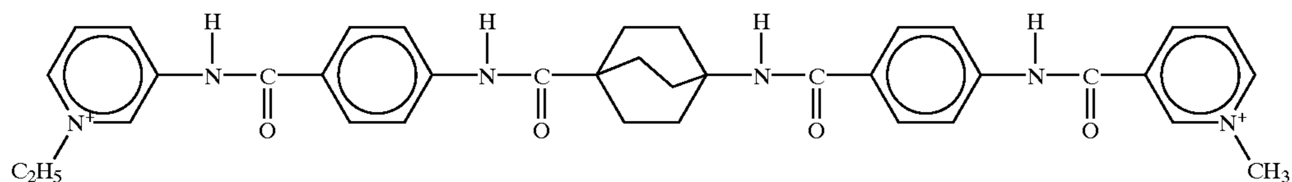
SN 16814
