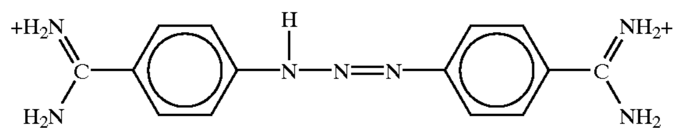
Berenil
