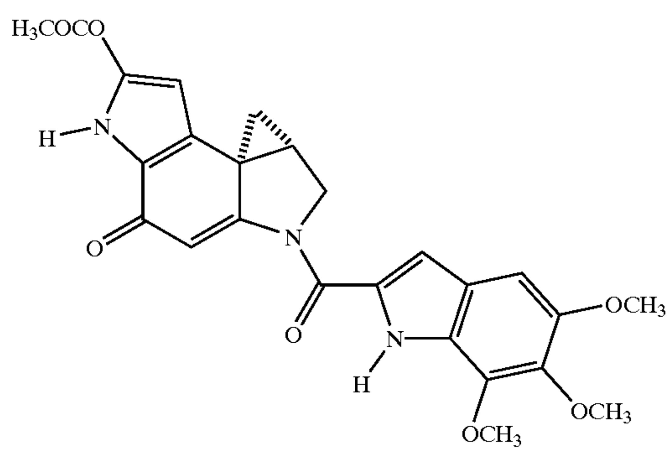
Duocarmycin SA
