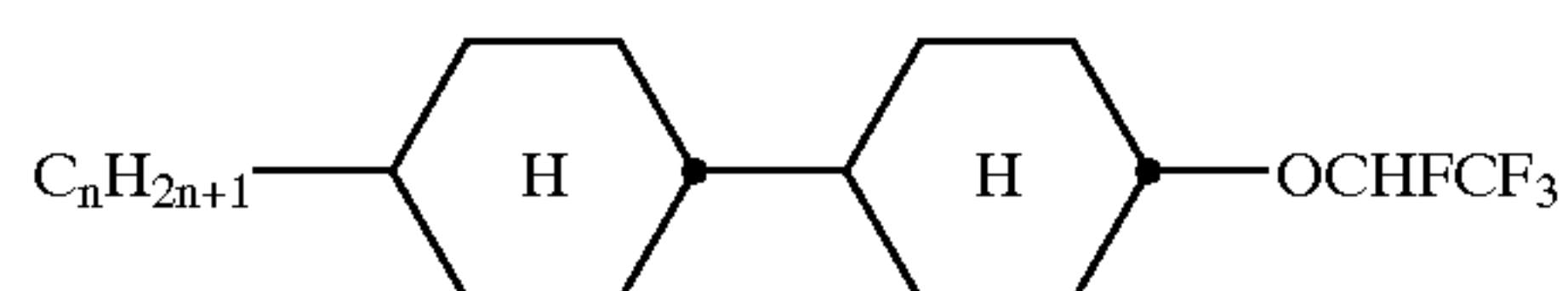
CC-n-OMT
