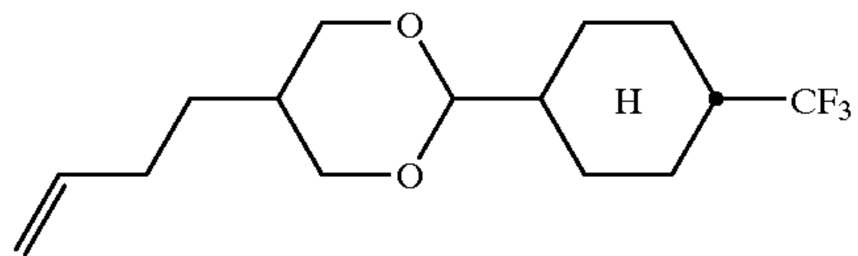
DC-V2-T
