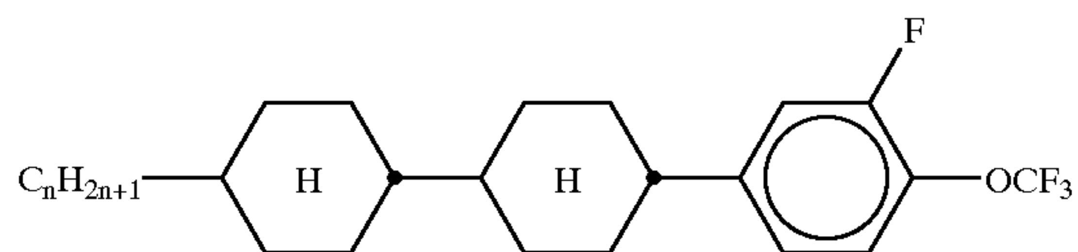
CCP-nOCF 3 .F
