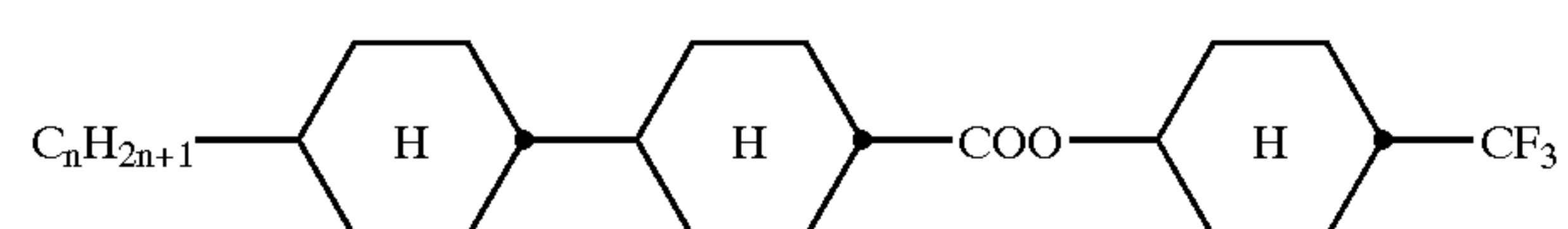
CCZC-n-T
