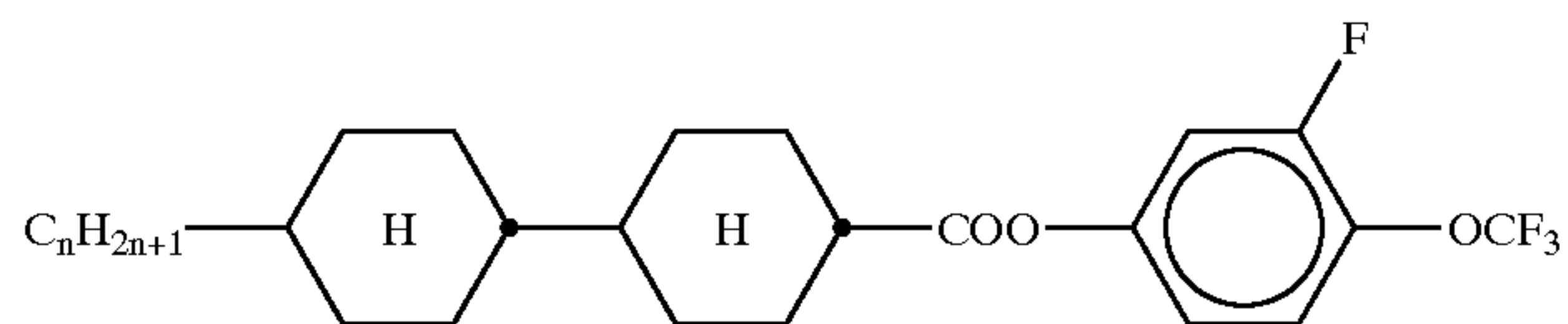
CCZG-n-OT
